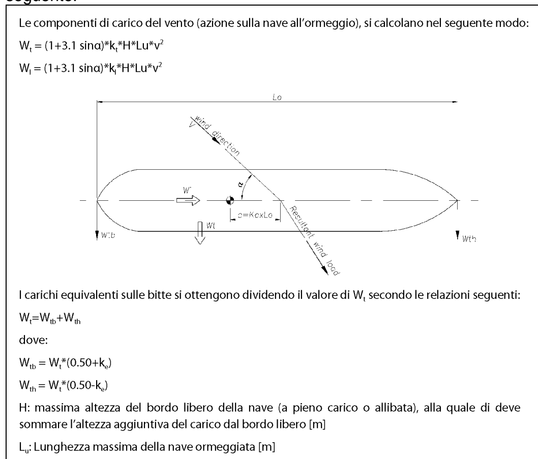
Figura 10: Calcolo del tiro sui ganci a scocco
