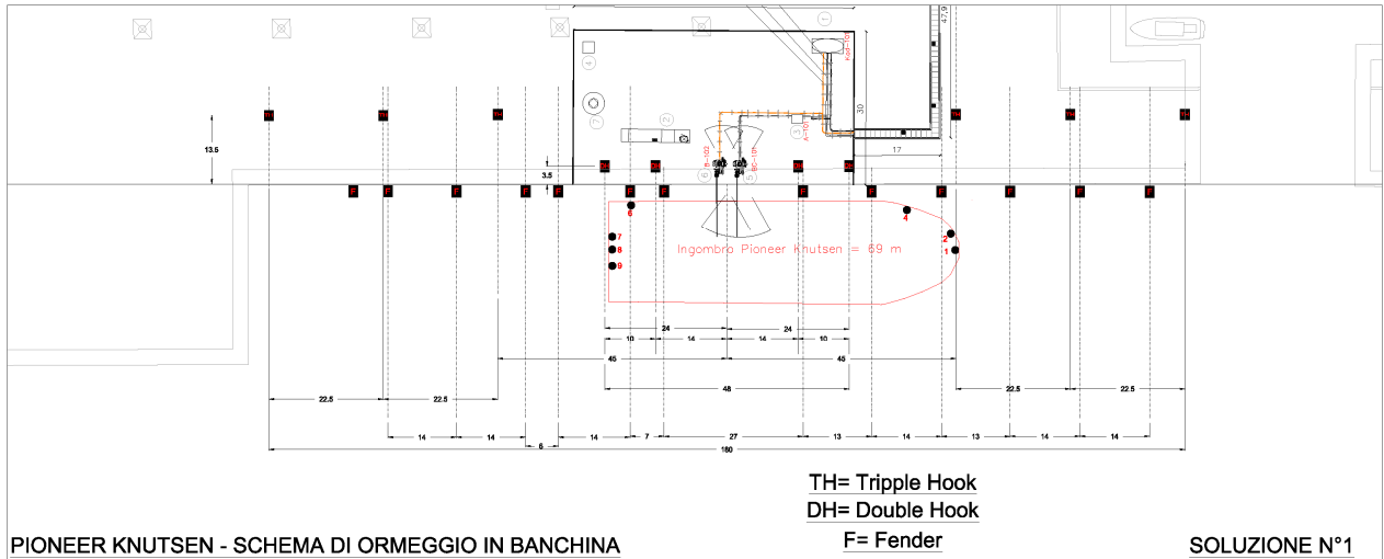
Figura 21: Schemi di ormeggio Pioner Knutsen – Soluzione n°1
