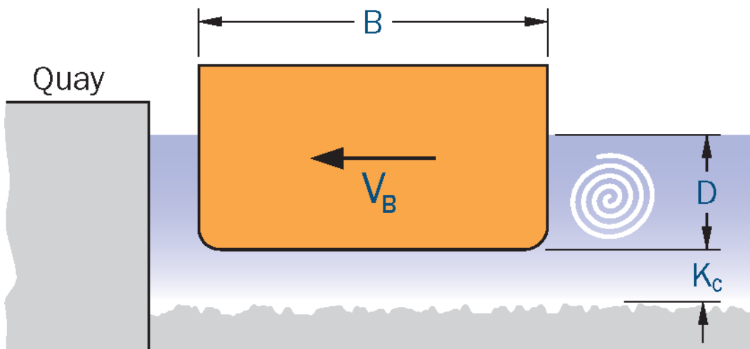
Figura 14: Calcolo del coefficiente di massa aggiunta
