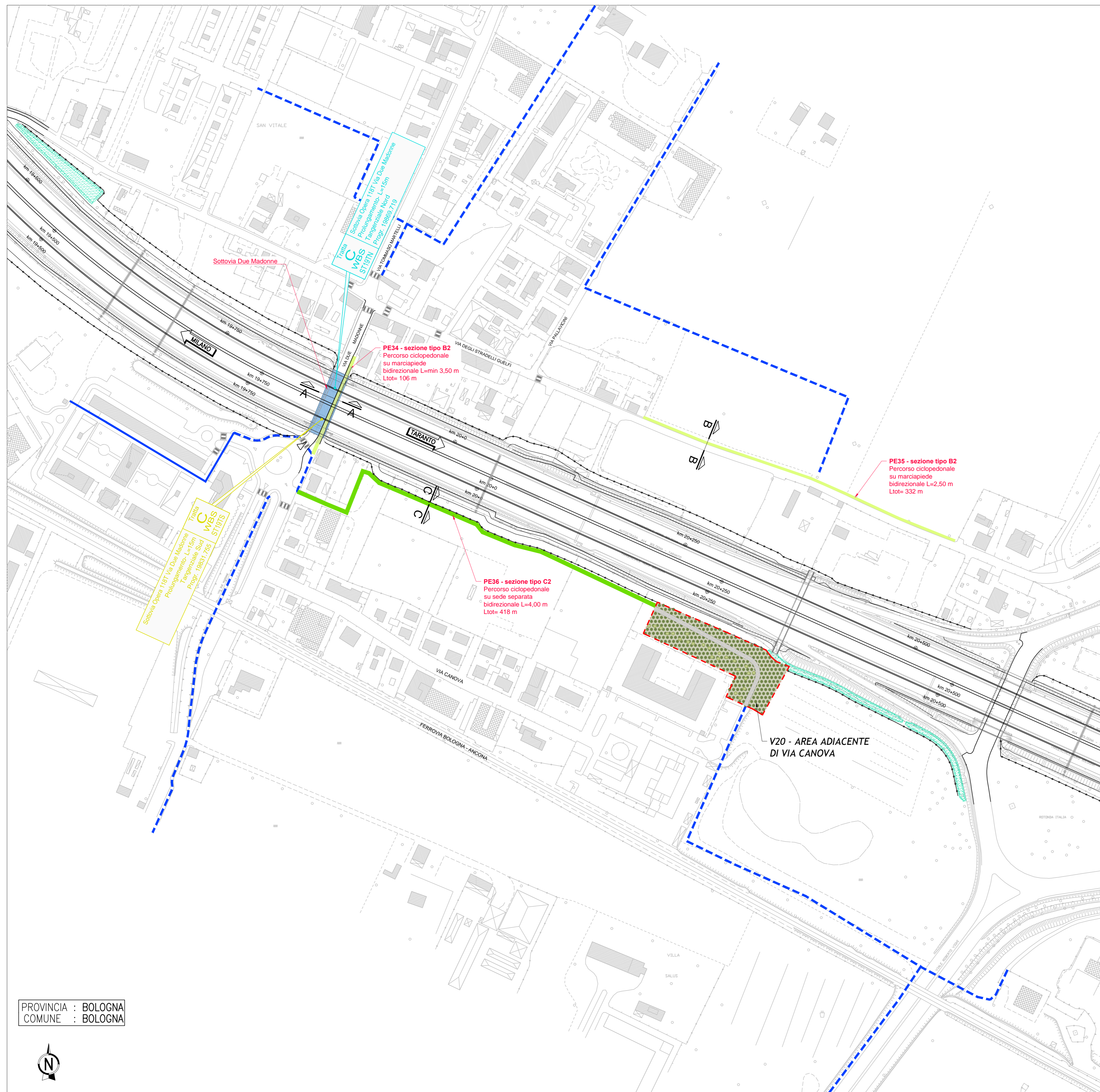
PLANIMETRIA DI PROGETTO - scala 1:2000
