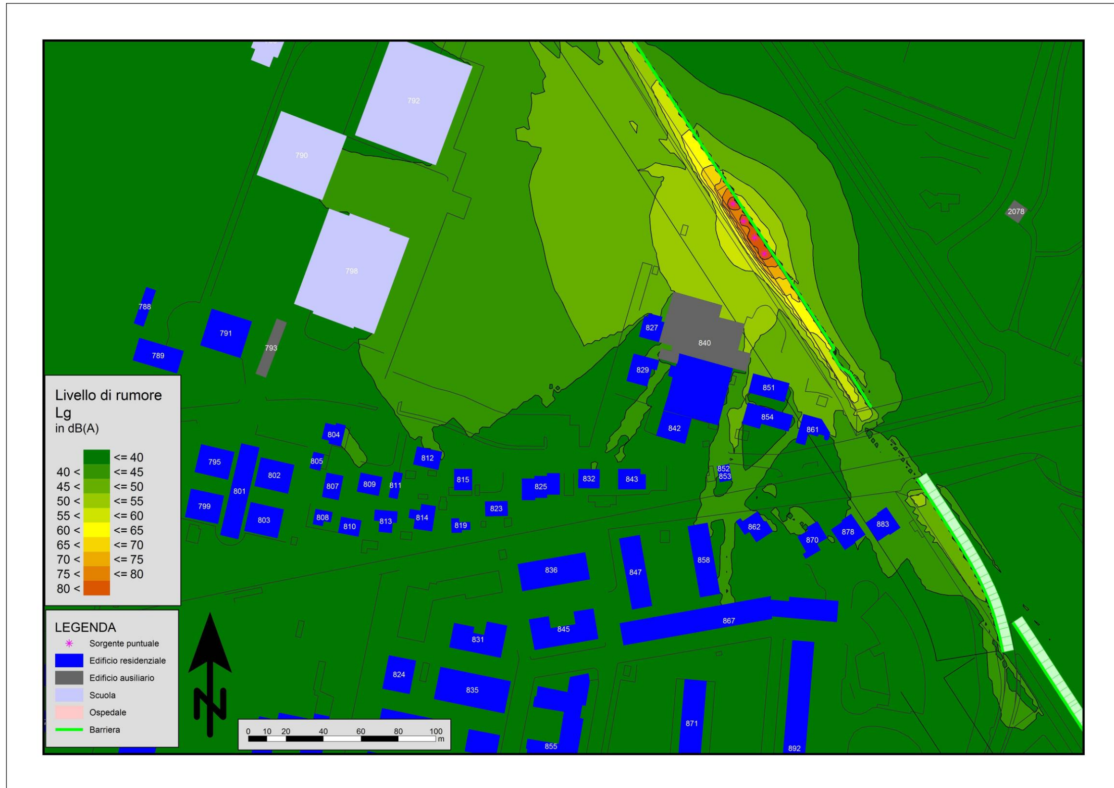
Figura Errore. Nel documento non esiste testo dello stile specificato.-23: Mappa Cantiere Sezione TS 524 – formazione rilevati (lavorazioni a metà altezza) non mitigato
