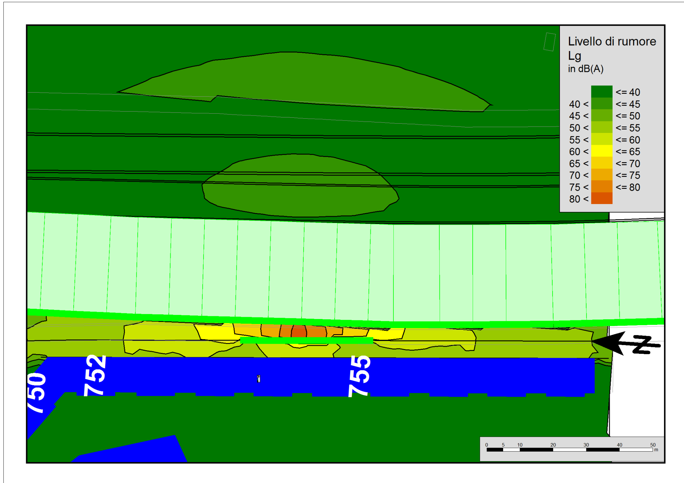
Figura Erronea. Nel documento non esiste testo dello stile specificato.-14: Mappa Cantiere – Sezione Galleria Antifonica San Donnino – realizzazione pali di sottofondazione mitigato
