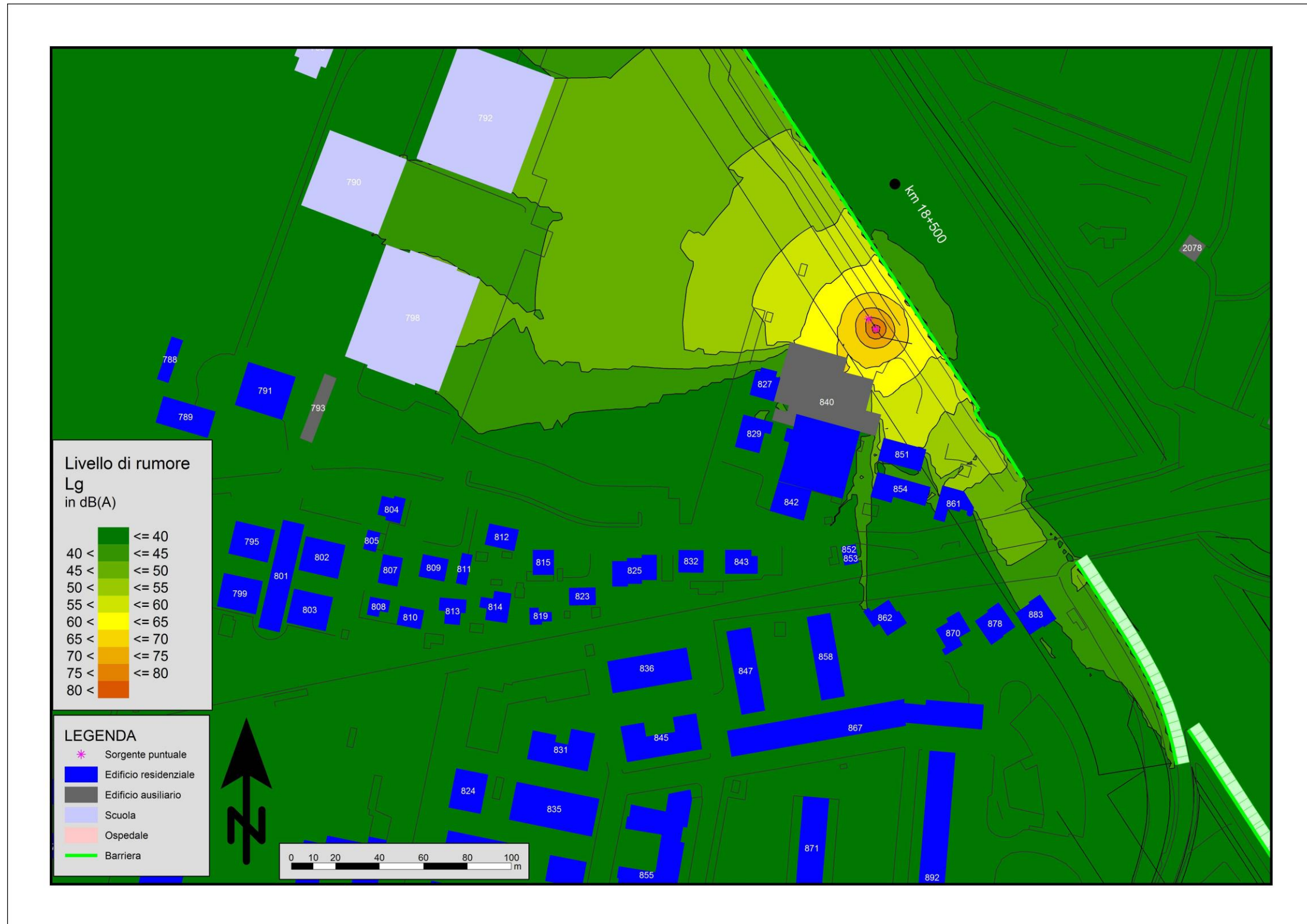
Figura Errore. Nel documento non esiste testo dello stile specificato.-19: Mappa Cantiere Sezione TS 524 – realizzazione pali di sottofondazione non mitigato
