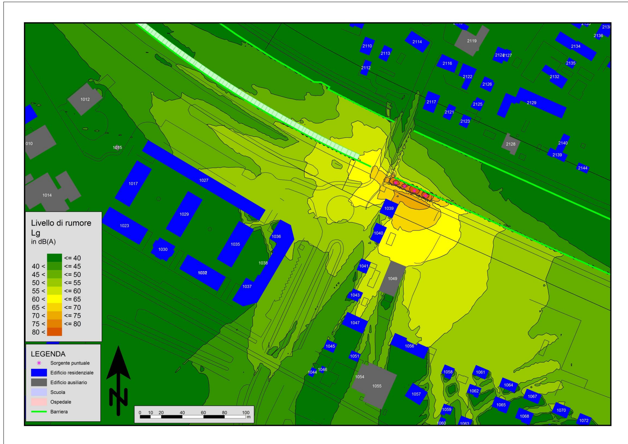
Figura Errone. Nel documento non esiste testo dello stile specificato.-29: Mappa Cantiere Sezione TS 588 – formazione rilevati (lavorazioni a metà altezza) non mitigato
