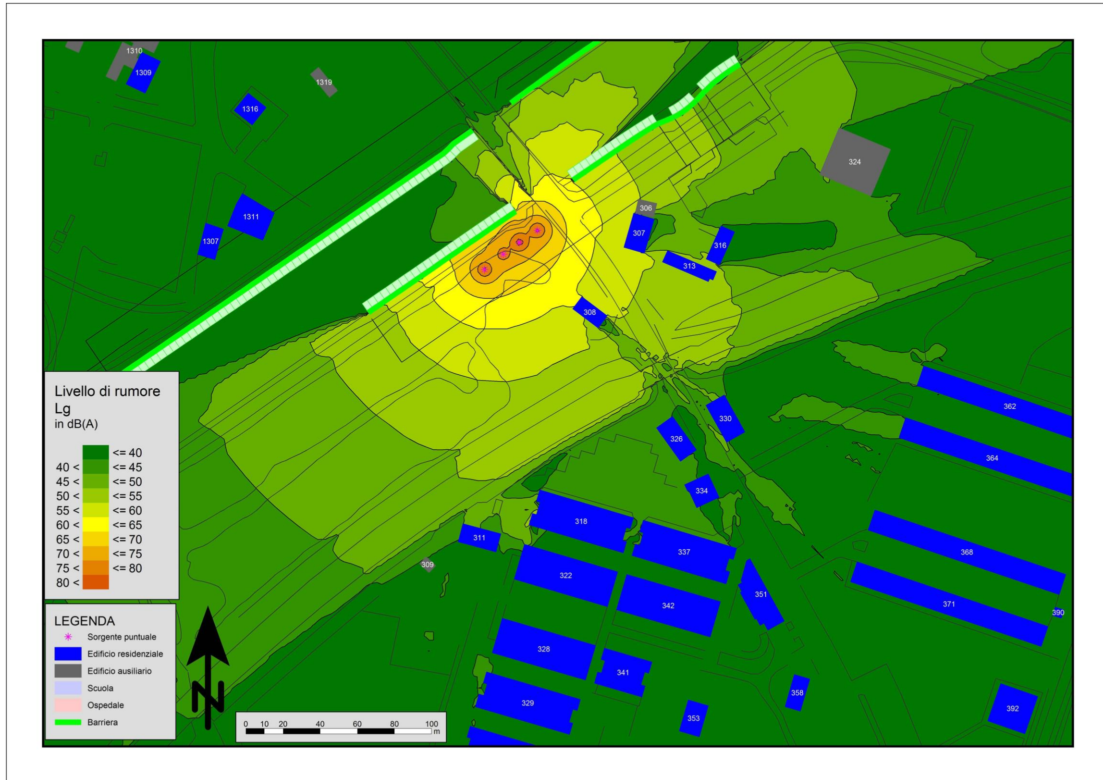
Figura Errore. Nel documento non esiste testo dello stile specificato.-3: Mappa Cantiere Sezione TS 136 – formazione rilevati (lavorazioni a quota piano di campagna) non mitigato
