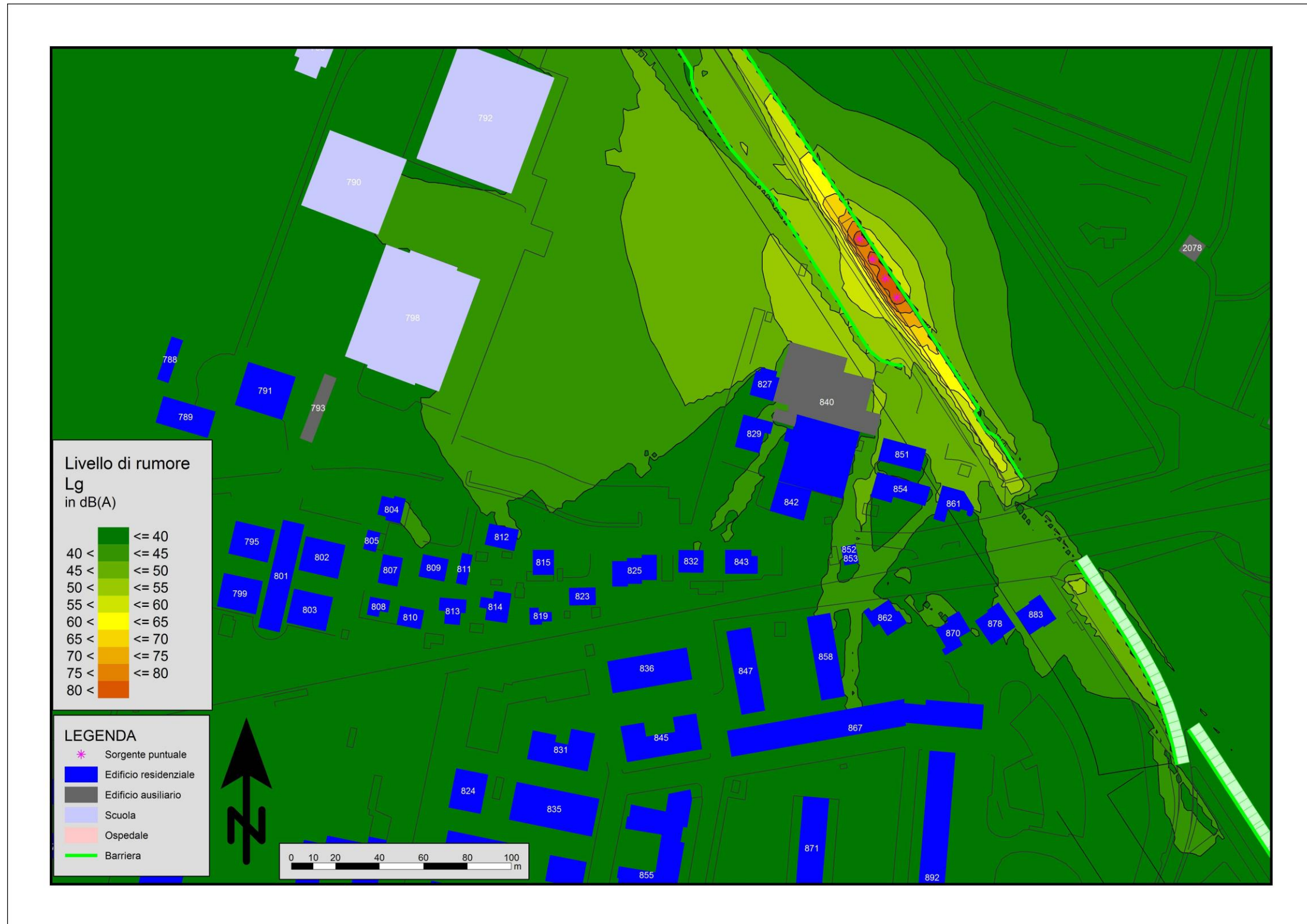
Figura Errore. Nel documento non esiste testo dello stile specificato.-24: Mappa Cantiere Sezione TS 524 – formazione rilevati (lavorazioni a metà altezza) mitigato
