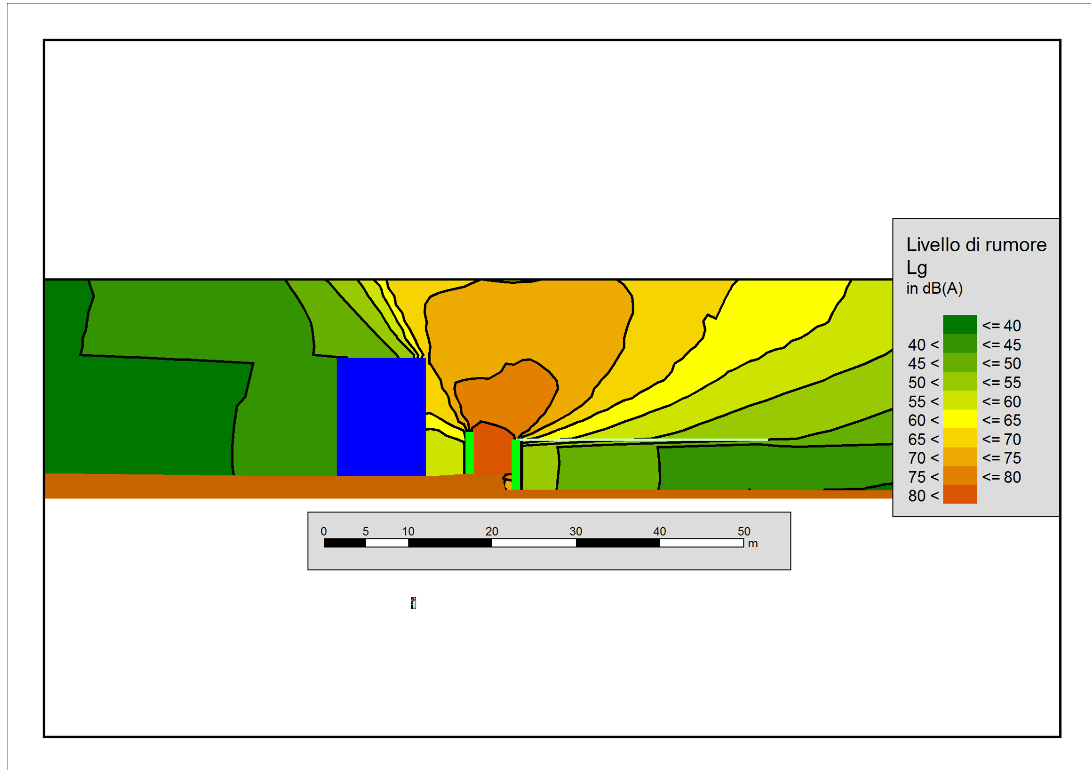
Figura Errore. Nel documento non esiste testo dello stile specificato.-18: Mappa Cantiere – Sezione Galleria Antifonica San Donnino – esecuzione getti mitigato sezione verticale
