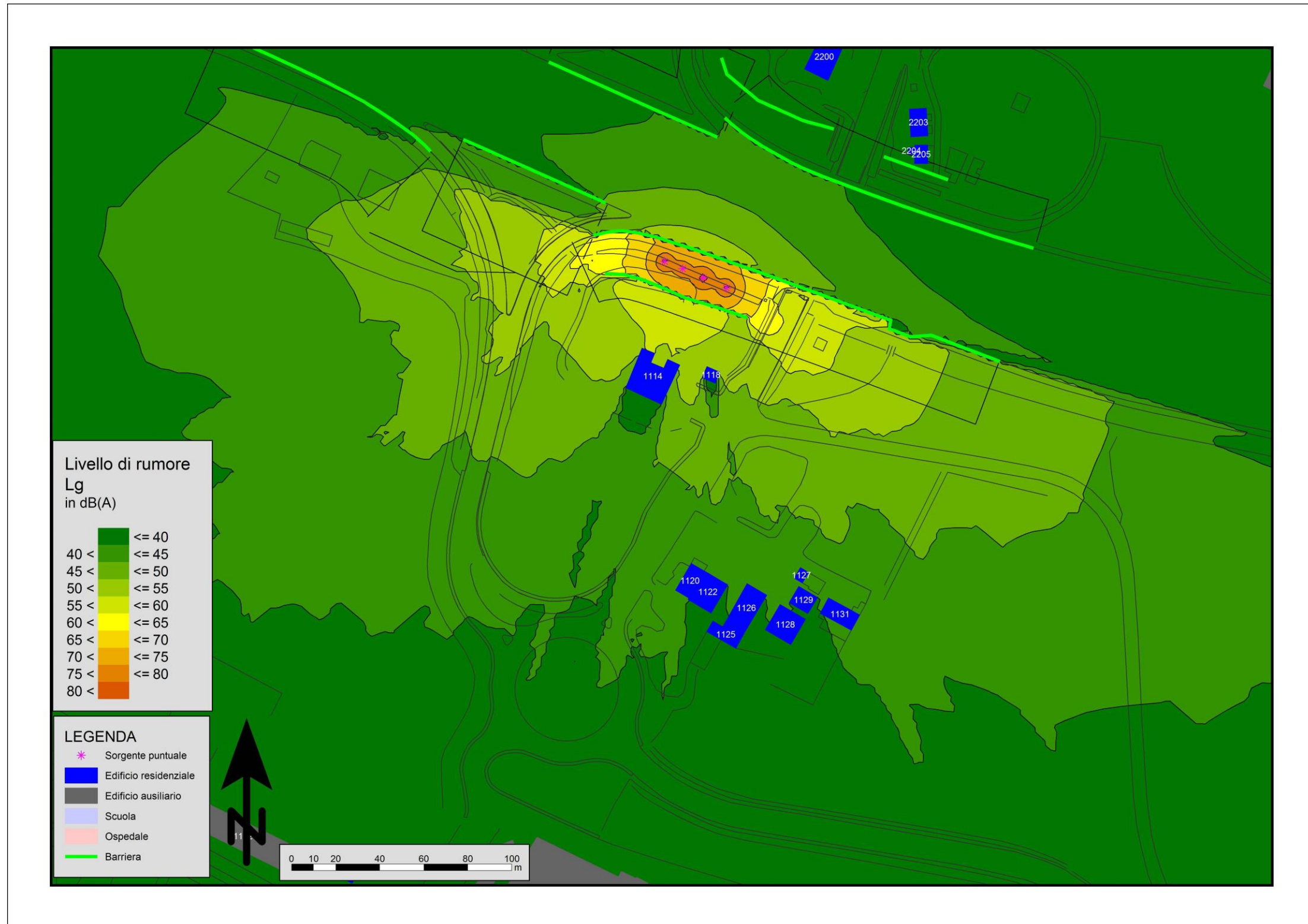
Figura Errone. Nel documento non esiste testo dello stile specificato.-34: Mappa Cantiere Sezione TS 683 – formazione rilevati (lavorazioni a metà altezza) mitigato
