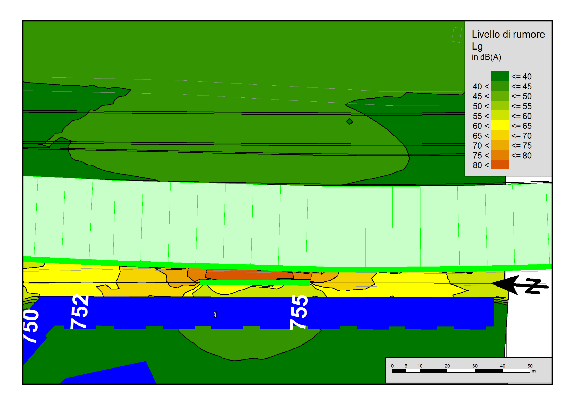
Figura Errore. Nel documento non esiste testo dello stile specificato.-17: Mappa Cantiere – Sezione Galleria Antifonica San Donnino – esecuzione getti mitigato
