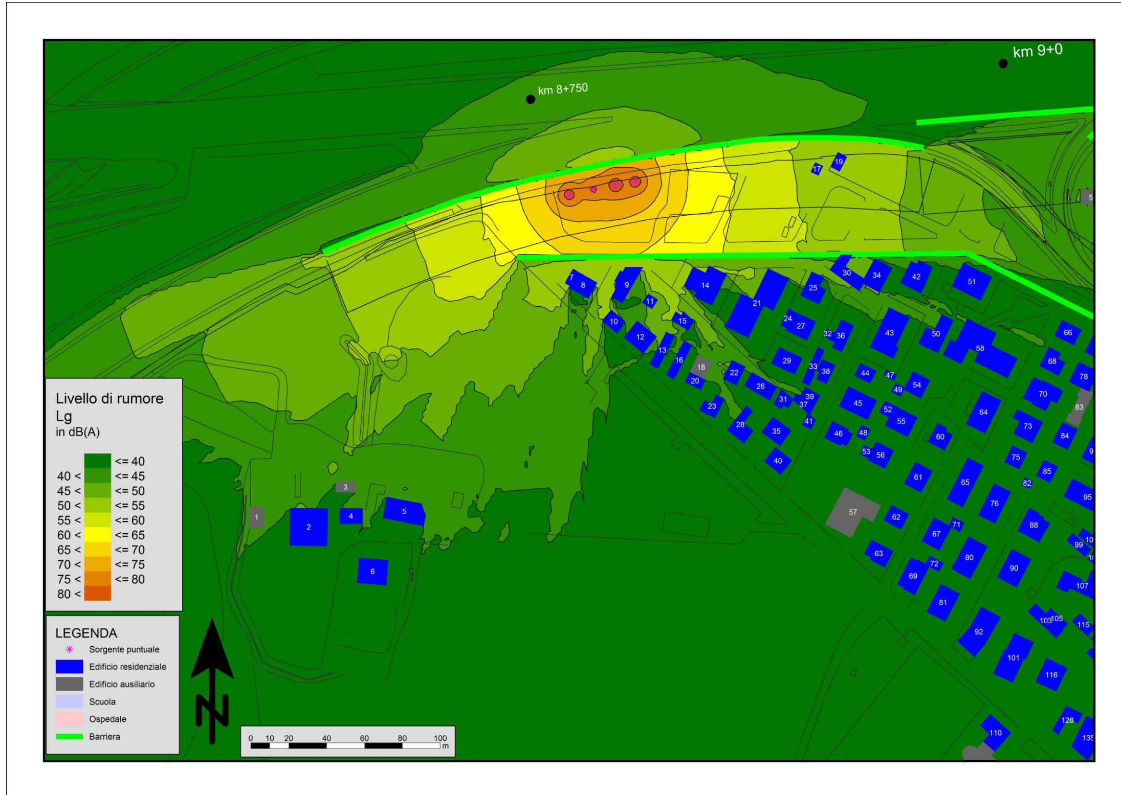
Figura Errore. Nel documento non esiste testo dello stile specificato.-2: Mappa Cantiere – formazione rilevati (lavorazioni a quota piano di campagna) mitigato – Sezione TS 35
