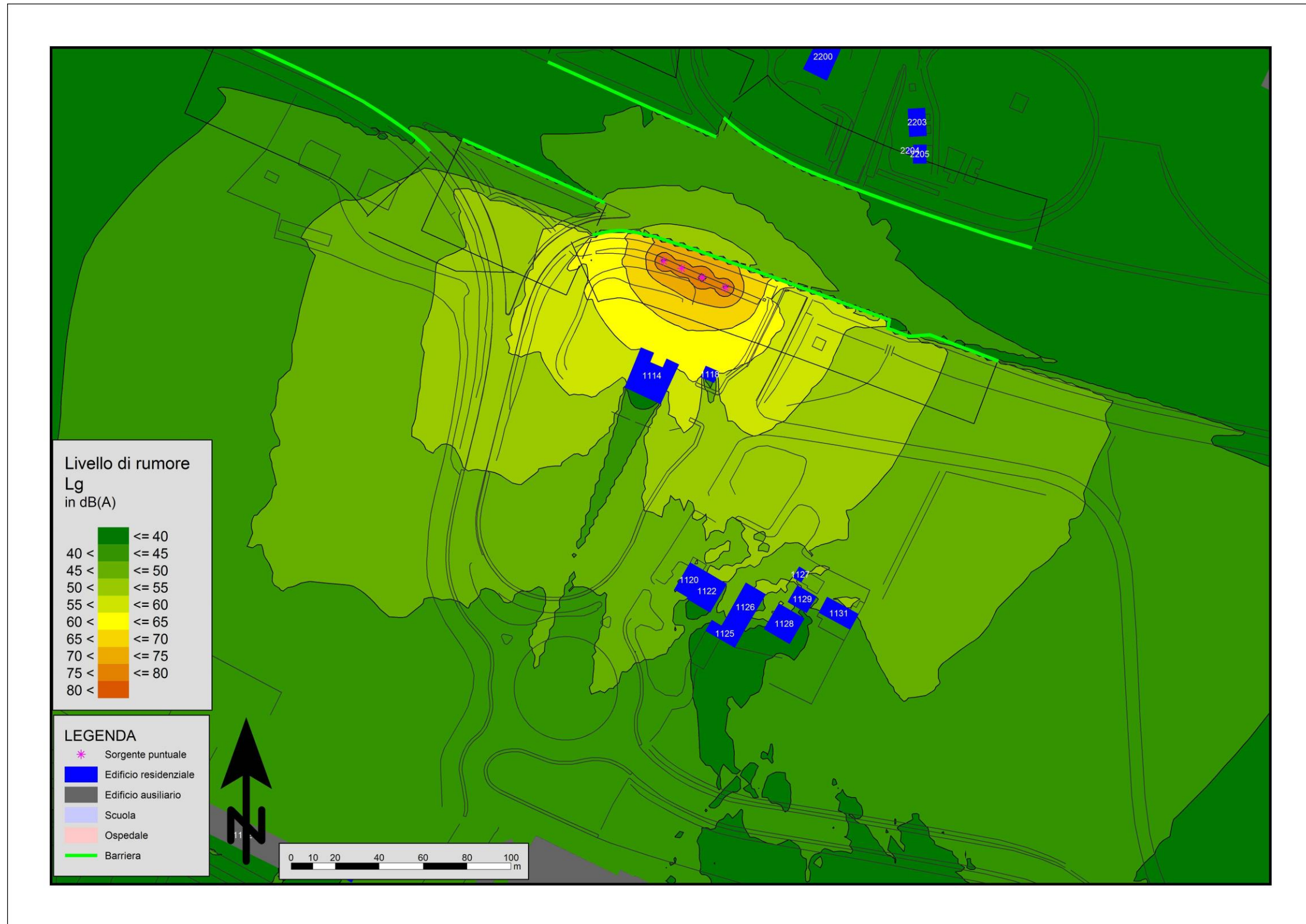
Figura Errone. Nel documento non esiste testo dello stile specificato.-33: Mappa Cantiere Sezione TS 683 – formazione rilevati (lavorazioni a metà altezza) non mitigato
