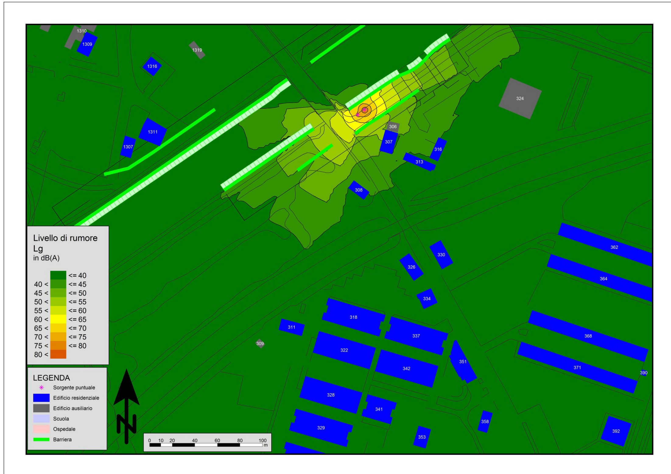
Figura Errore. Nel documento non esiste testo dello stile specificato.-8: Mappa Cantiere Sezione TS 139 – realizzazione pali di sottofondazione mitigato
