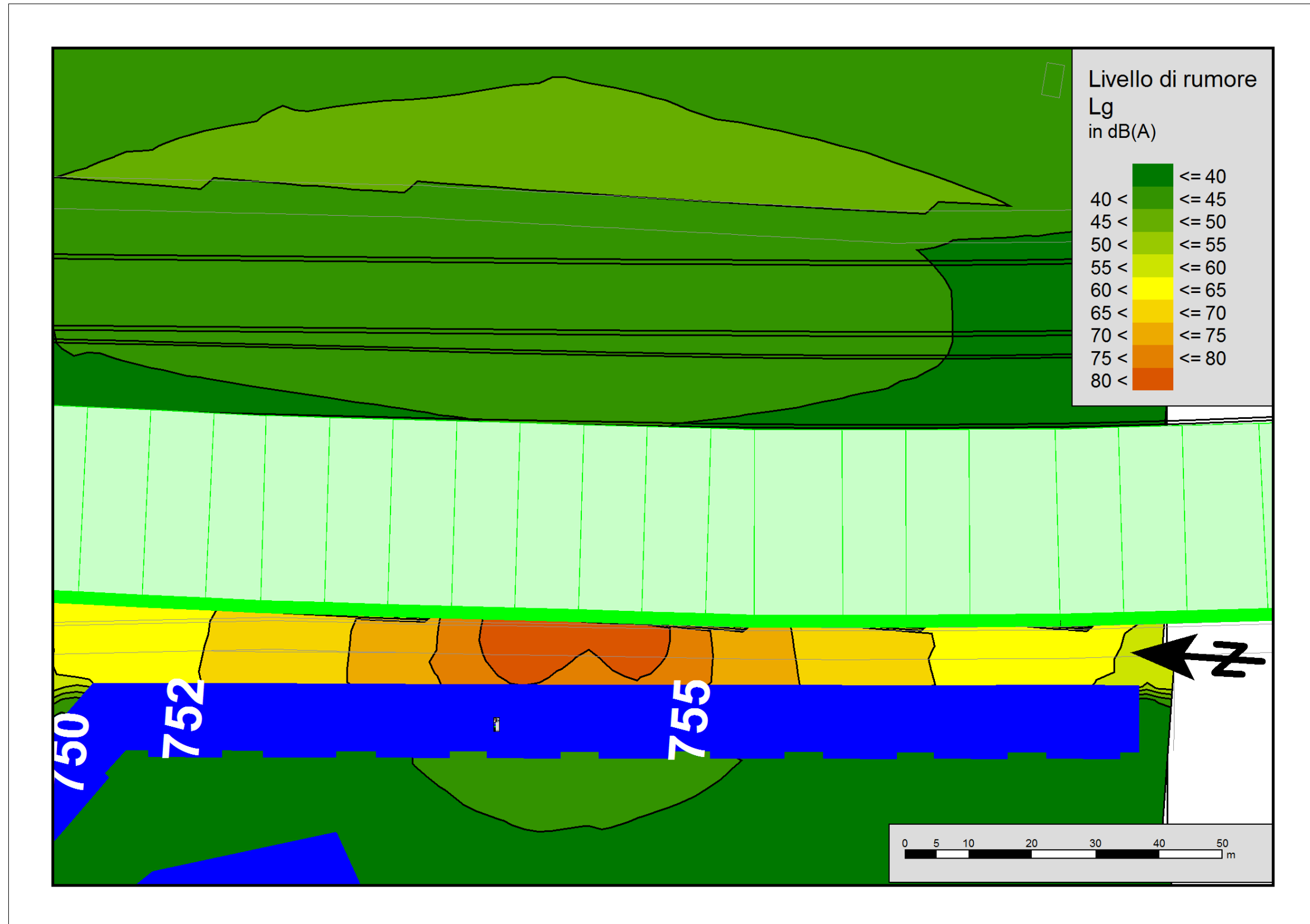
Figura Errore. Nel documento non esiste testo dello stile specificato.-16: Mappa Cantiere – Sezione Galleria Antifonica San Donnino – esecuzione getti non mitigato
