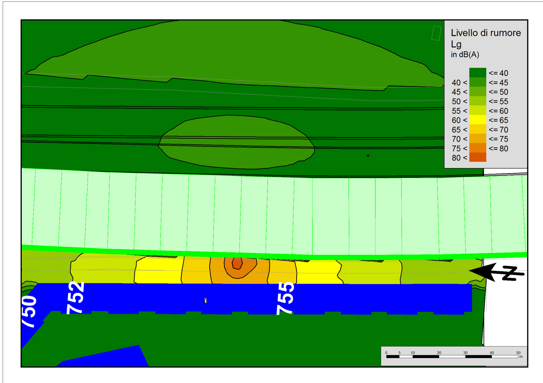
Figura Erronea. Nel documento non esiste testo dello stile specificato.-13: Mappa Cantiere – Sezione Galleria Antifonica San Donnino – realizzazione pali di sottofondazione non mitigato
