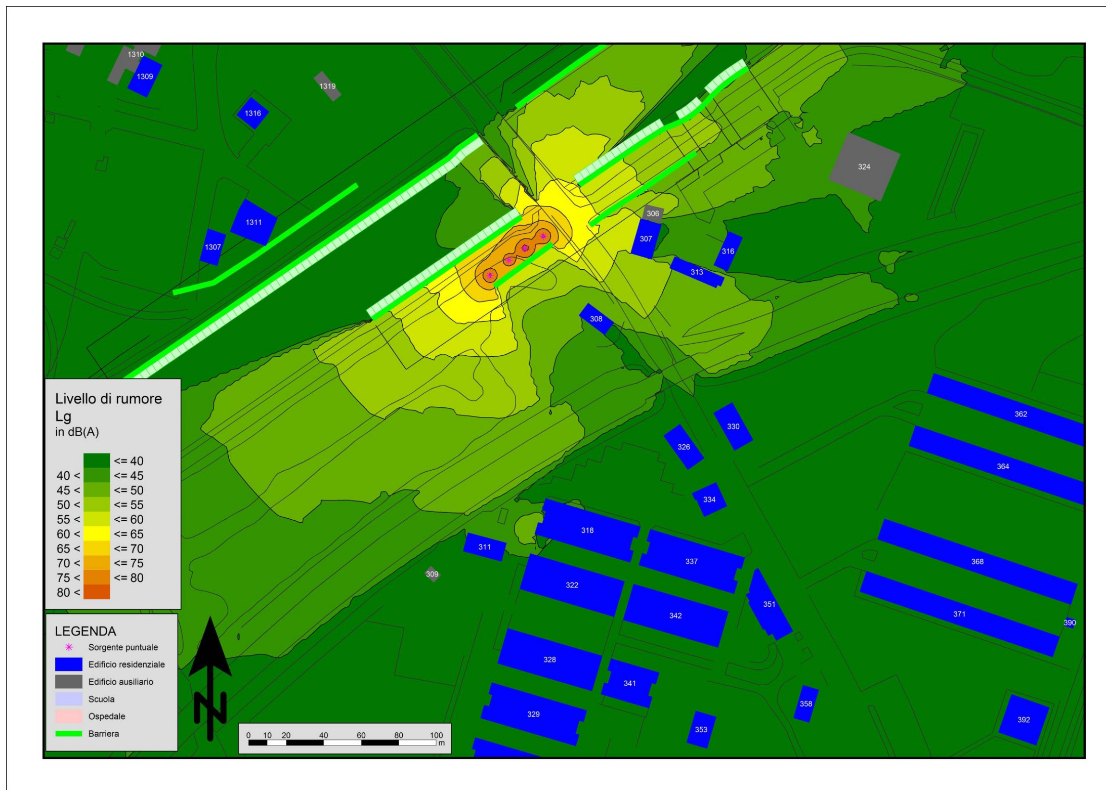
Figura Errore. Nel documento non esiste testo dello stile specificato.-4: Mappa Cantiere Sezione TS 136 – formazione rilevati (lavorazioni a quota piano di campagna) mitigato
