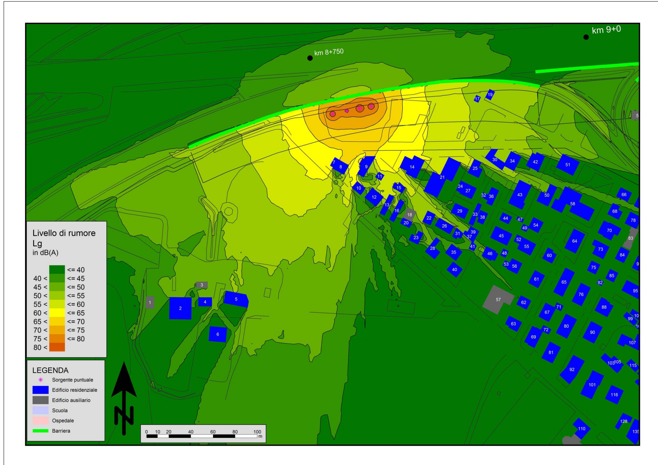
Figura Errore. Nel documento non esiste testo dello stile specificato.-1: Mappa Cantiere – formazione rilevati (lavorazioni a quota piano di campagna) non mitigato – Sezione TS 35
