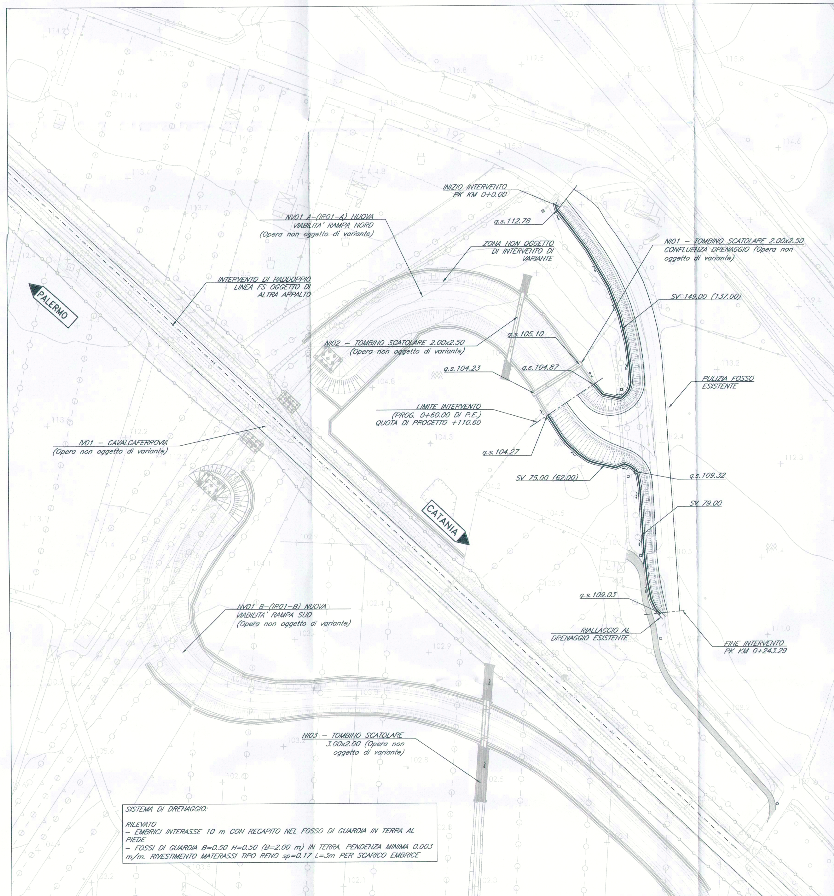
PLANIMETRIA DI SMALTIMENTO IDRAULICO Scala 1:1000
