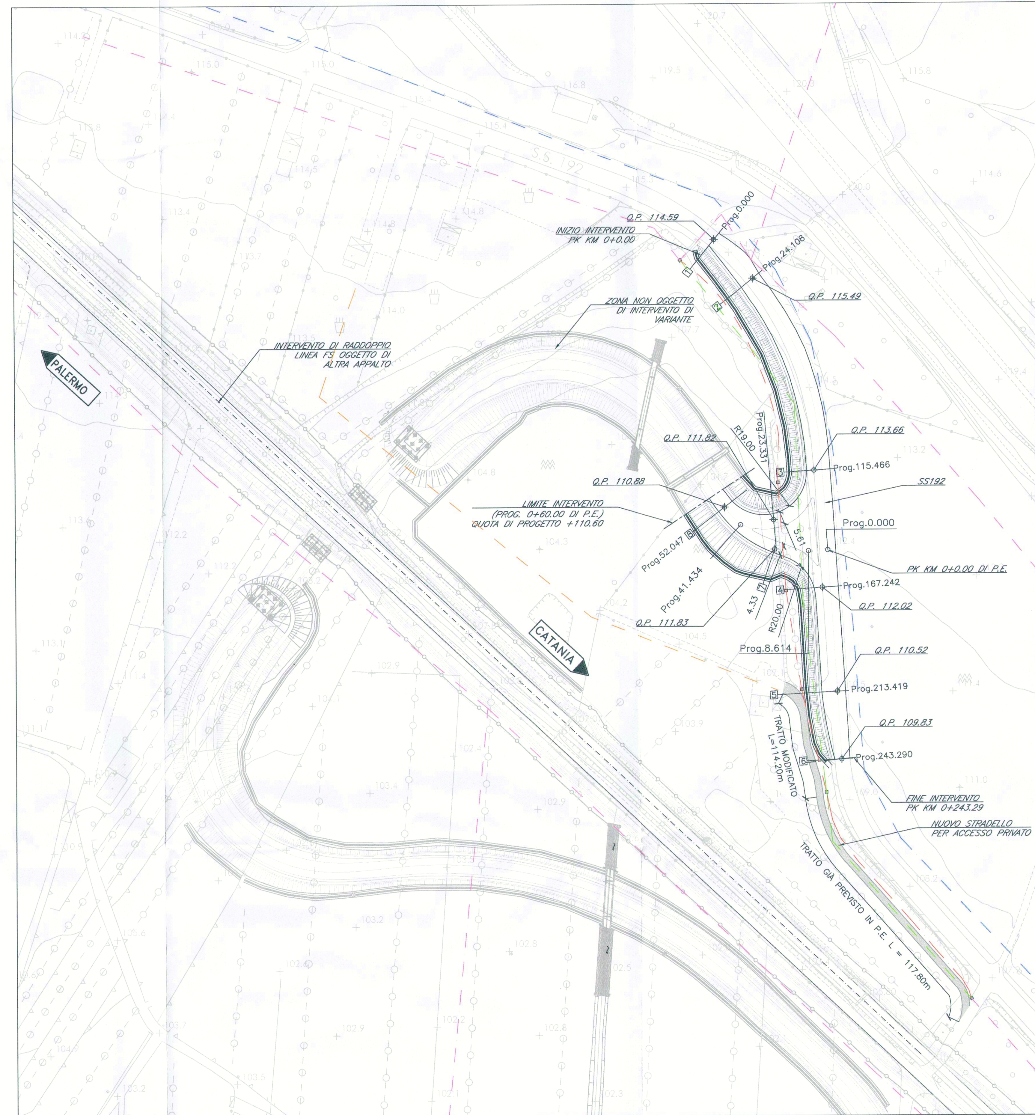
PLANIMETRIA DI PROGETTO Scala 1:1000
