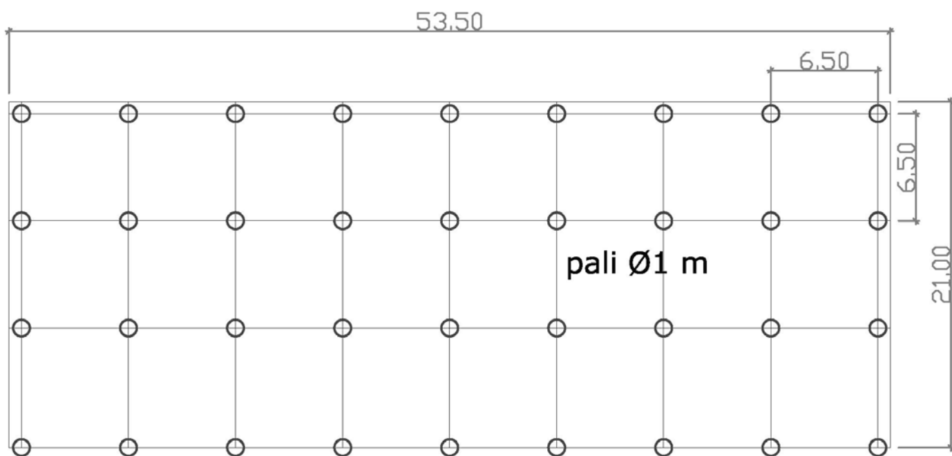
Figura 8 – Molo d'attracco della Società Diano. Pianta
