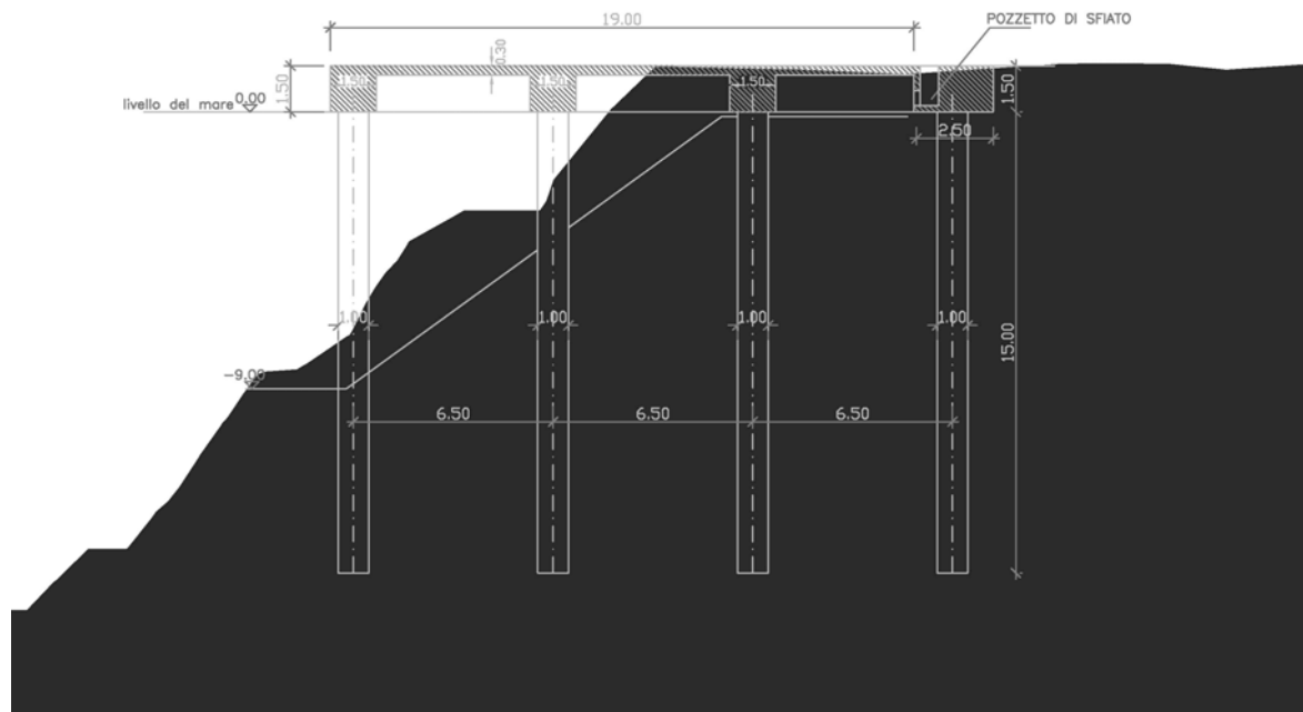
Figura 10 – Sezione tipo di entrambi gli attracchi
