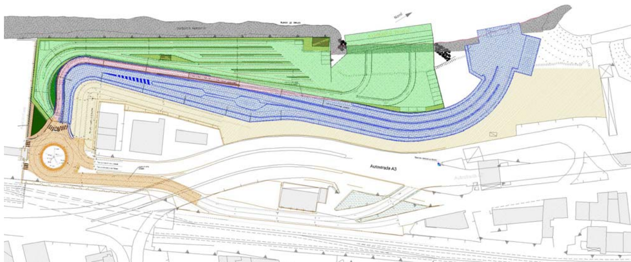
Figura 5 - Planimetria generale dell'opera con destinazione delle aree
