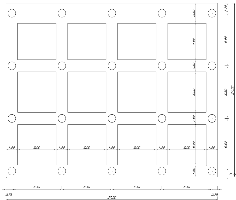
Figura 8 – Molo d'attracco della Società Diano. Pianta
