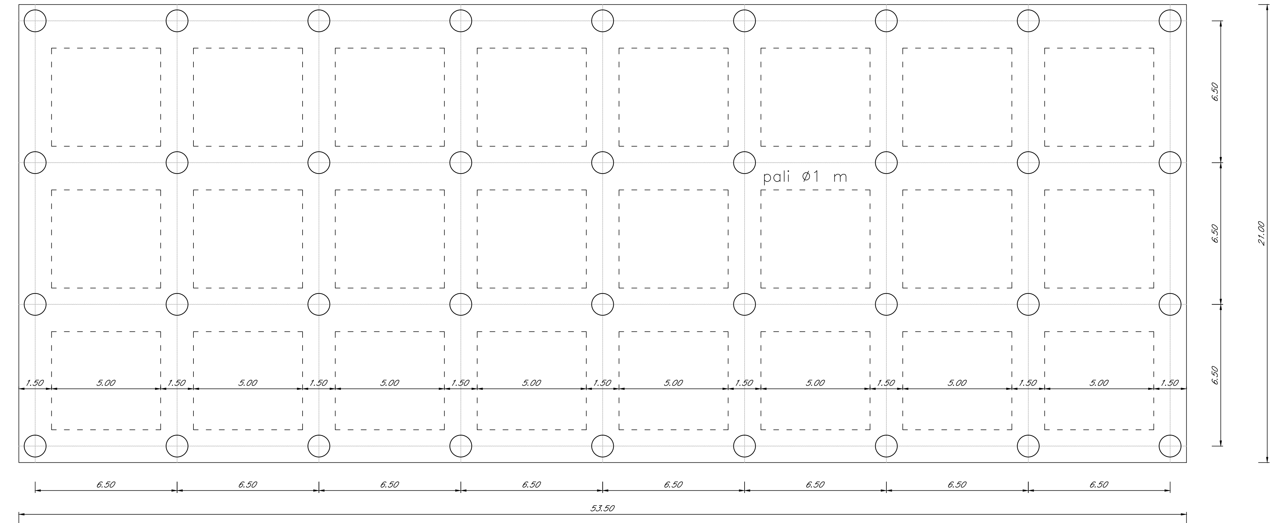
PIANTA STRUTTURALE BANCHINA DI ATTRACCO
