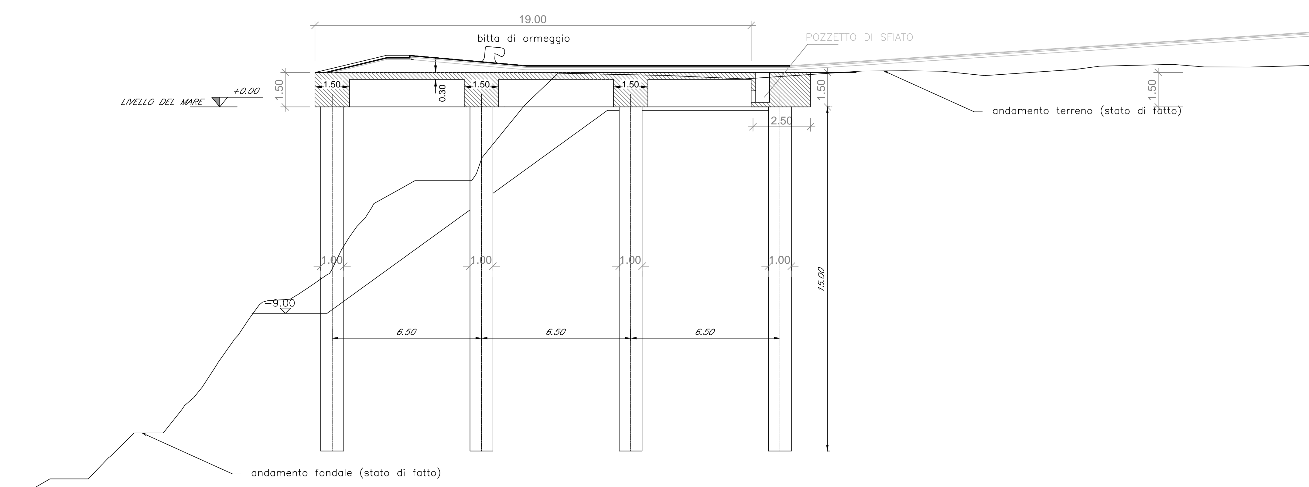
SEZIONE TIPO BANCHINA SOVRAPPONATA ALLO STATO DI FATTO
