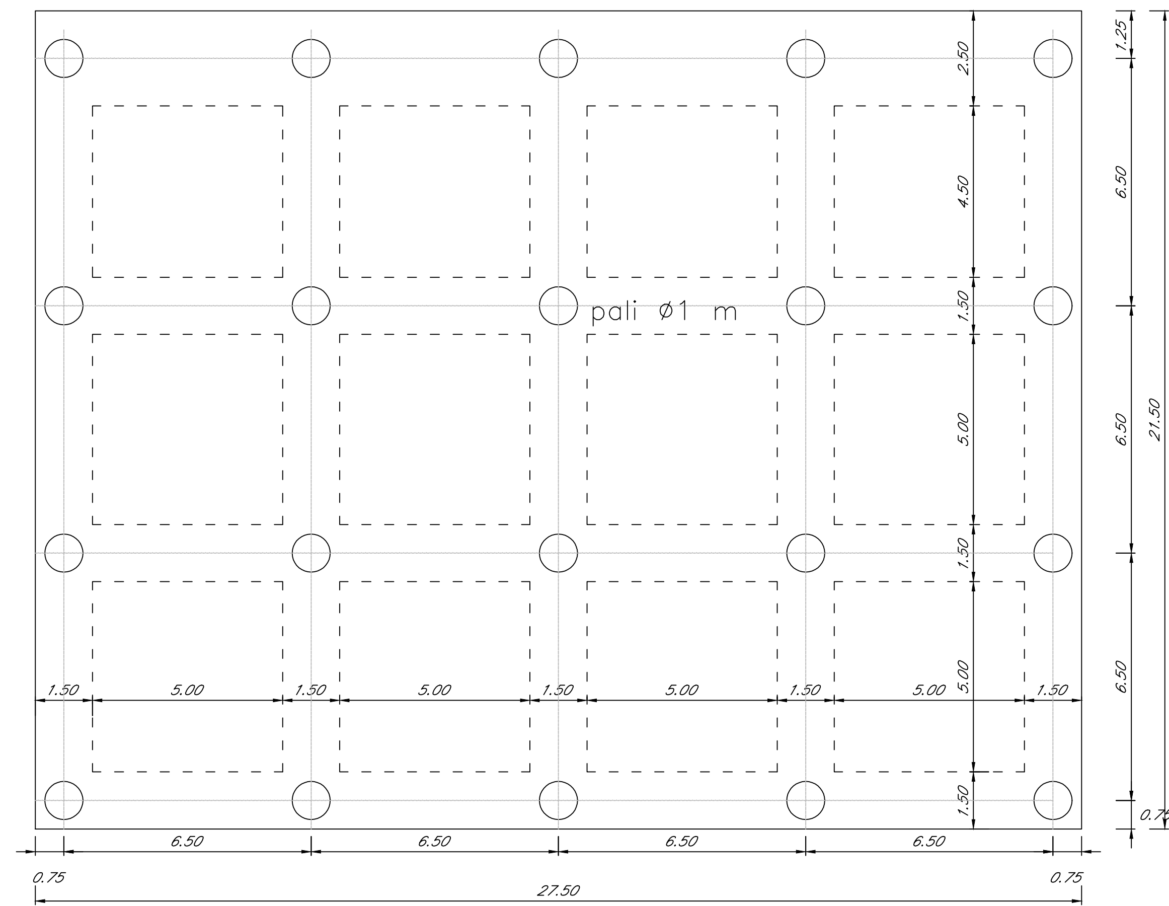
PIANTA STRUTTURALE BANCHINA DI ATTRACCO
