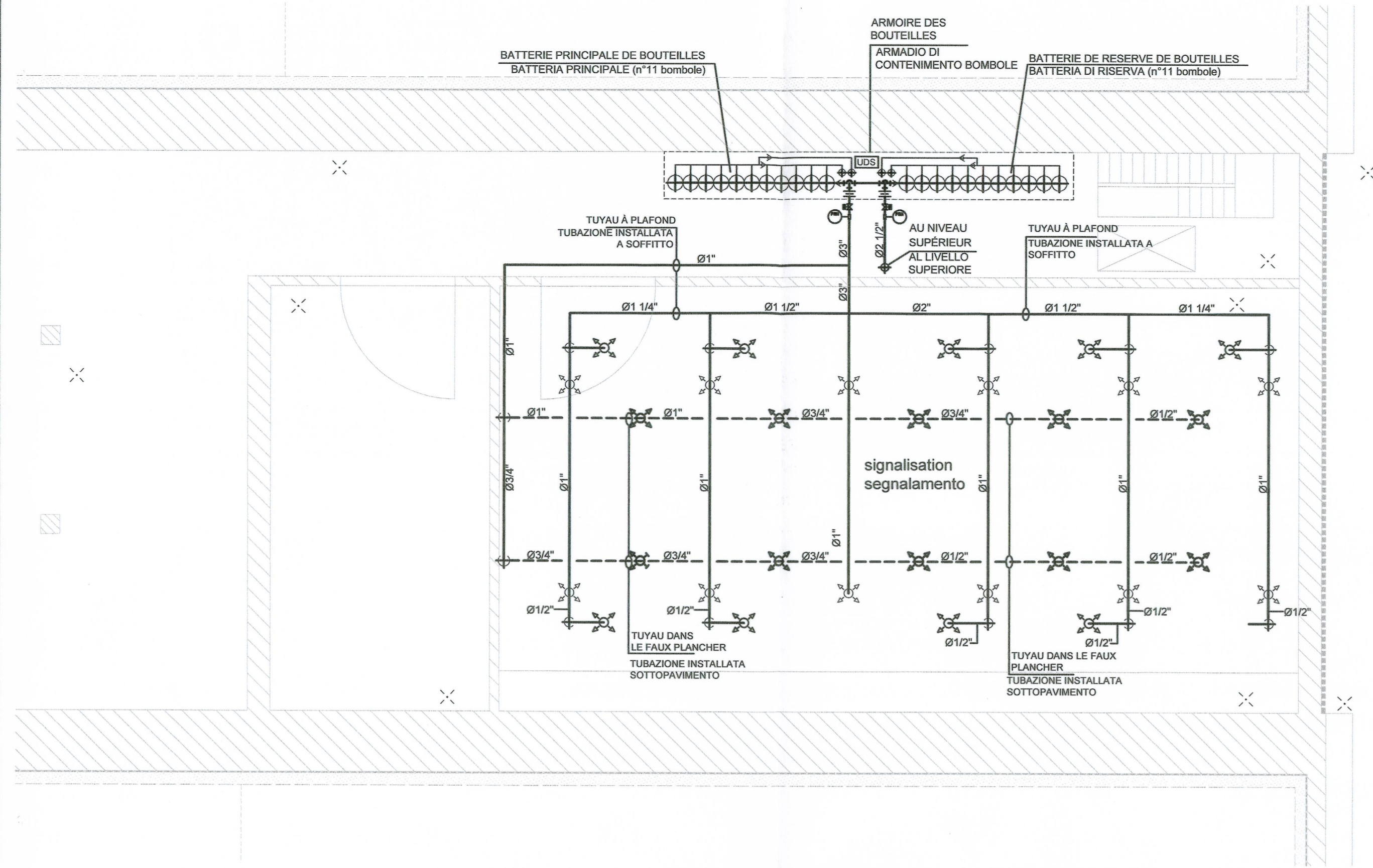
PLAN AU NIVEAU E1 - HAUTEUR 0,65 STRALCIO PIANTA PIANO E1 - QUOTA 0,65
