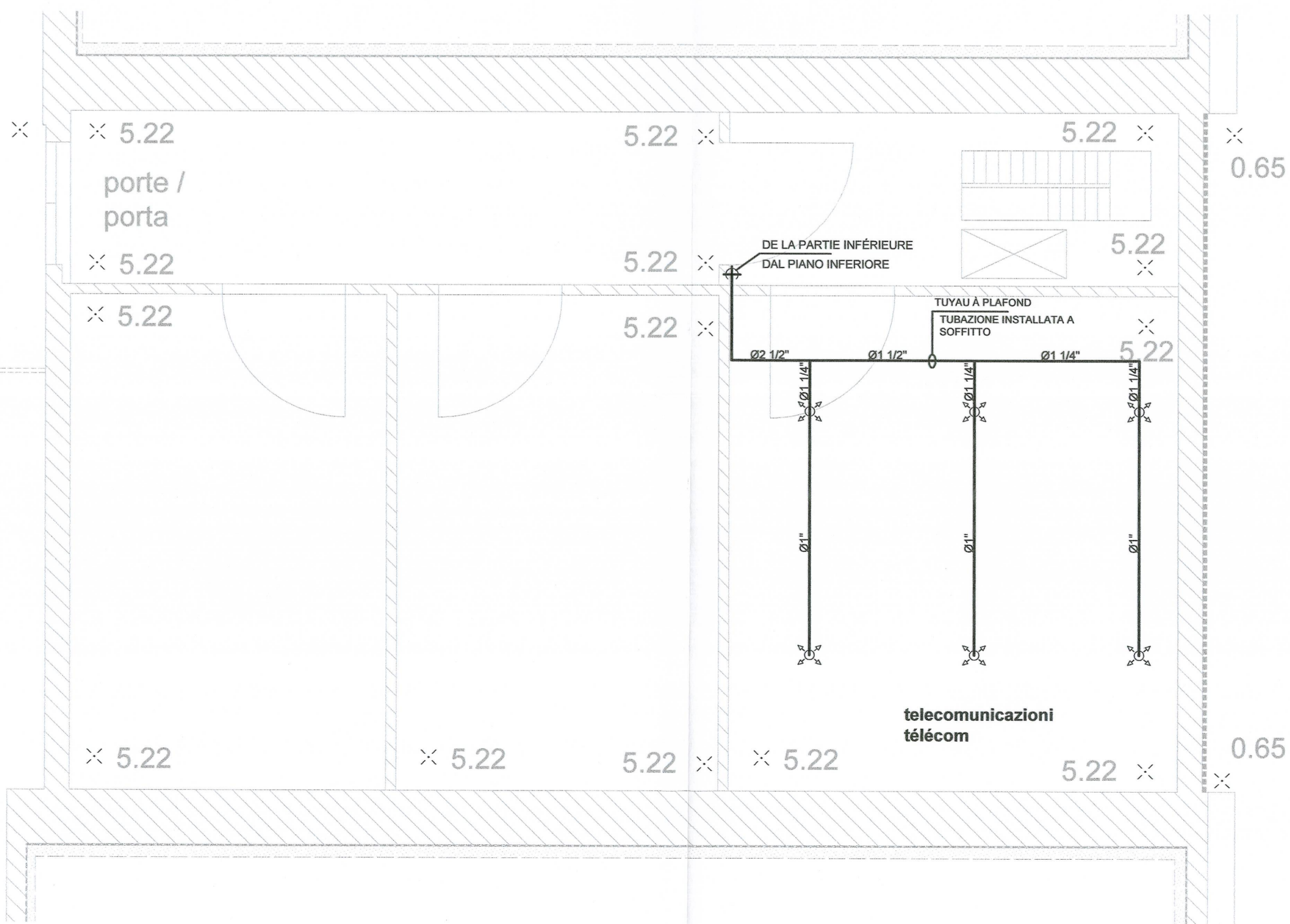
PLAN AU NIVEAU E2 - HAUTEUR 5,22 STRALCIO PIANTA PIANO E2 - QUOTA 5,22
