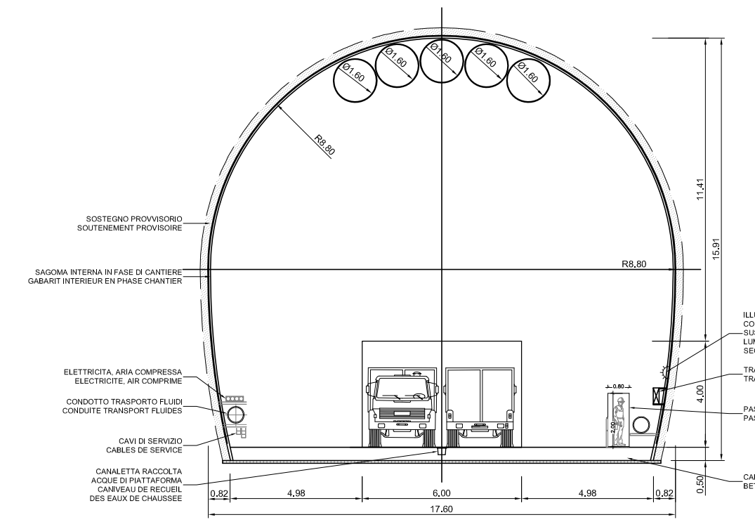
SEZIONE TIPO P-F CAVERNA TECNICA COUPE TYPE P-F CAVERNE TECHNIQUE
