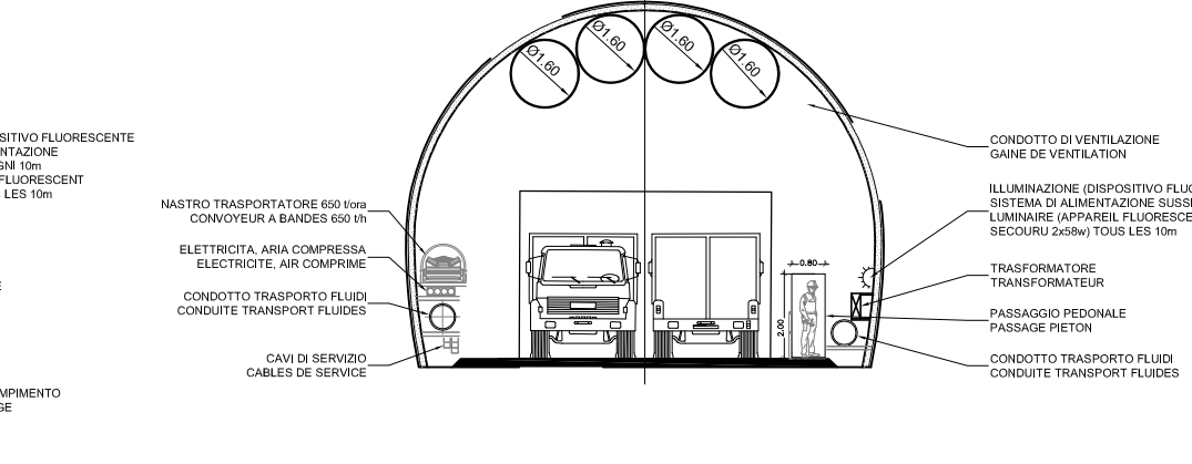
SEZIONE TIPO E-G GALERIA DI CONNESSIONE 2 COUPE TYPE E-G GALERIE DE CONNEXION 2
