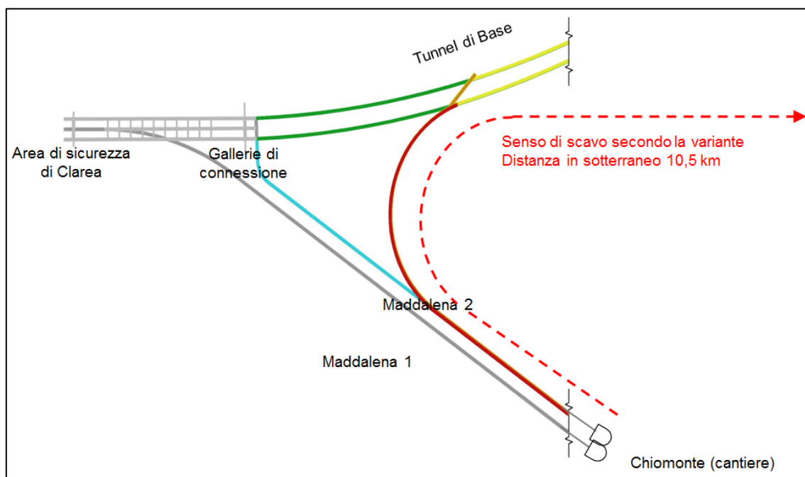
Figura 5 – Gallerie Maddalena (opere in sotterraneo)
