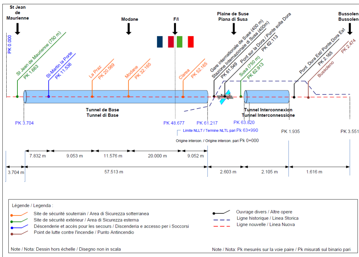
Figura 1 – Schema linea NLTL
