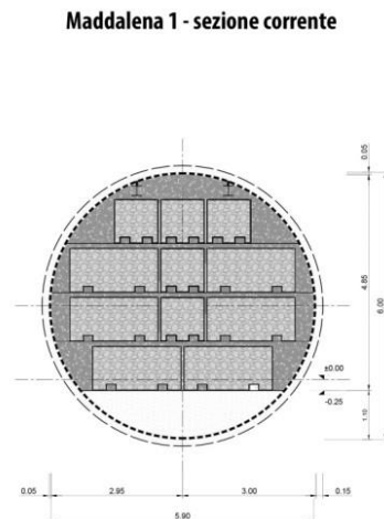
Figura 3 – Sezione corrente galleria di Maddalena 1 – stoccaggio rocce verdi
