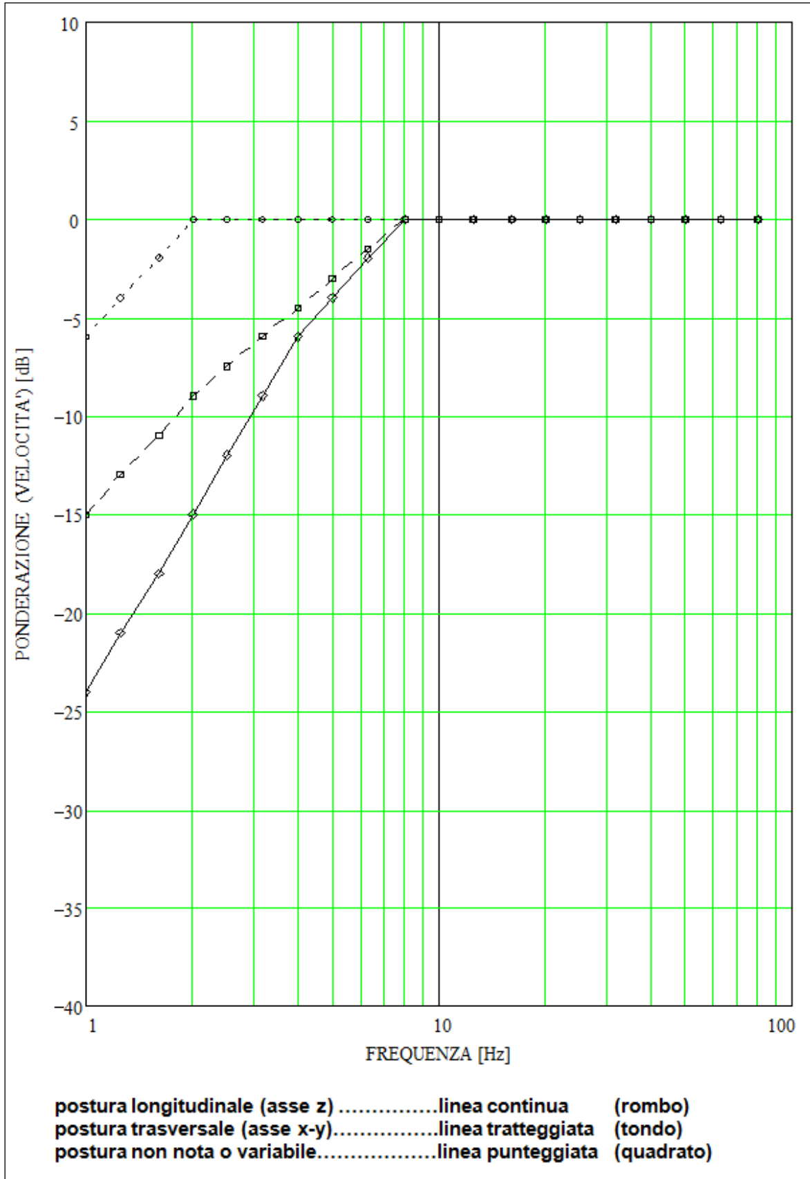
Figura 20 – Curve spettrali di ponderazione per le accelerazioni
