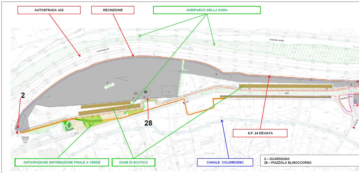
Figura 11 – Layout Susa Autoporto
