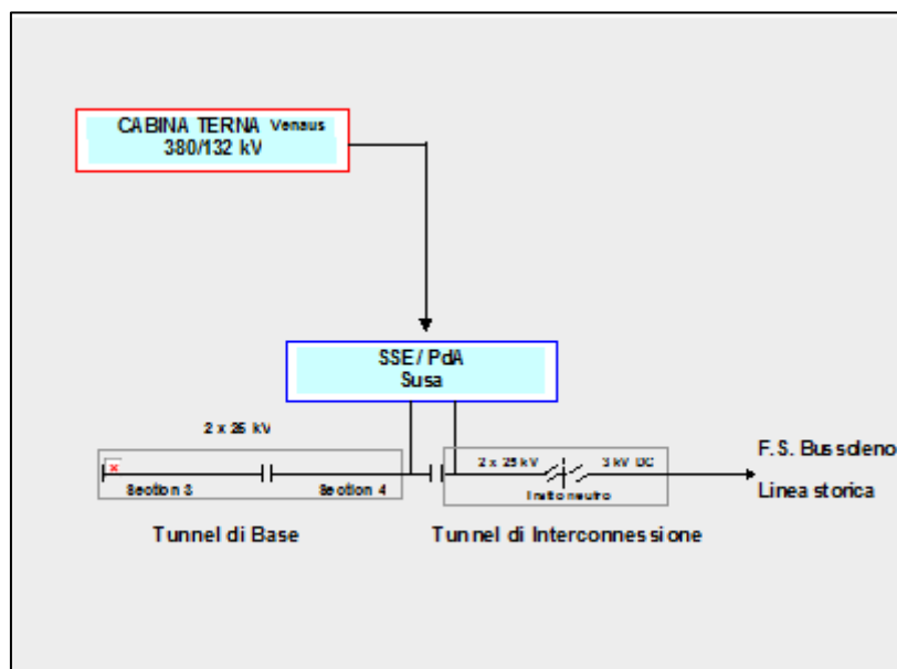
Figura 21 – Schema di alimentazione elettrica della linea NTLT
