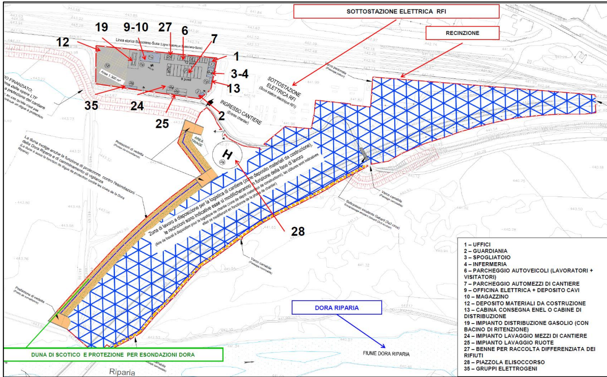
Figura 13 – Layout Innesto Bussoleno
