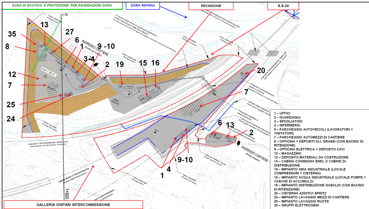
Figura 14 – Layout Imbocco Est Tunnel di Interconnessione
