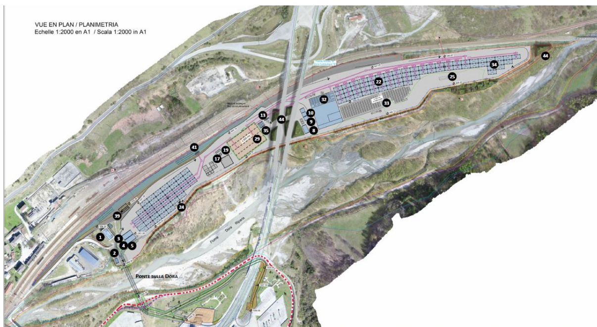
Figura 8 – Layout area industriale di Salbertrand (doc. rif. PRV_TS3_C3C_7207: Album di inquadramento dei cantieri oggetto di variante)
