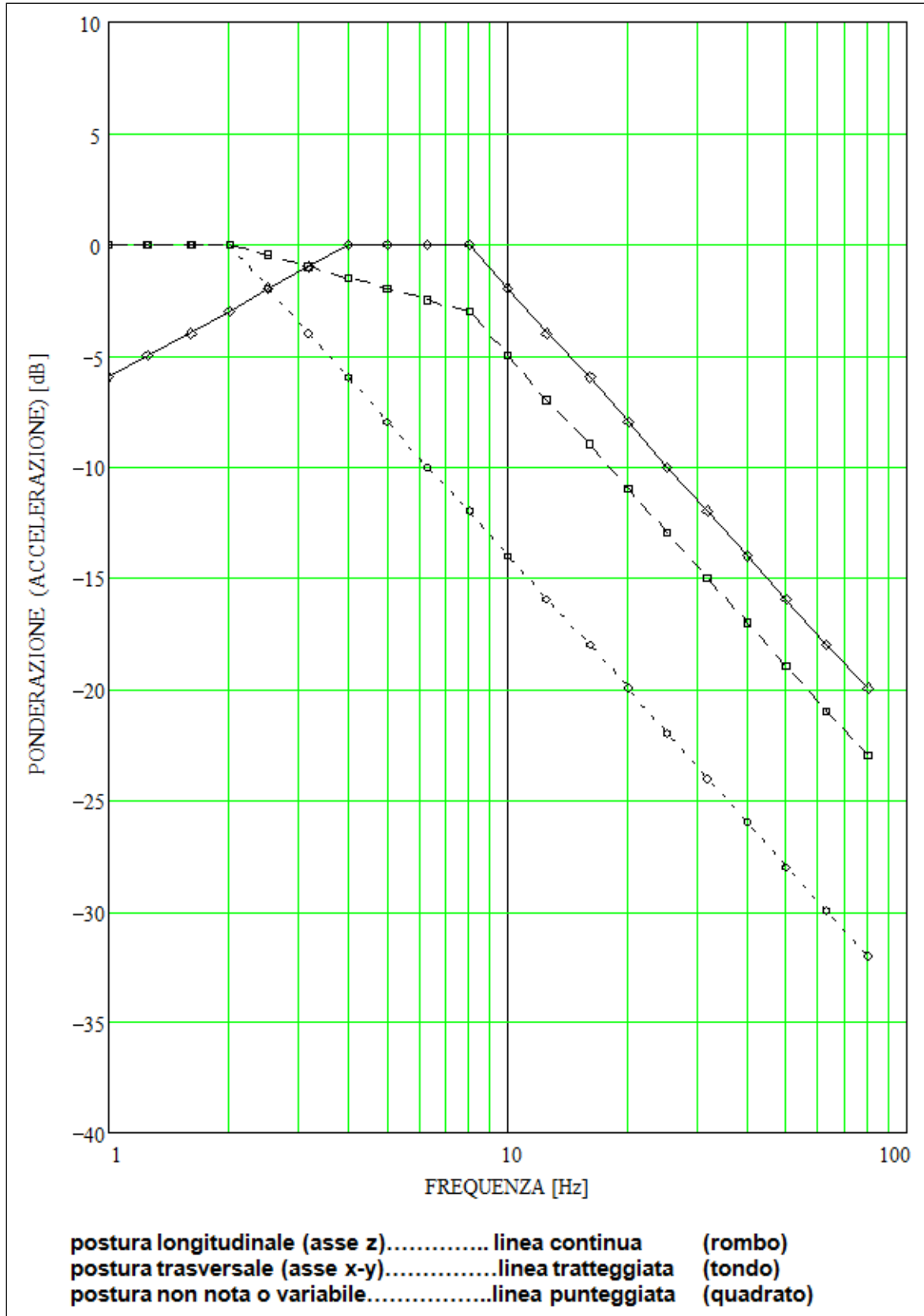
Figura 19 – Curve spettrali di ponderazione per le accelerazioni
