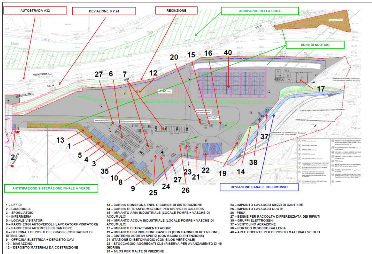
Figura 12 – Layout Imbocco Ovest TdI
