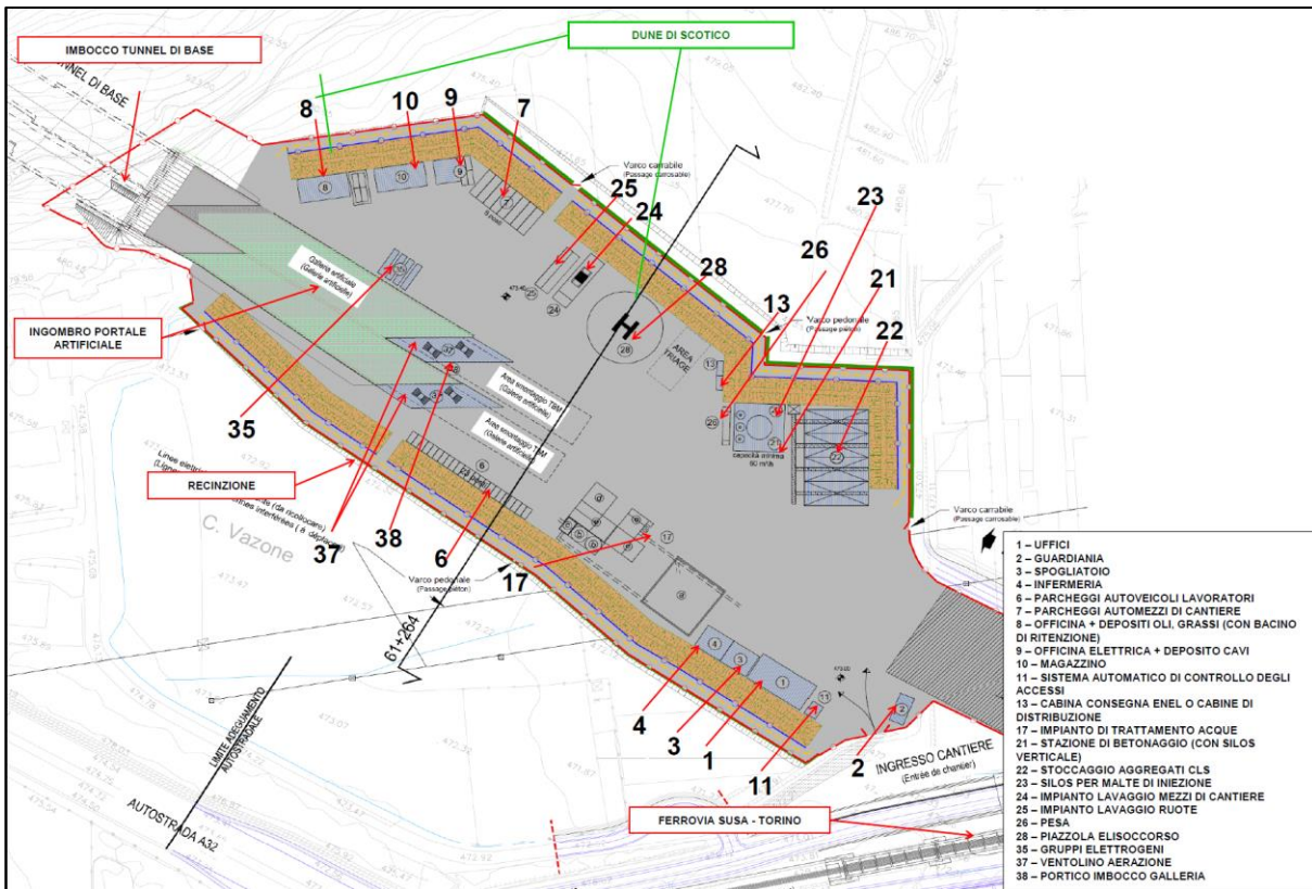
Figura 10 – Layout Imbocco Est TdB
