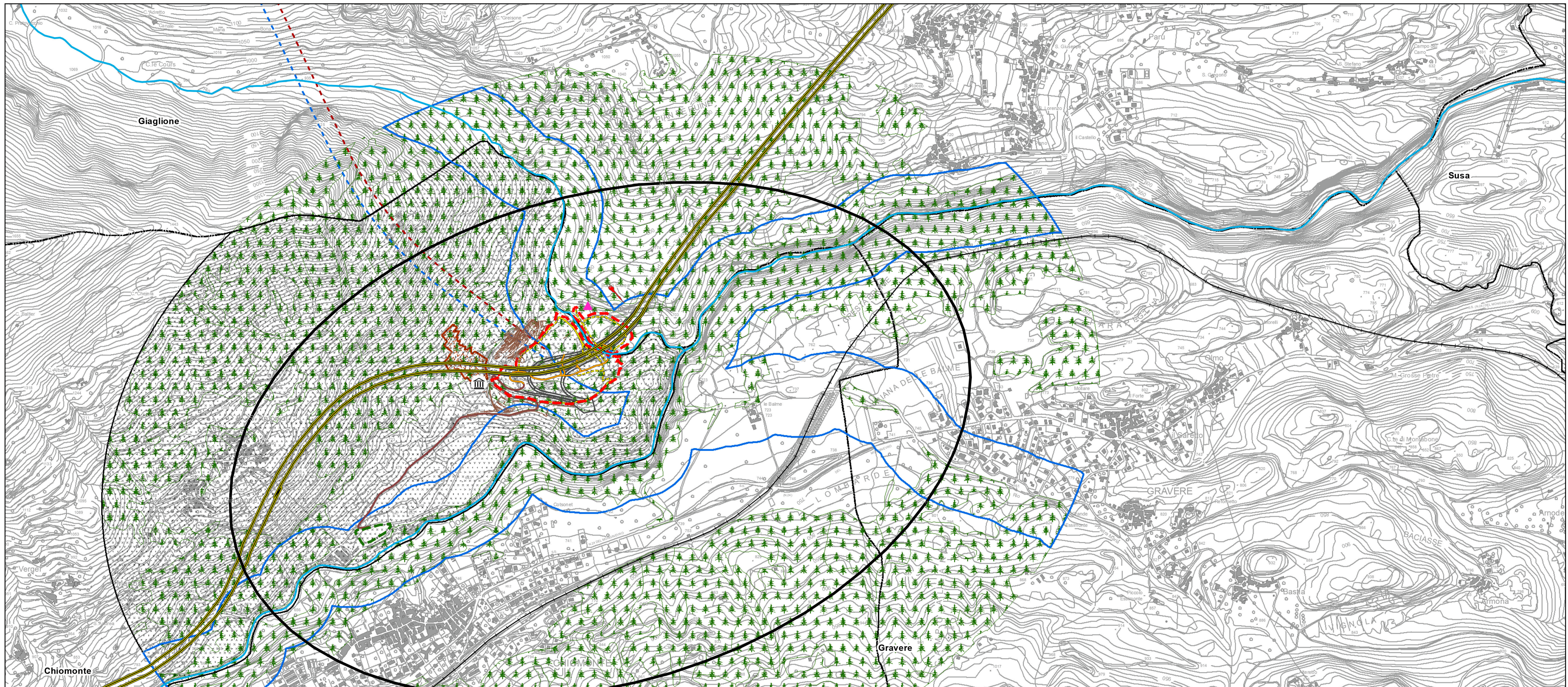
COMPARAZIONE AREE DI CANTIERE NELLE DIVERSE FASI AUTORIZZATIVE - Scala 1:5000
