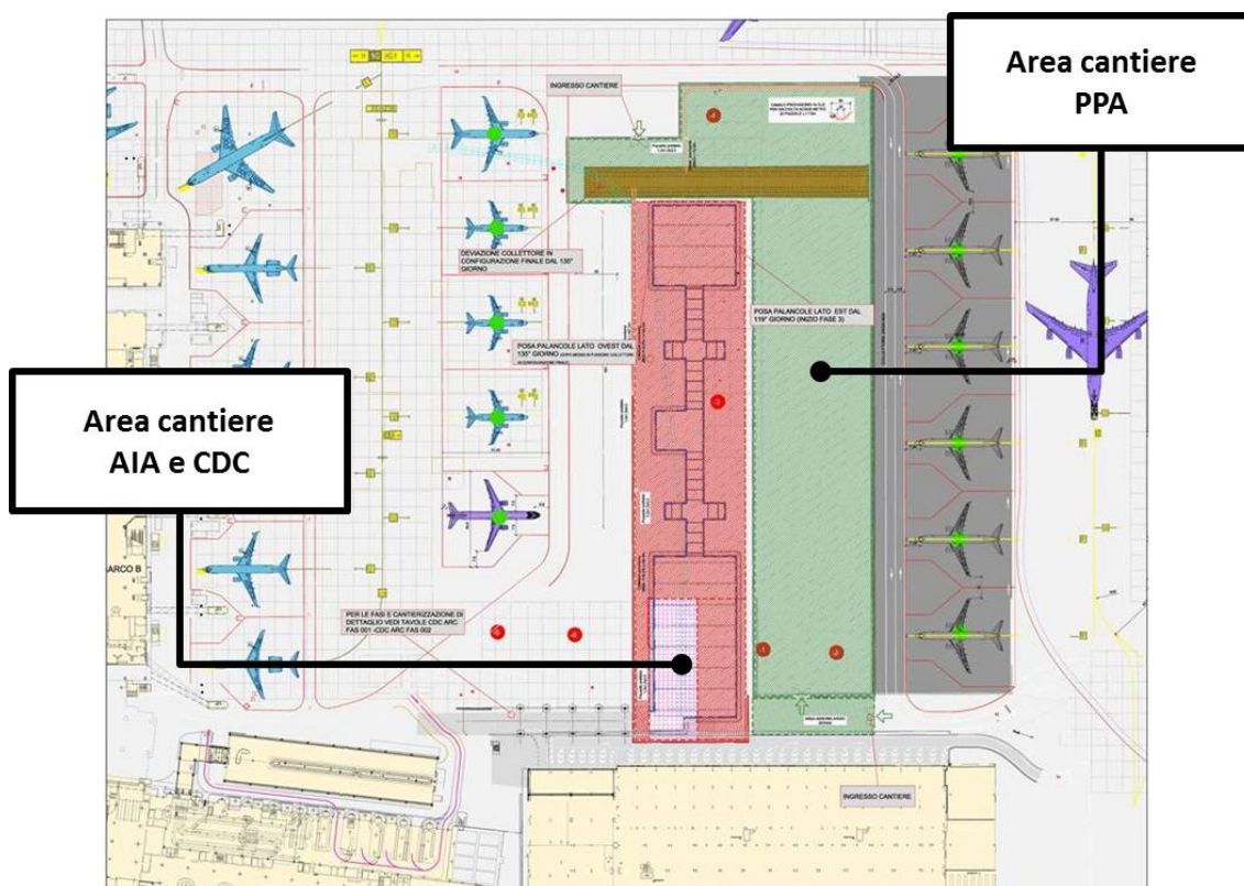
Figura 7-16 Sovrapposizione dei cantieri relativi alla realizzazione dell'Area di imbarco A (AIA), del Corpo di collegamento (CDC) e dei piazzali aeromobili di pertinenza Area di imbarco A (PPA).
