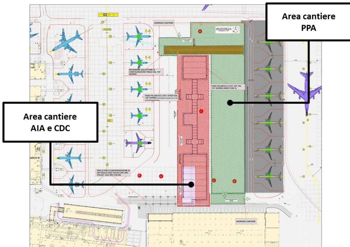
Figura 7-10 Sovrapposizione dei cantieri relativi alla realizzazione dell'Area di imbarco A (AIA), del Corpo di collegamento (CDC) e dei piazzali aeromobili di pertinenza Area di imbarco A (PPA).
