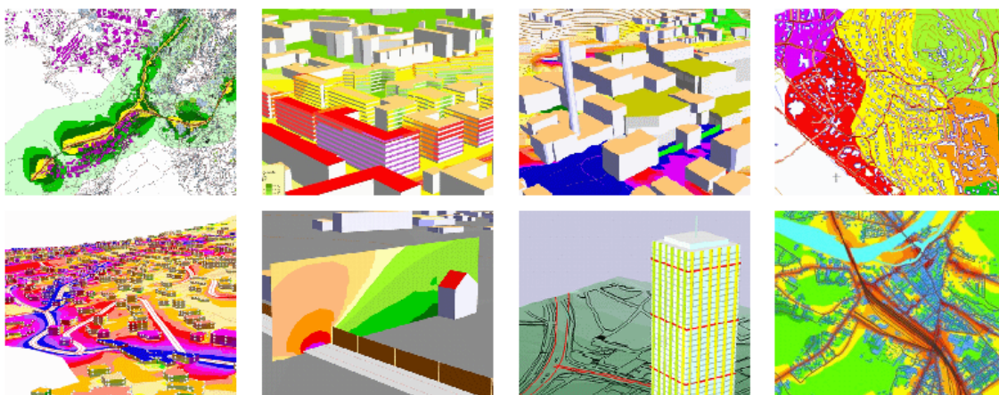
Figura 7-14 SoundPlan – esempio di output del modello in 2D e 3D della mappatura acustica
