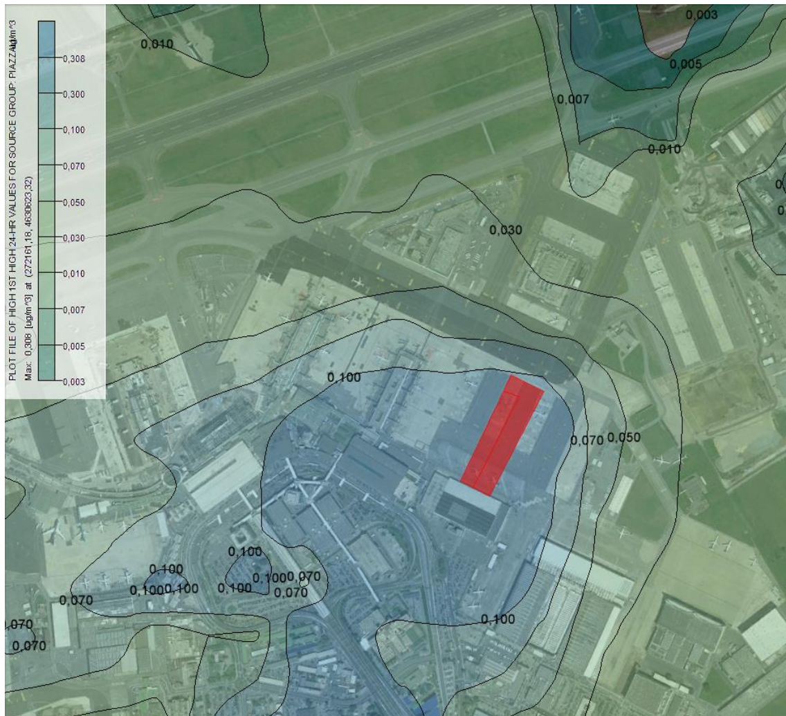
Figura 7-12 Massimi sulla maglia di calcolo media 24h PM 10 Fase 1
