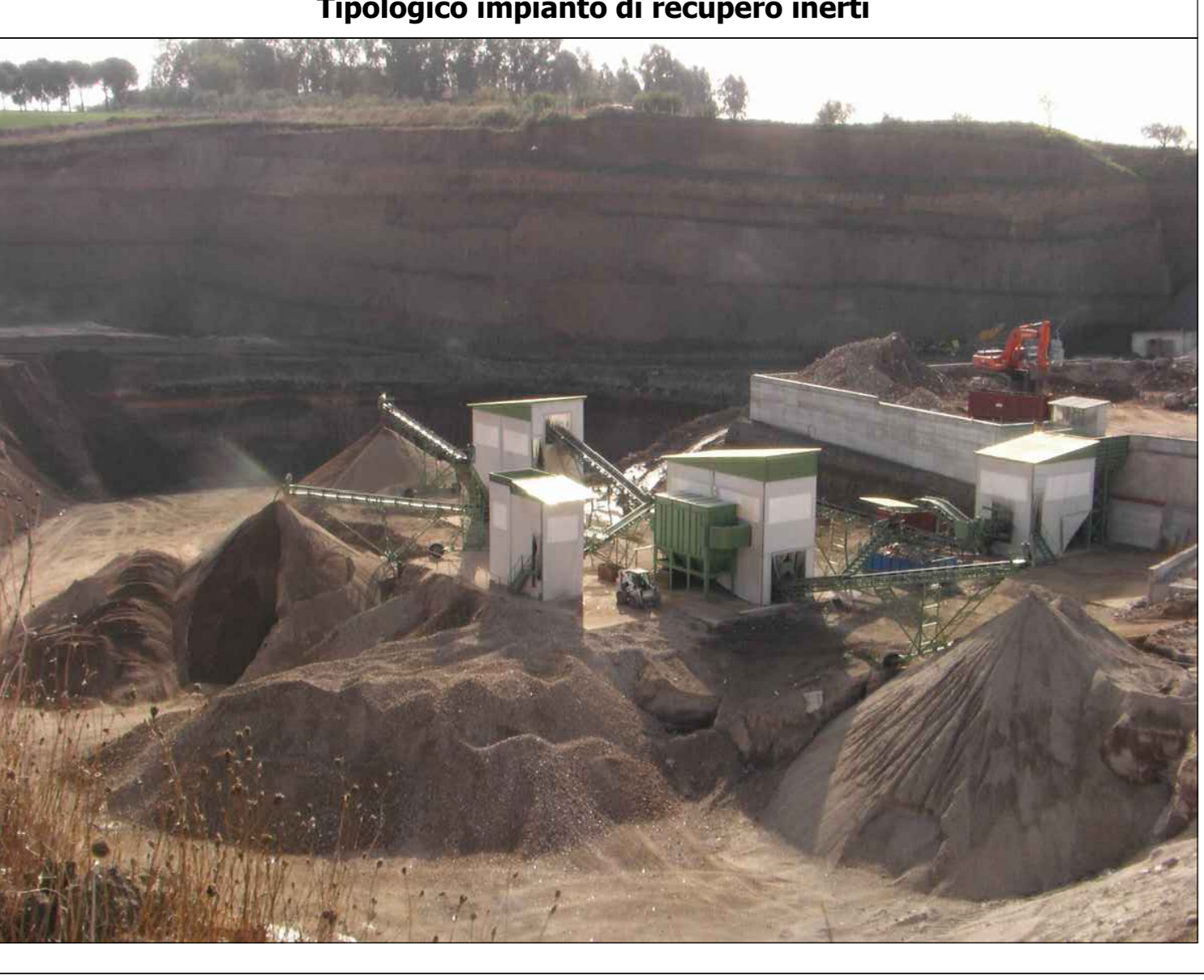
Tipologico impianto di recupero inertii
