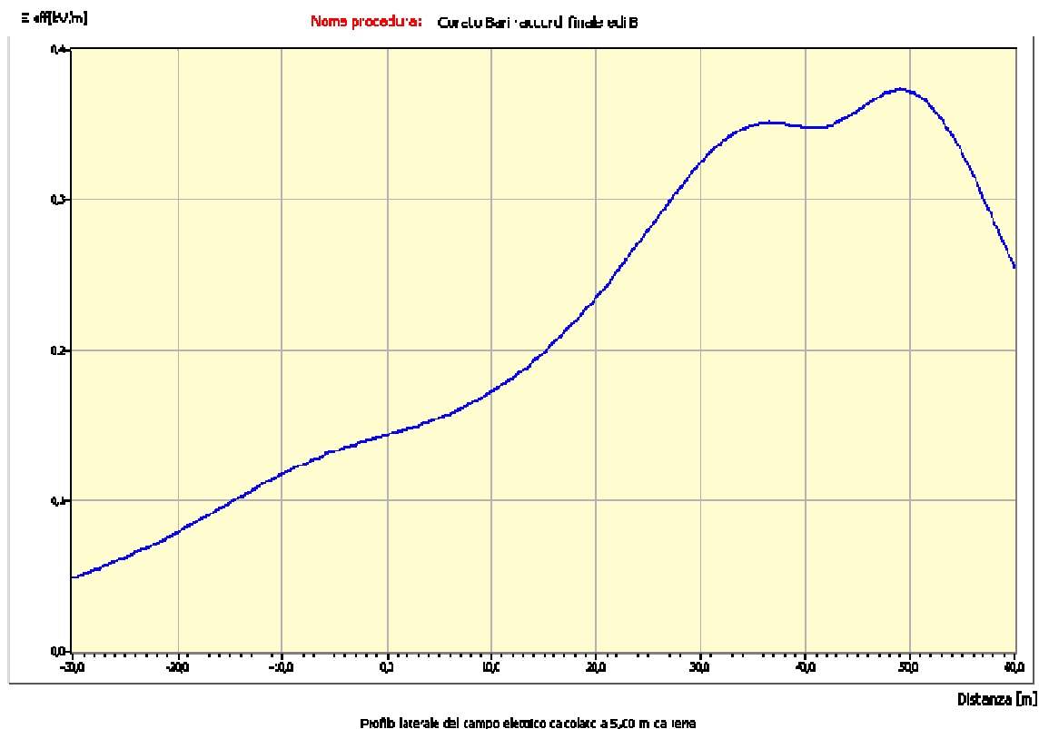
Campo elettrico a 5 m di altezza
