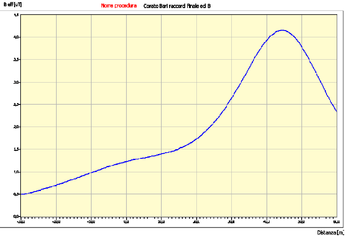
Profilo laterale dell'induzione magnetica calcolata a 5,00 m da terra
