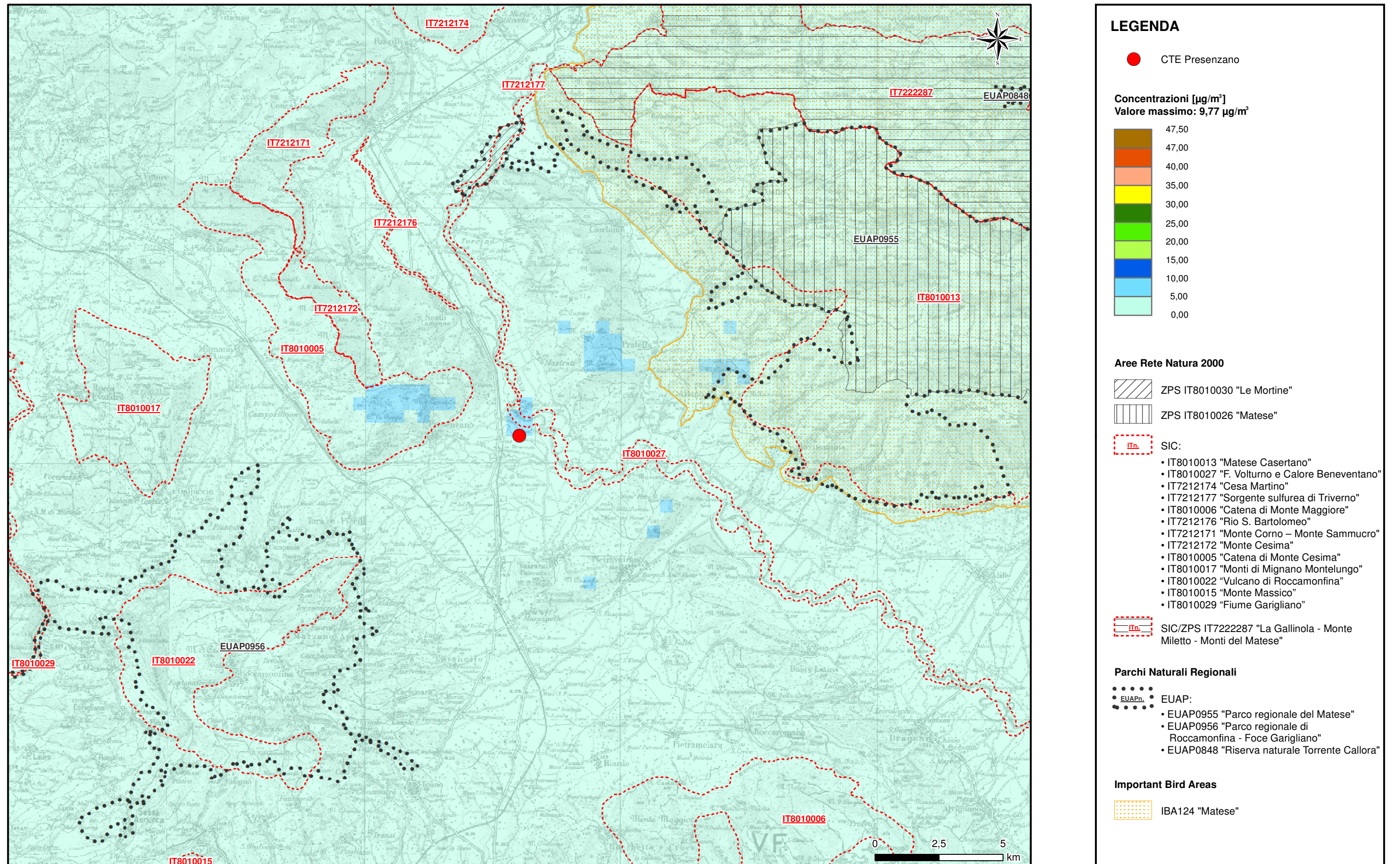
Figura 4.7.2a ScENARIO futuro: 99,8° percentile delle concentrazioni medie orarie di NO x
