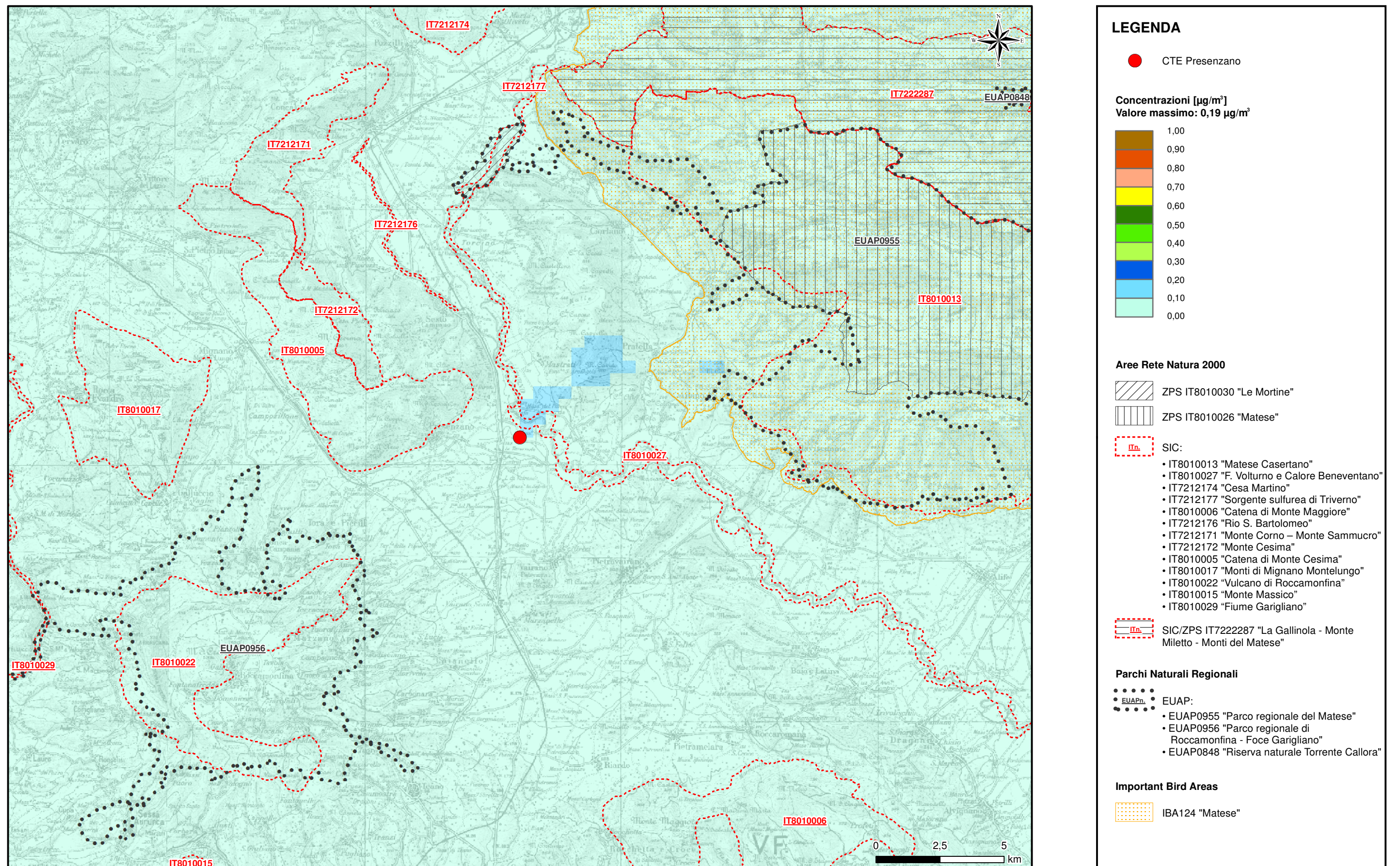
Figura 4.7.2b Scenario futuro: concentrazione media annua di NOx
