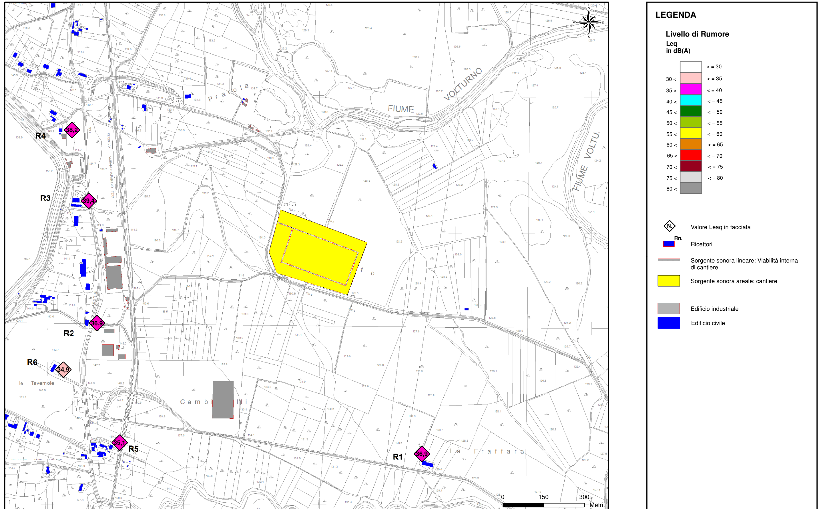
Figura 5.2.2a Livello equivalente dBA ai ricettori limitrofi alla Centrale nella fase di cantiere - periodo diurno
