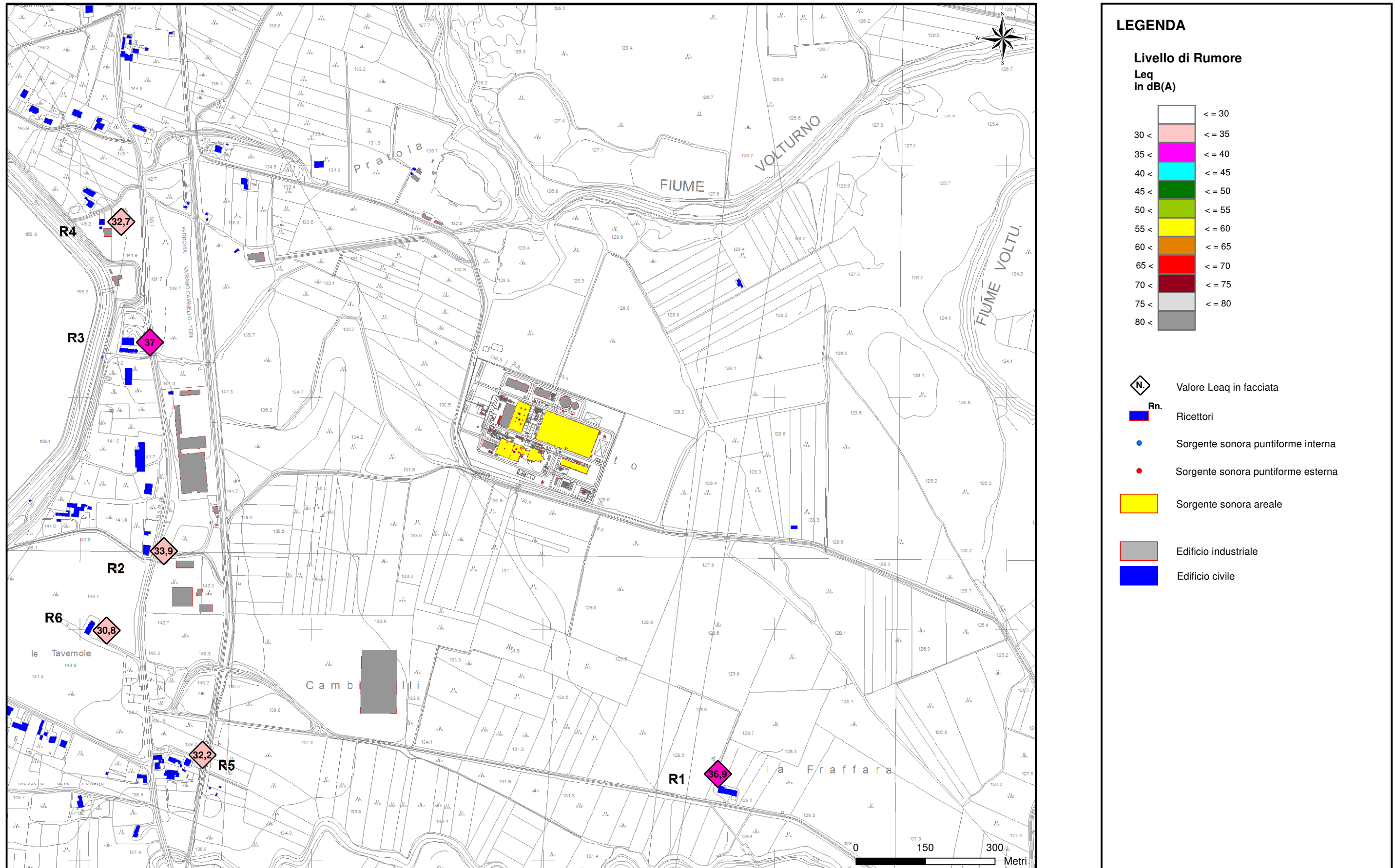
Figura 5.3.2a Livello equivalente dBA ai ricettori limitrofi alla Centrale nella fase di esercizio - periodo diurno
