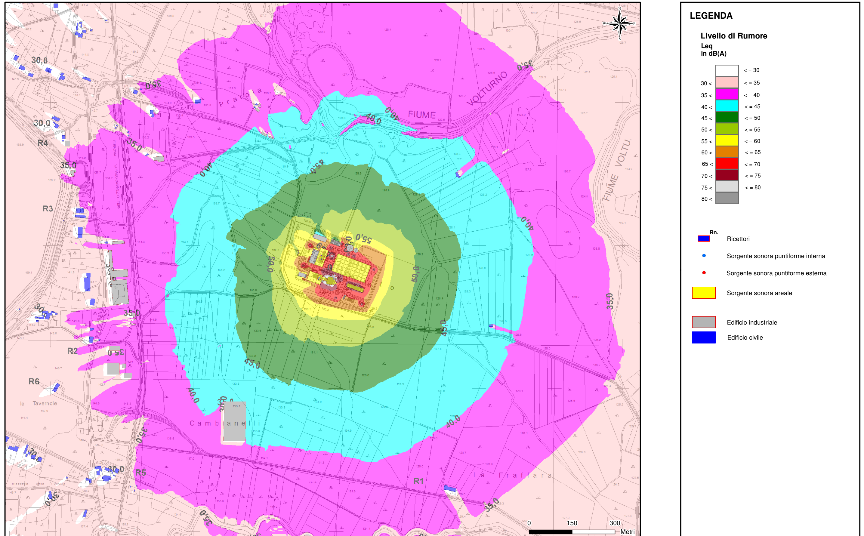
Figura 5.3.2b Isofoniche nella fase di esercizio della Centrale - periodo diurno
