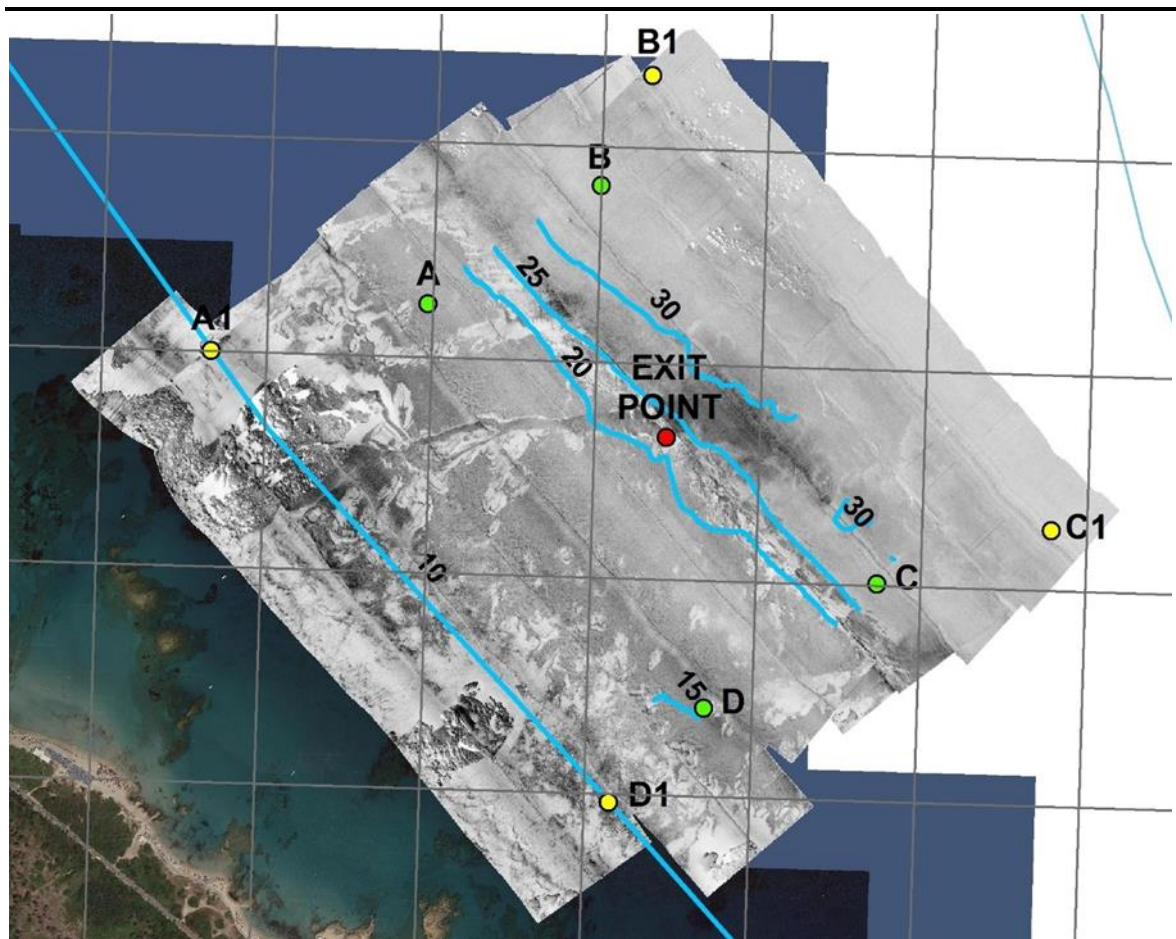
Figura 2.1 La carta con i risultati del rilievo side scan sonar montata sulle foto satellitari della linea di costa (riduzione, originale in scala 1:2.000)
