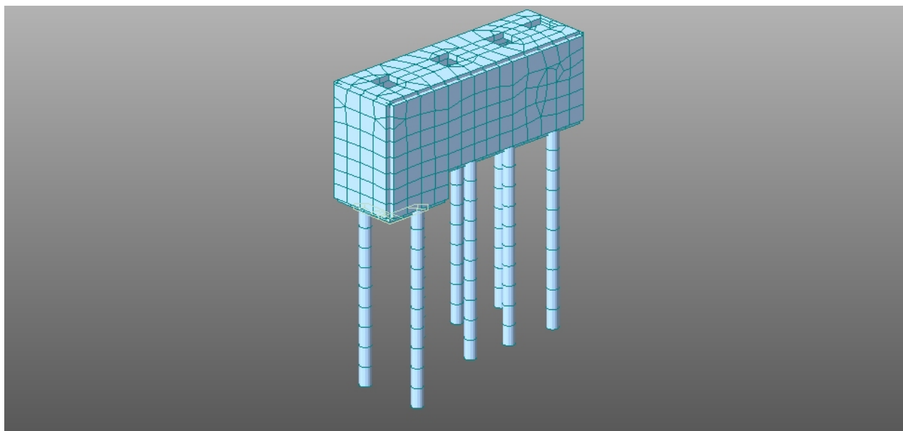
Vista assonometrica del modello F.E.M.
