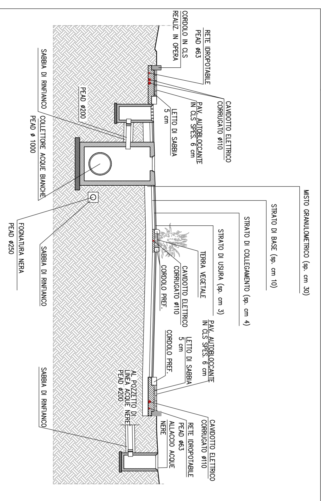
Sezione tipo V.S. 28B - V.S. 28D scala 1:100
