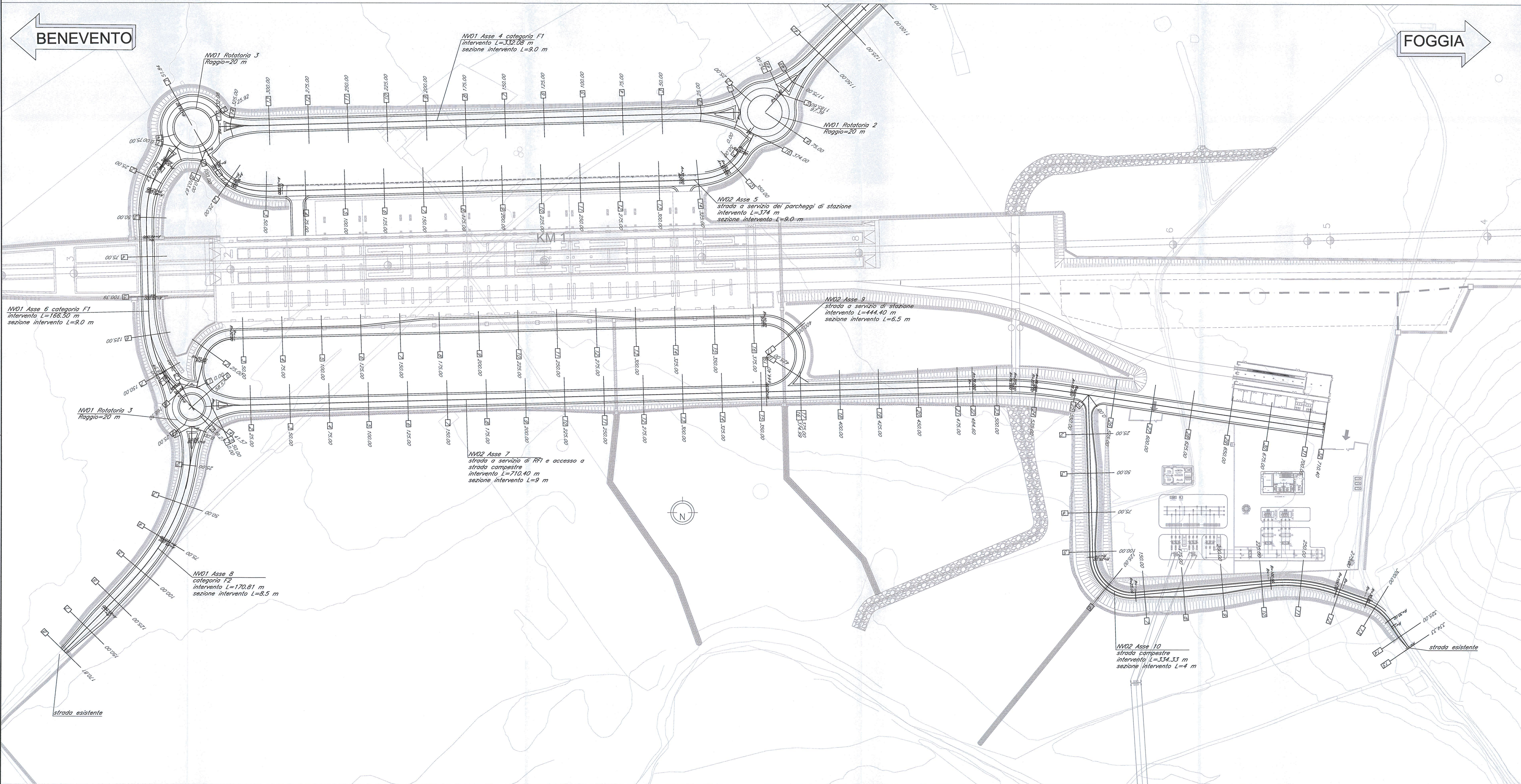
PLANIMETRIA ASSE 5-7-9 E 10
