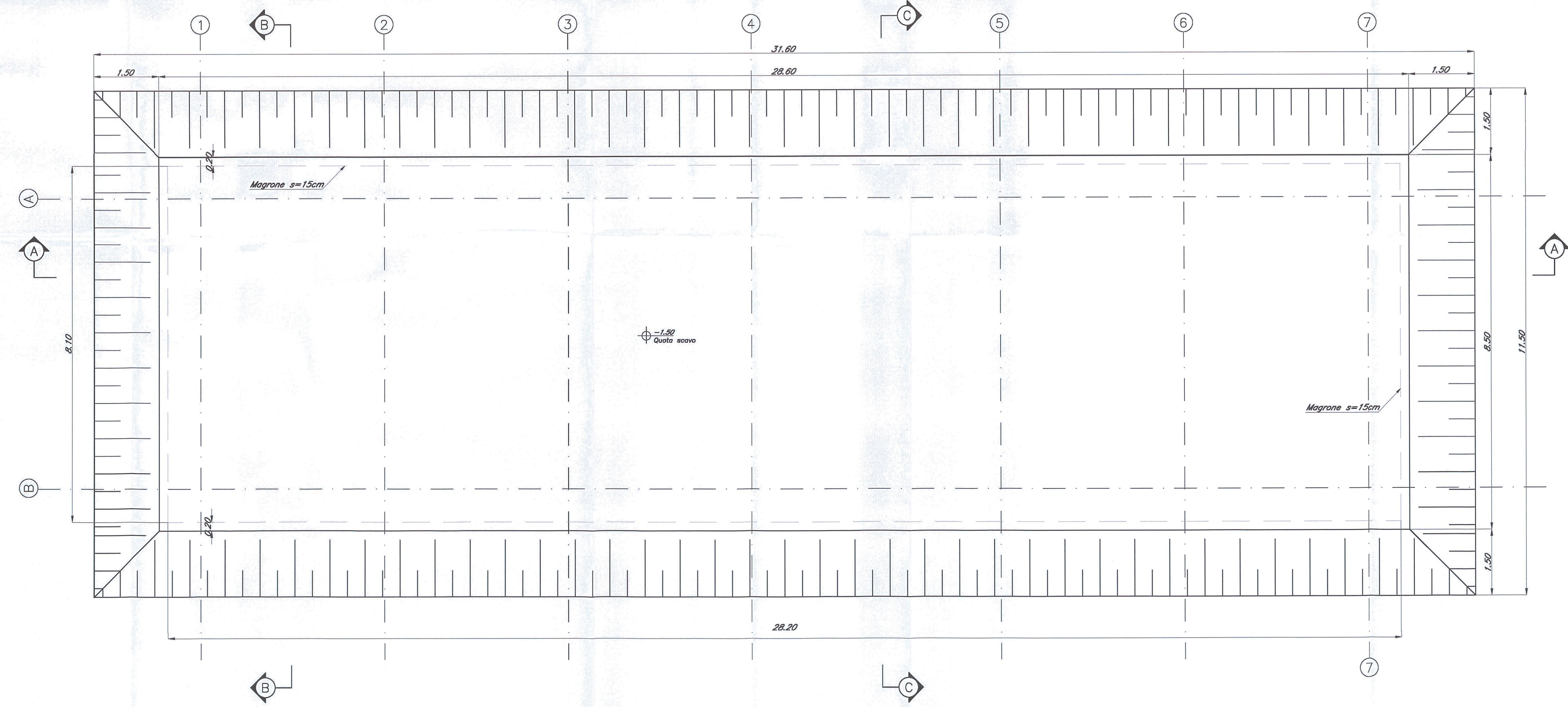
PIANTA SCAVI Scala 1:50
