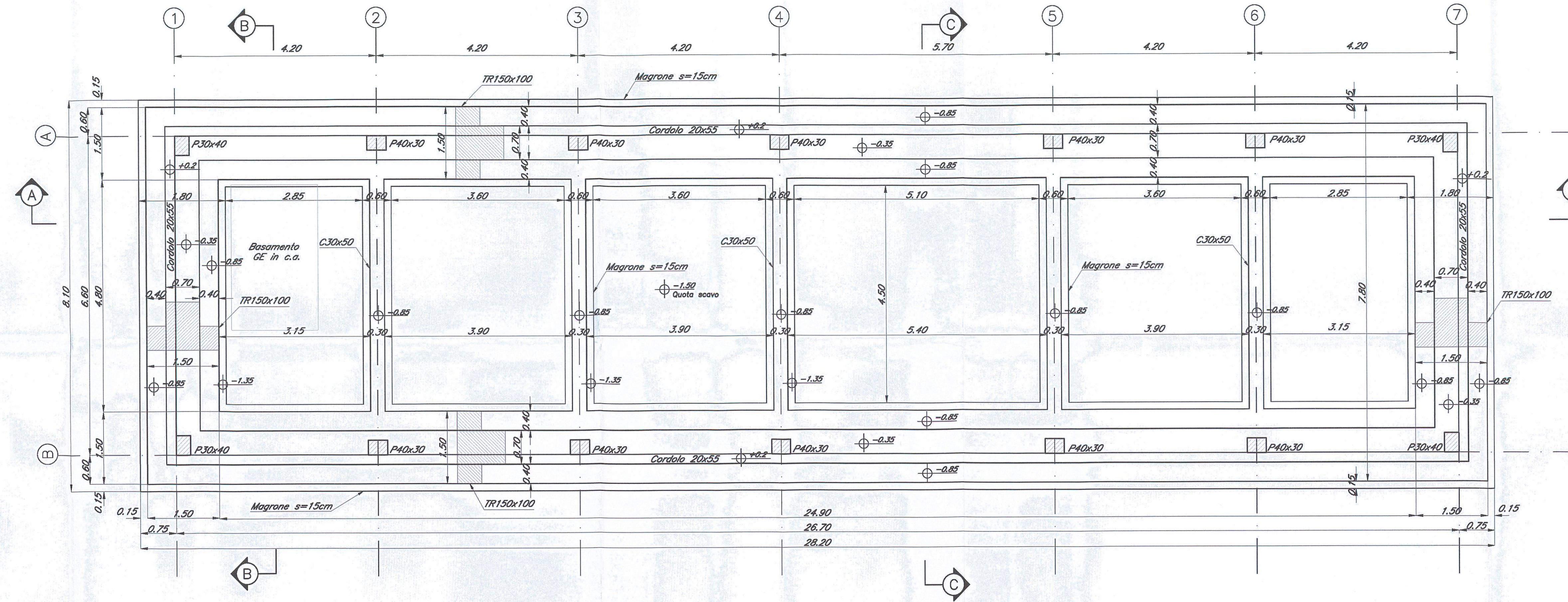
PIANTA CARPENTERIA FONDAZIONE Scala 1:50
