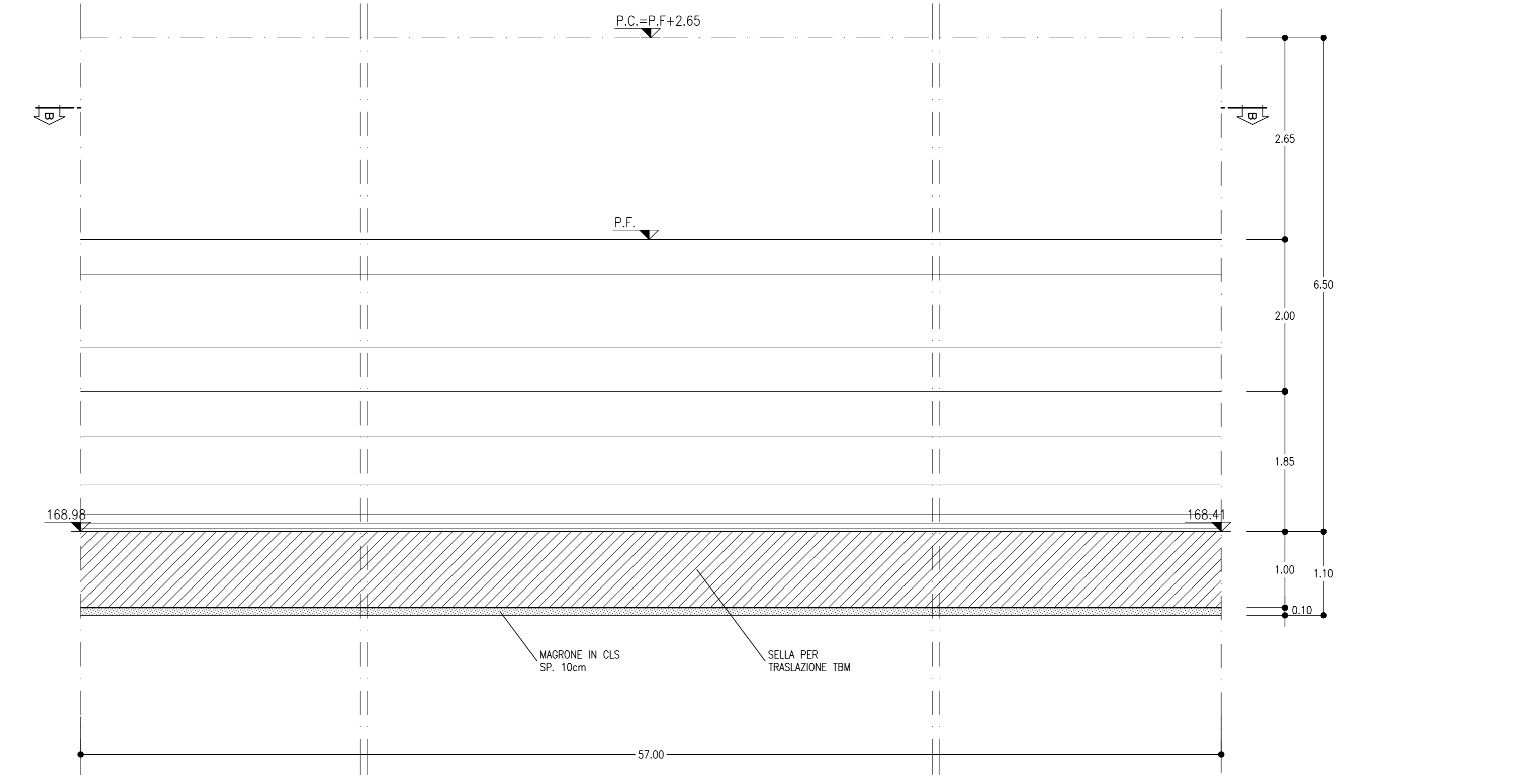
SELLA TRASLAZIONE TBM SCALA 1:50 SEZIONE A-A
