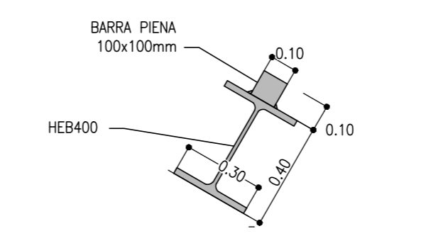
SELLA TRASLAZIONE TBM SCALA 1:50 SEZIONE A-A
