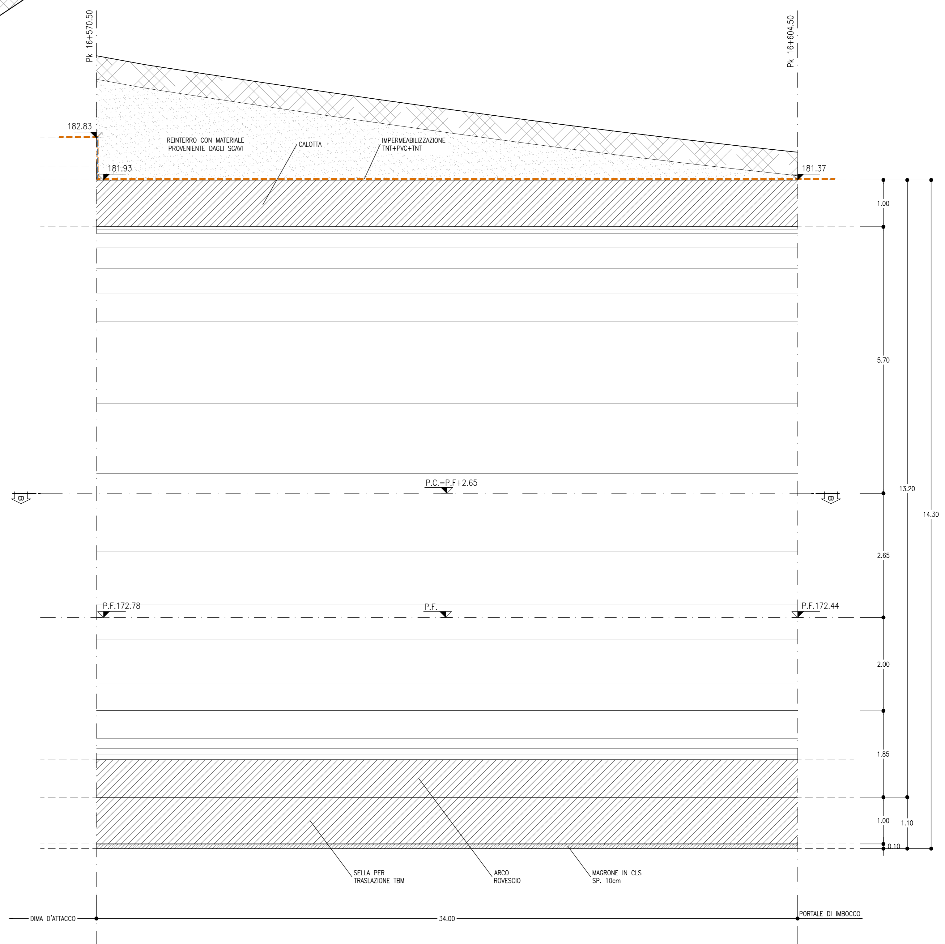
PARTICOLARE "A" SCALA 1:20
