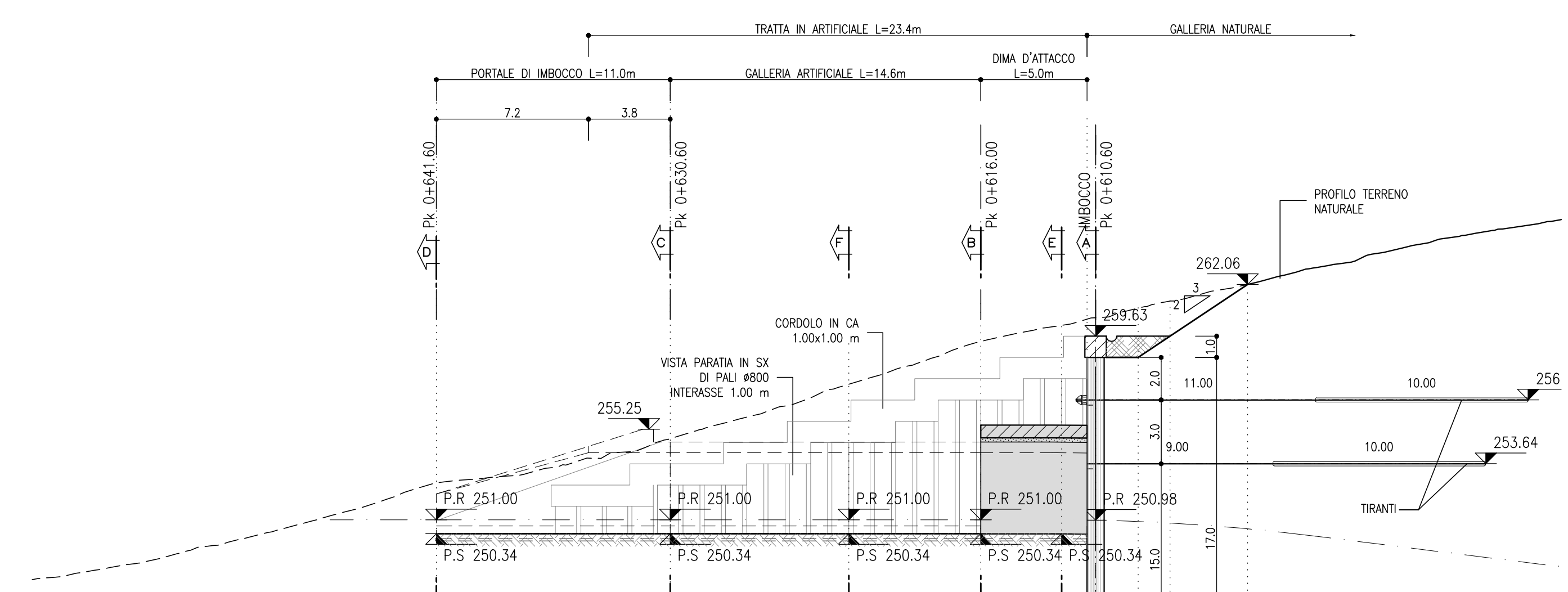
PROFILO LONGITUDINALE SCALA 1:200
