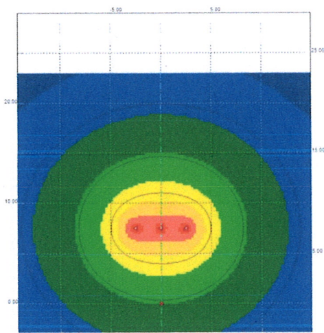
Fig.2 – Fascia di rispetto a 3 µT su terna di sbarre AT (I=200 A)
