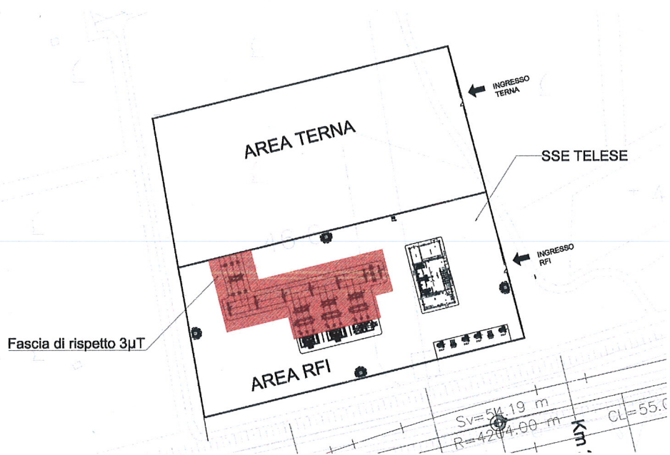
Fig.1 – Fascia di rispetto a 3 µT
