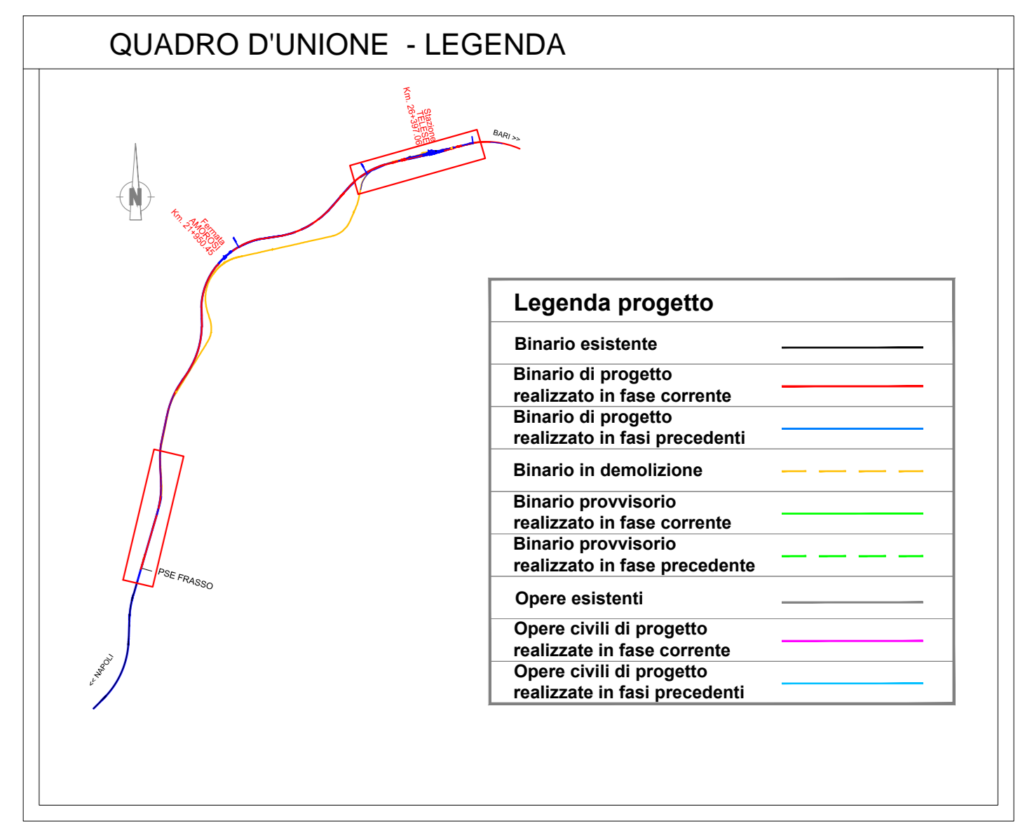
Inquadramento da inizio Lotto al Km 18+400
