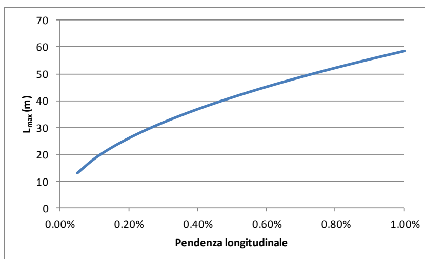
Fig. 7 – Distanza minima degli scarichi in rilevato
