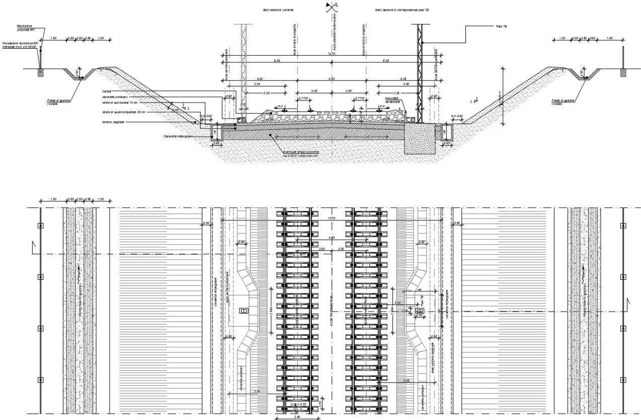
Fig. 4 – Sezione ferroviaria in trincea a doppia linea
