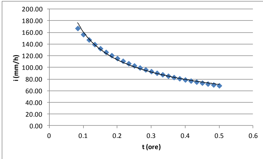
Fig. 1 – Interpolazione per Tr 100 anni
