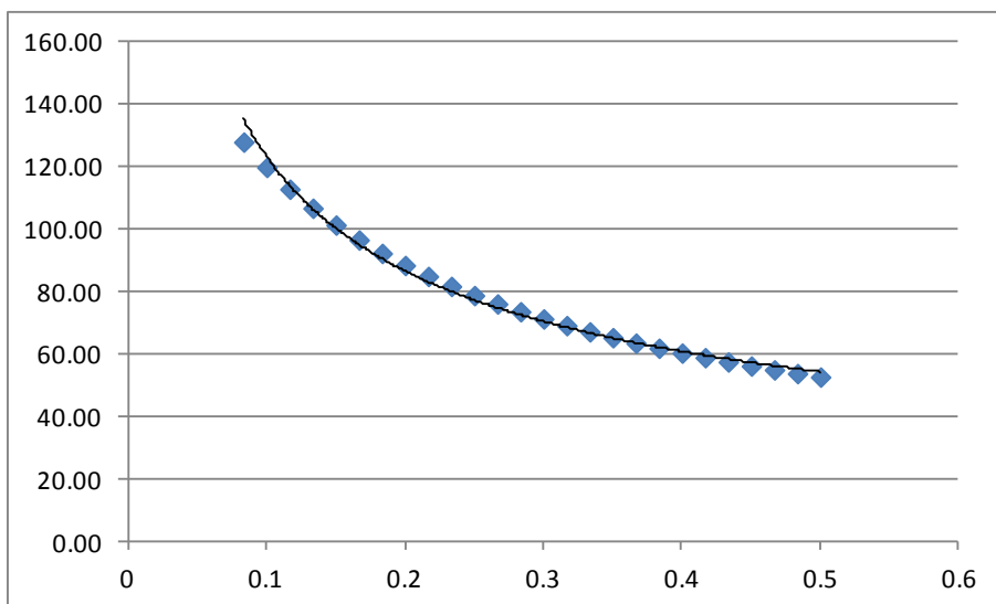
Fig. 2 – Interpolazione per Tr 25 anni
