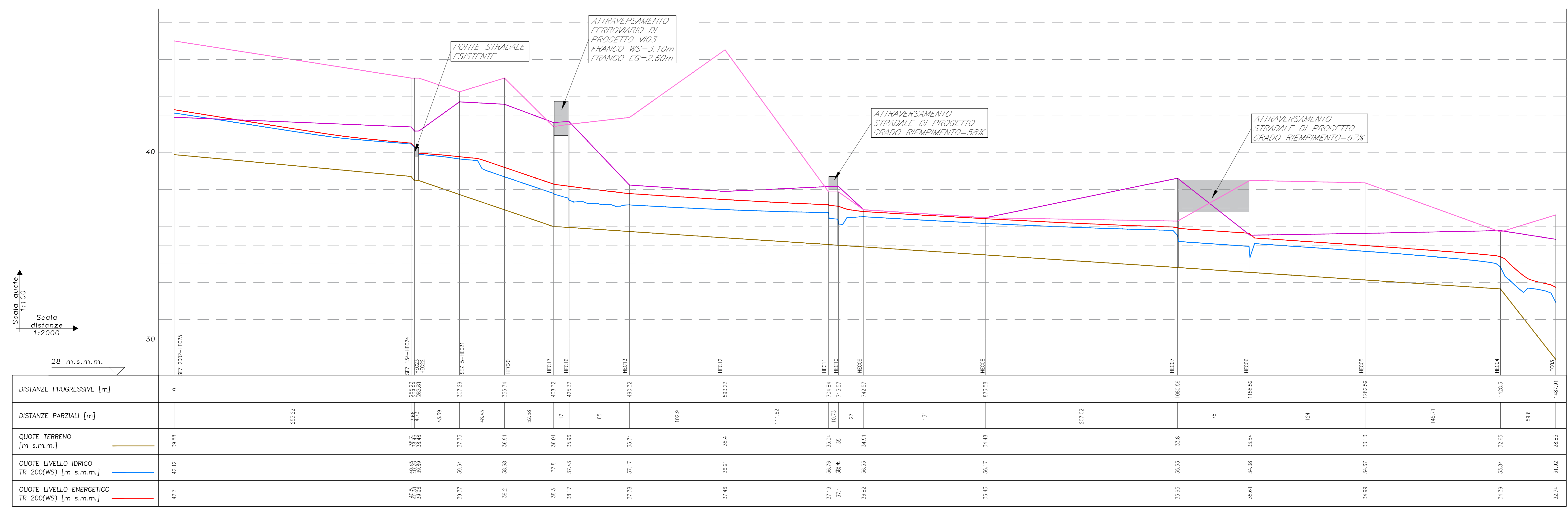
PROFILO IDRICO POST OPERAM
