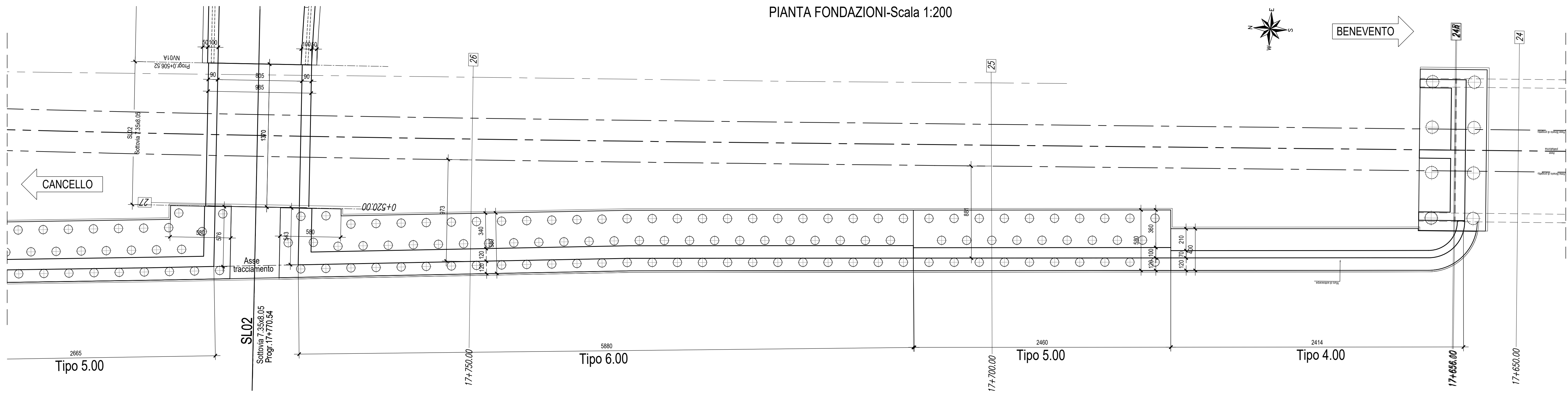
PIANTA FONDAZIONI-Scala 1:200
