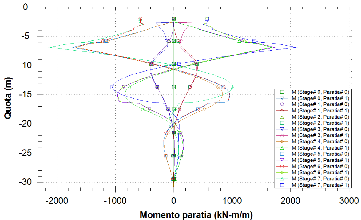
Figura 34 – SLE – Momento Flettente
