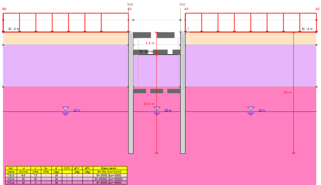
Figura 13 – Esecuzione scavo iniziale fino ad intradosso solettone intermedio(step 1)
