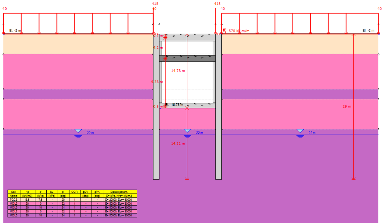
Figura 30 – Sistemazione finale (step 6)
