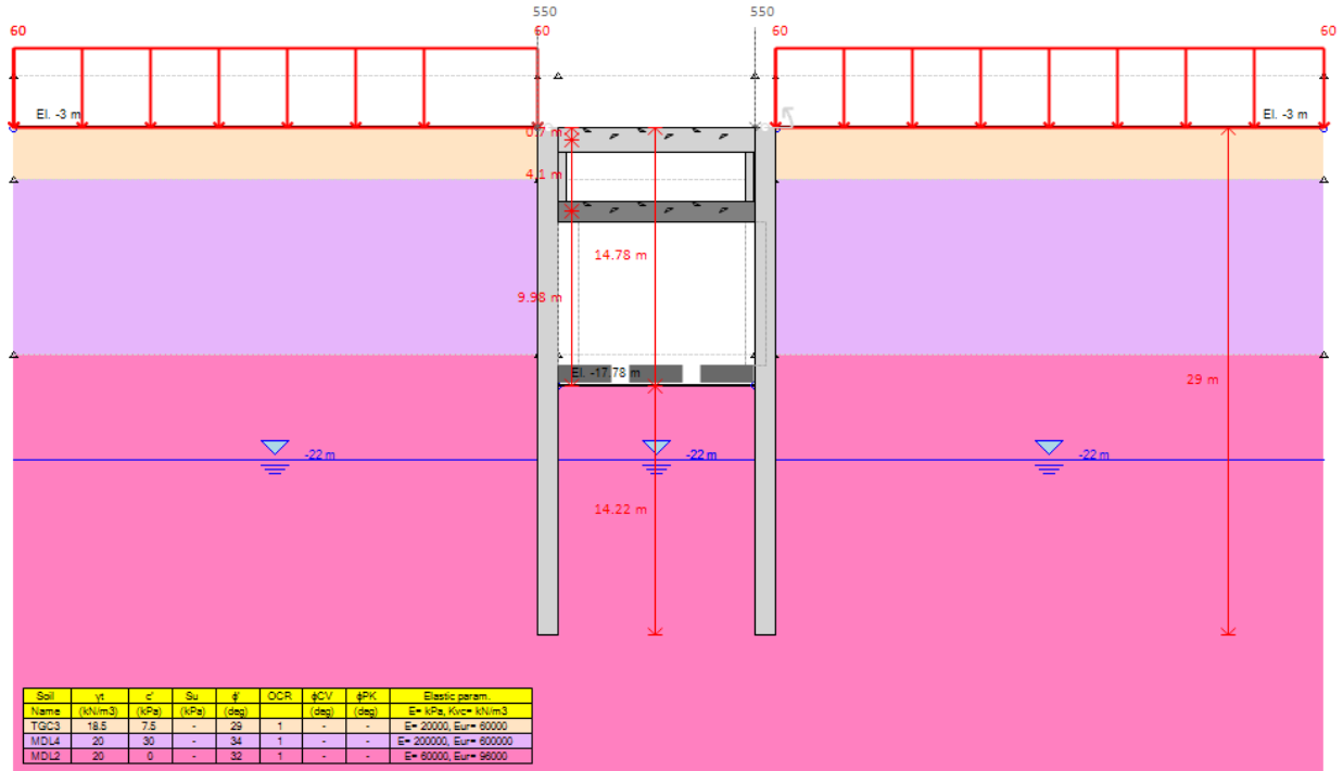
Figura 16 – Esecuzione scavo a foro cieco fino ad intradosso solettone di base (step 3)
