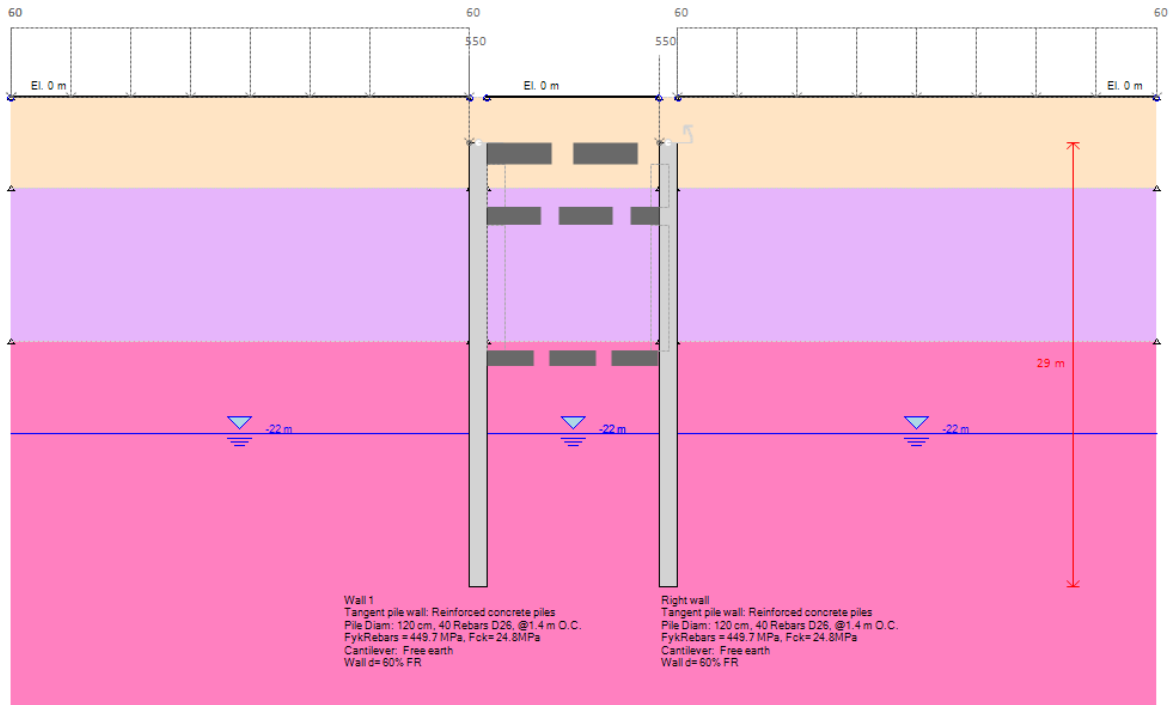
Figura 12 – Esecuzione pali \varphi=1200 mm ed inizializzazione geostatica (step 0)
