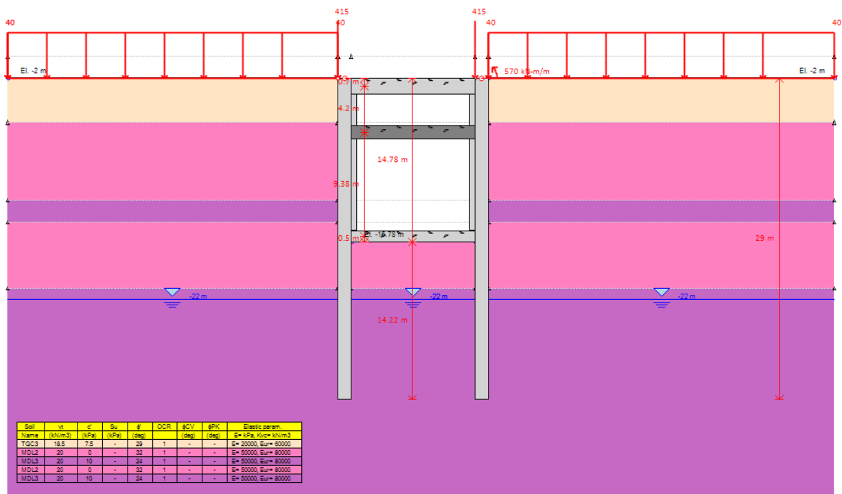
Figura 31 – Attivazione sisma (step 7)
