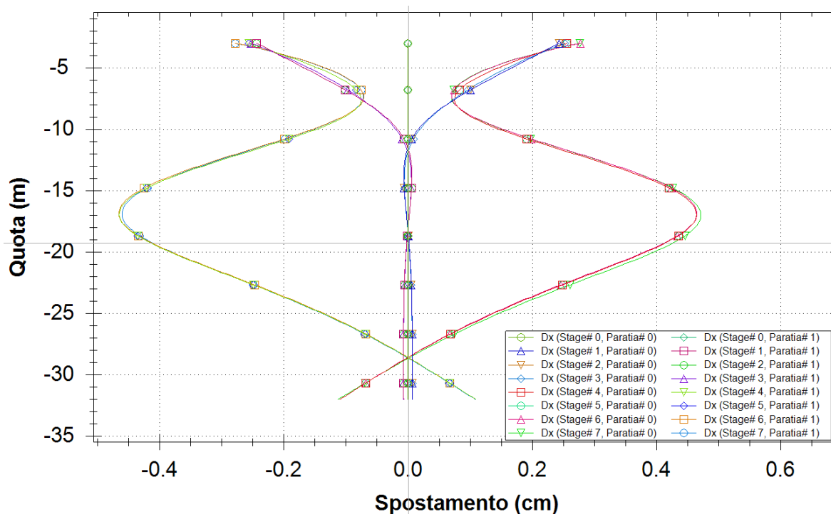
Figura 23 – SLE - Deformazioni Fase per Fase
