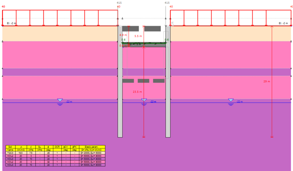
Figura 26 – Realizzazione solettone intermedio (step 2)
