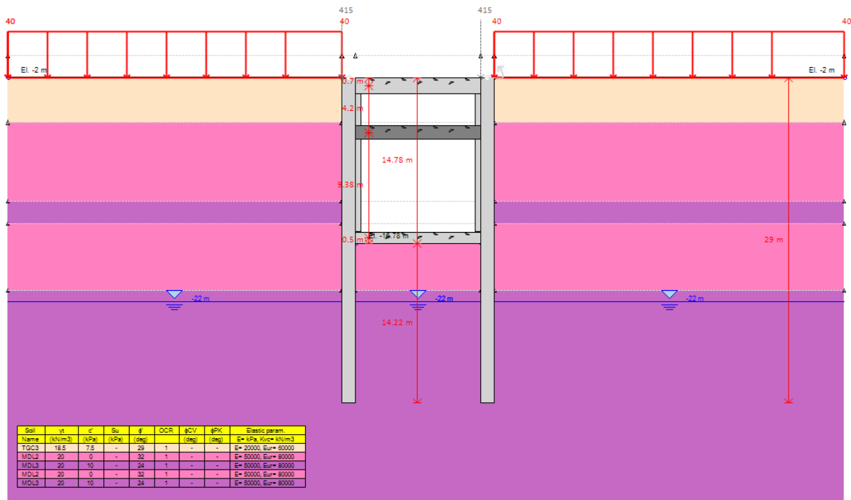
Figura 29 – Realizzazione solettone di base e pareti di rivestimento camera inferiore (step 5)
