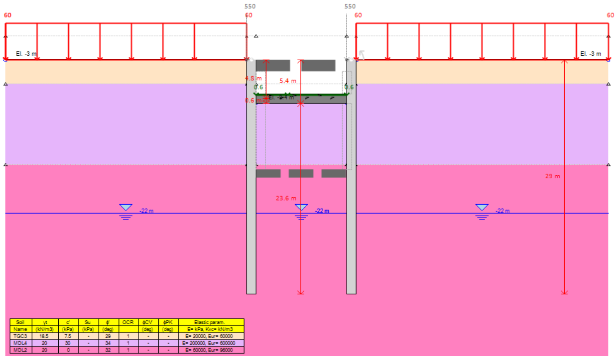
Figura 14 – Realizzazione solettone di intermedio (step 2)
