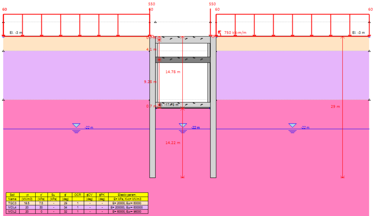
Figura 18 – Sistemazione finale (step 5)
