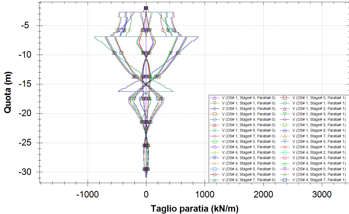
Figura 33 – A1-M1-R1(Statica "DS#1" e Sismica "DS#4") – Taglio
