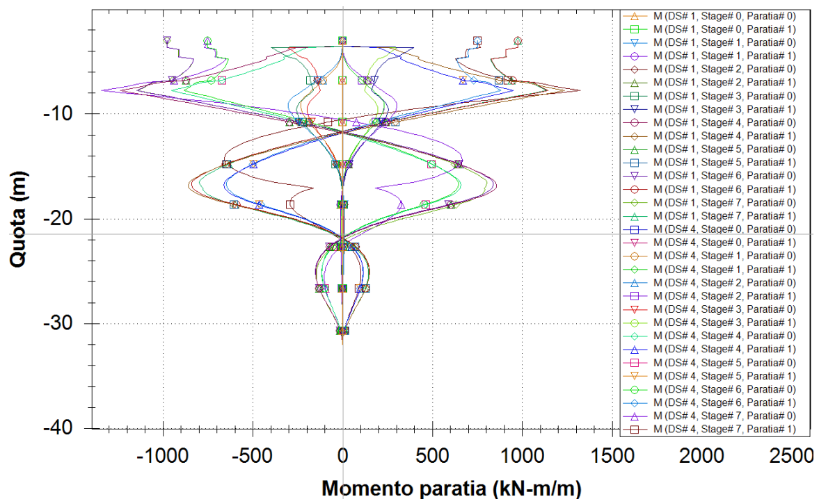
Figura 20 – A1-M1-R1(Statica "DS#1" e Sismica "DS#4") – Momento Flettente
