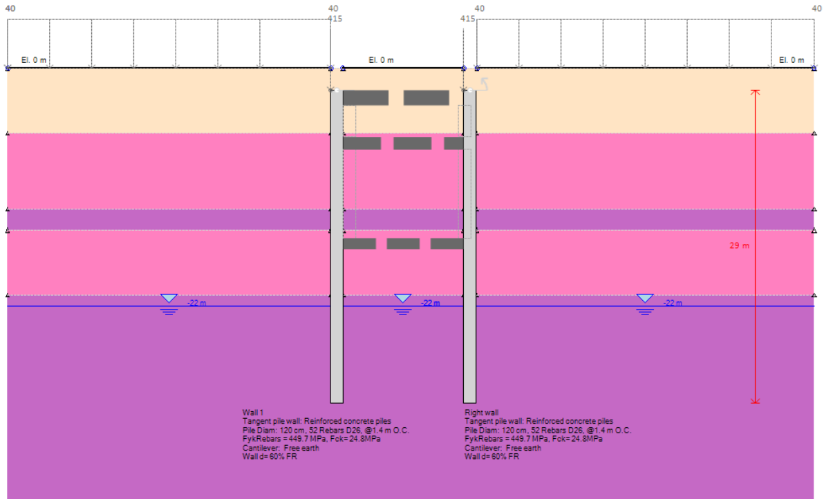
Figura 24 – Esecuzione pali \phi=1200 mm ed inizializzazione geostatica (step 0)
