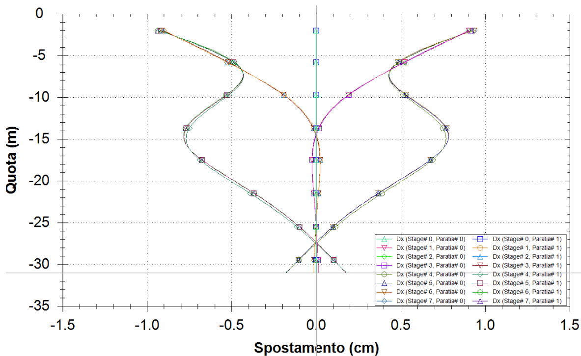
Figura 35 – SLE - Deformazioni Fase per Fase
