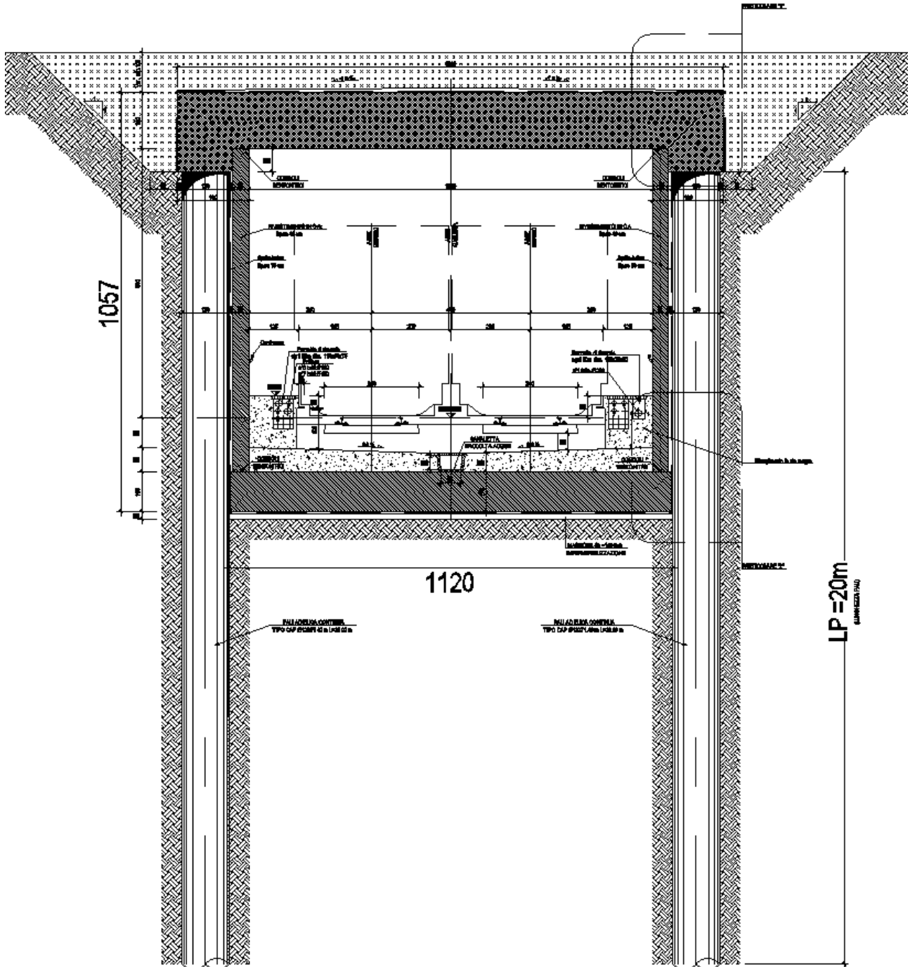
Figura 1 – Sezione tipo A
