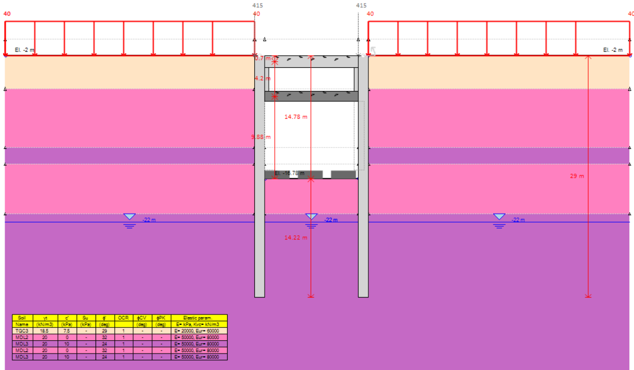
Figura 28 – Esecuzione scavo a foro cieco fino ad intradosso solettone di base (step 4)
