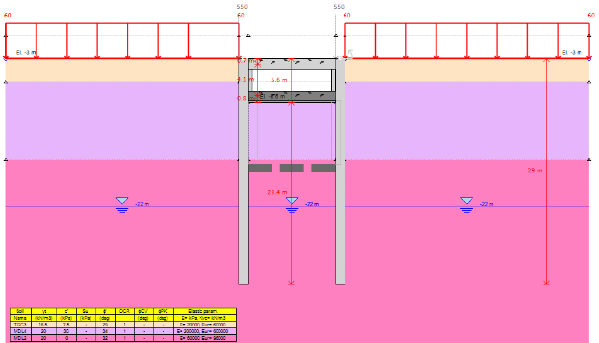
Figura 15 – Realizzazione solettone di copertura e pareti di rivestimento camera superiore (step 2)
