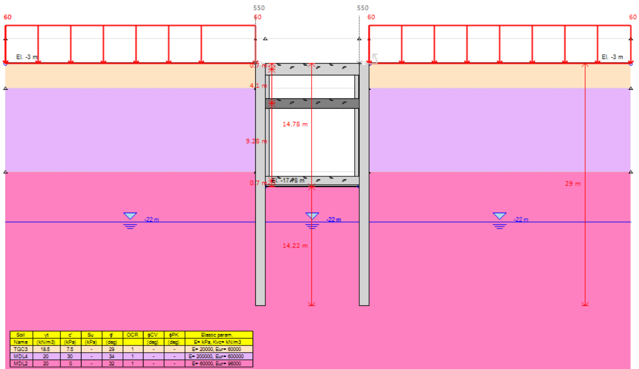
Figura 17 – Realizzazione solettone di base e pareti di rivestimento camera inferiore (step 4)
