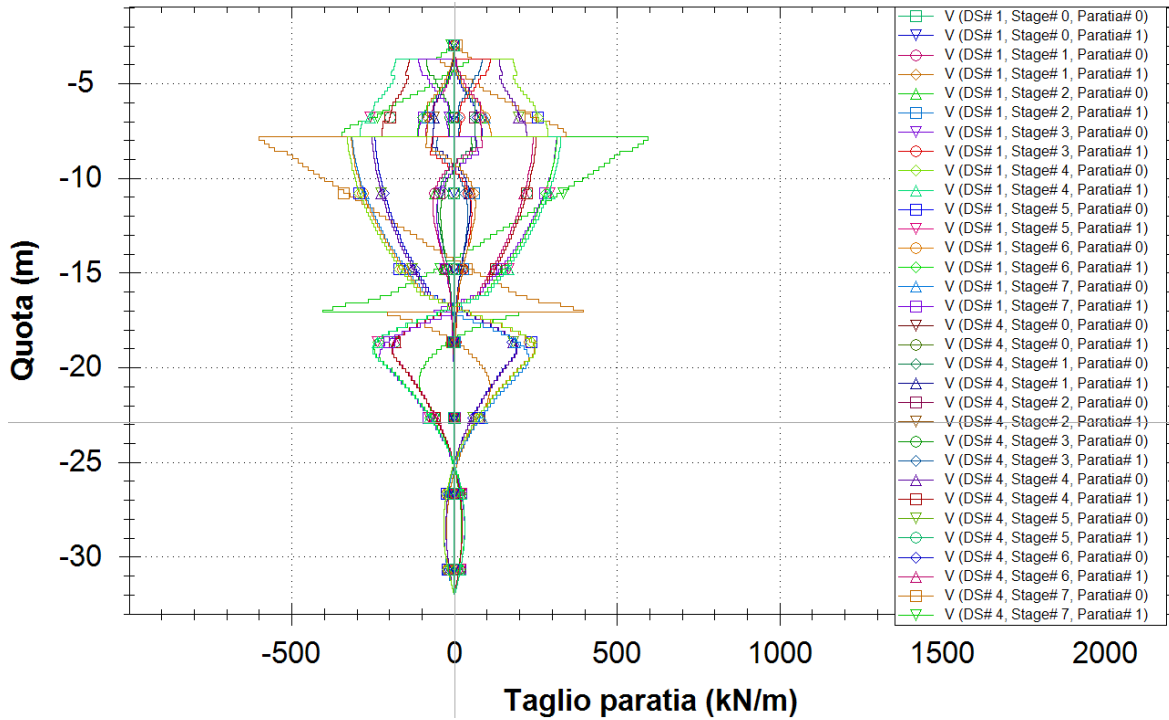
Figura 21 – A1-M1-R1(Statica "DS#1" e Sismica "DS#4") – Taglio
