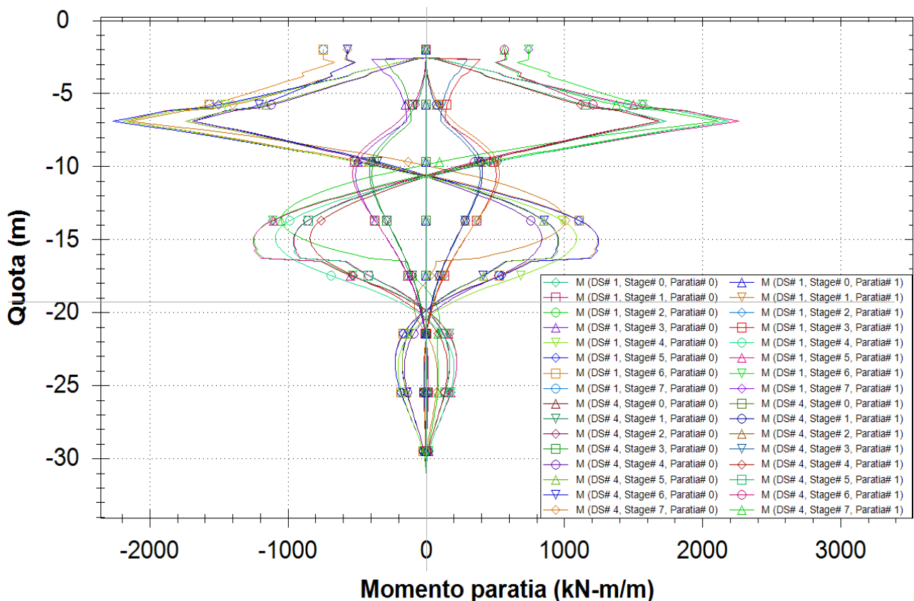
Figura 32 – A1-M1-R1(Statica "DS#1" e Sismica "DS#4") – Momento Flettente
