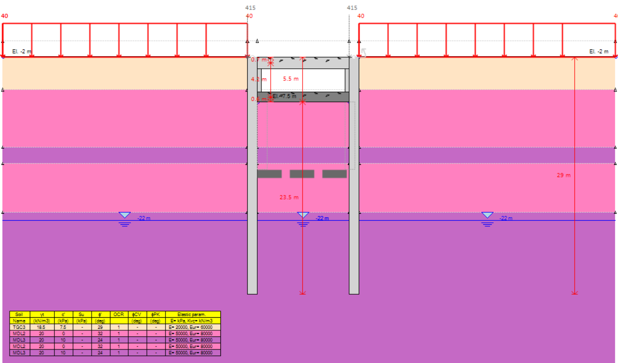
Figura 27 – Realizzazione solettone di copertura e pareti di rivestimento camera superiore (step 3)
