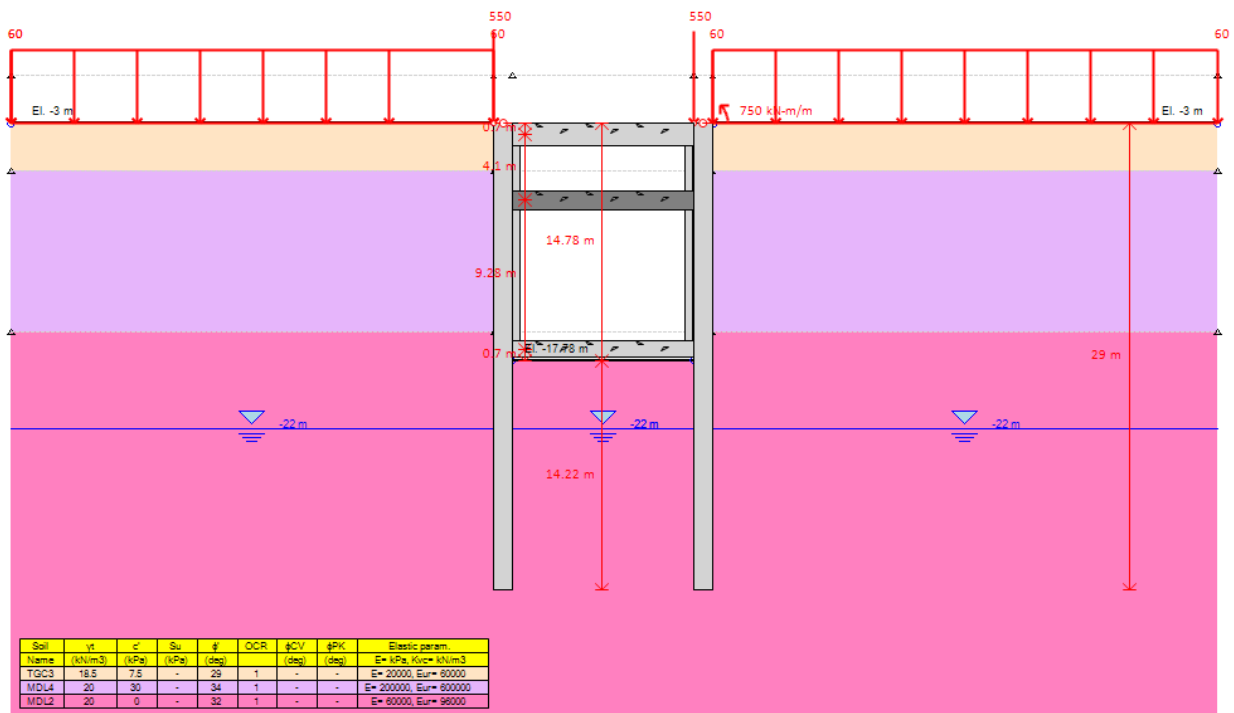
Figura 19 – Attivazione sisma (step 6)
