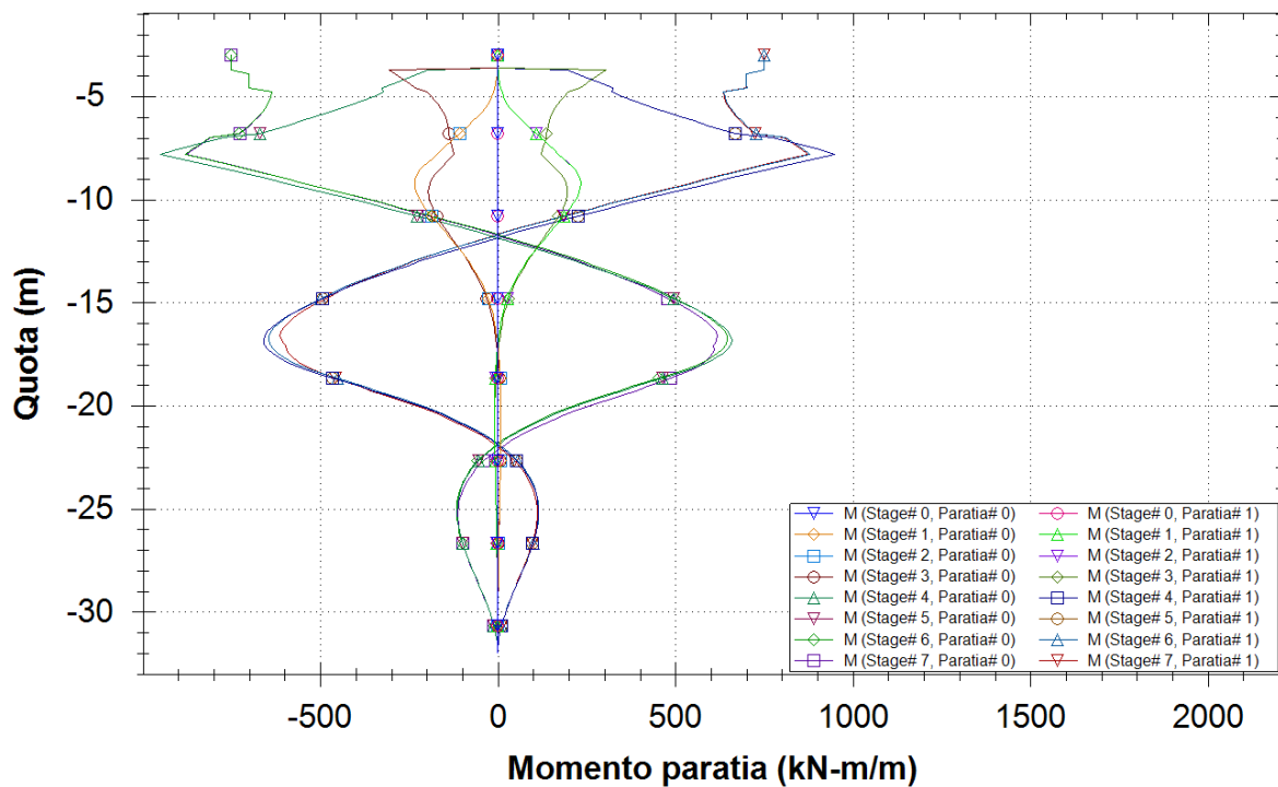
Figura 22 – SLE – Momento Flettente
