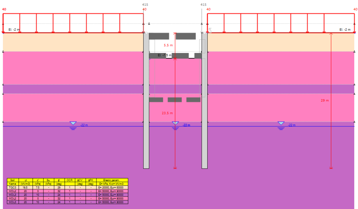
Figura 25 – Esecuzione scavo iniziale fino ad intradosso solettone intermedio(step 1)
