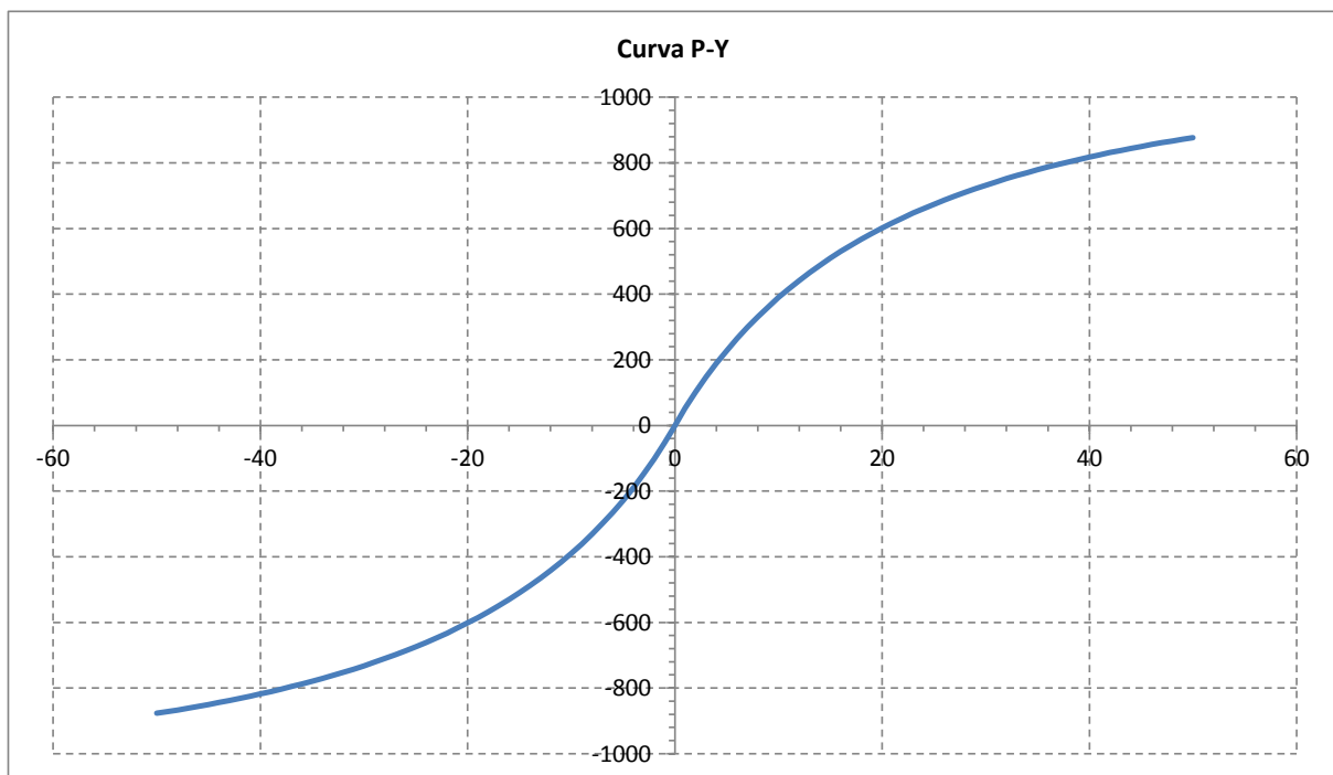
Figura 15 – curva P-Y a quota 10 m da testa palo
