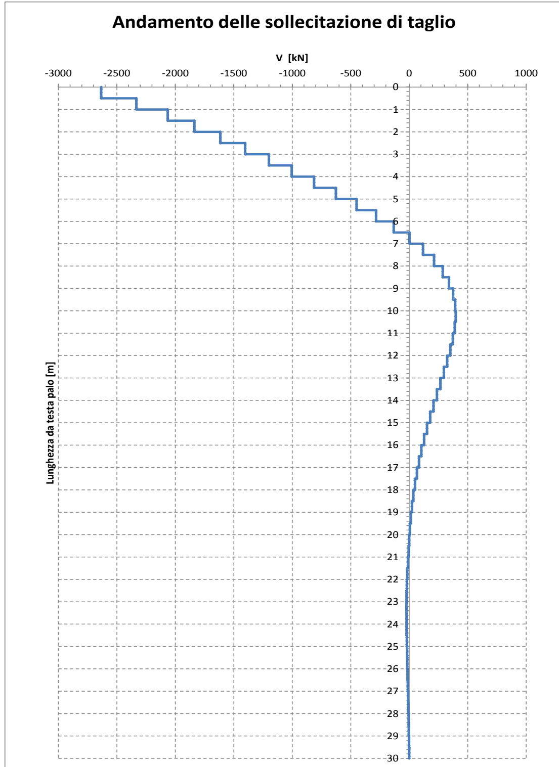
Figura 17 – Andamento taglio
