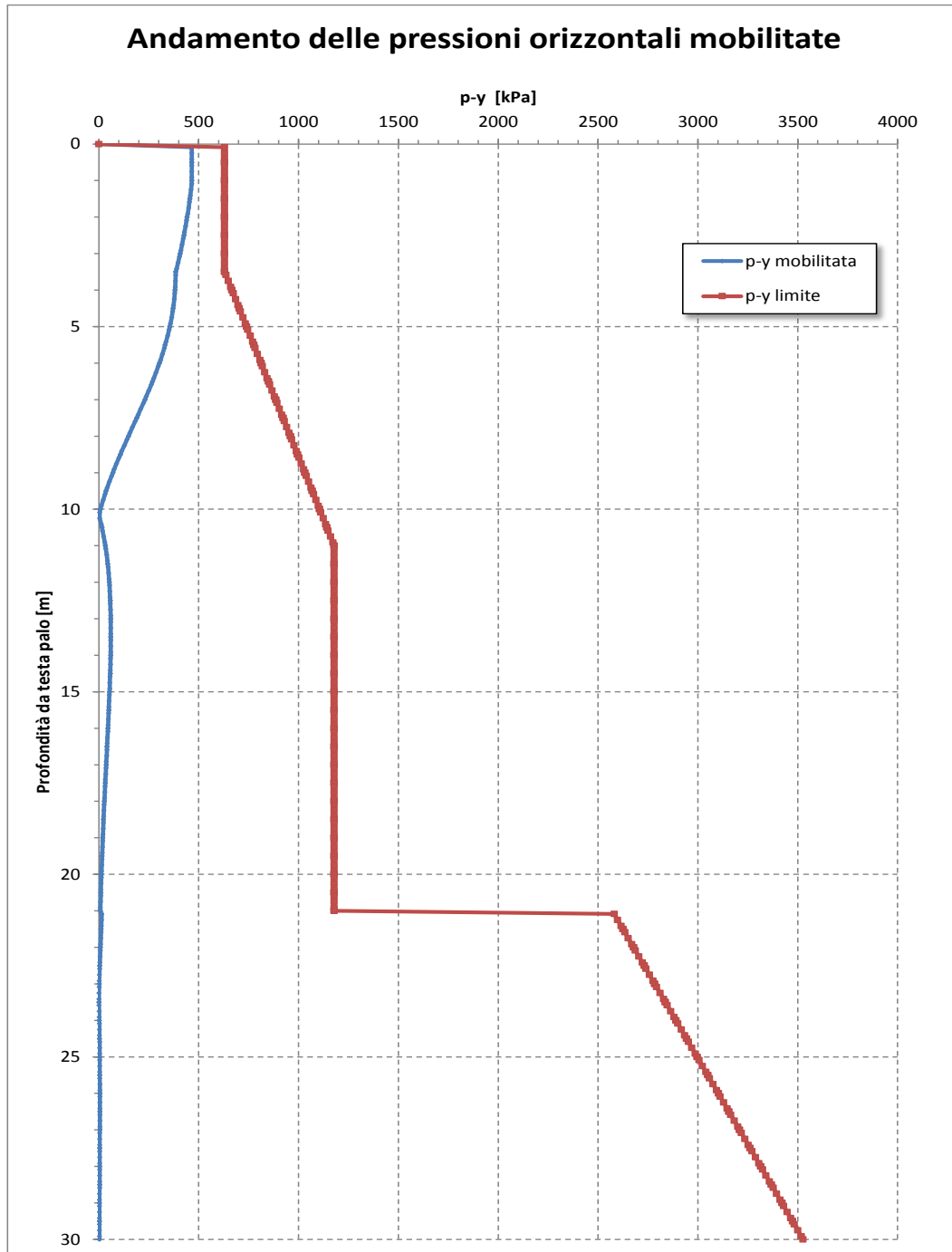
Figura 16 – Andamento pressioni orizzontali
