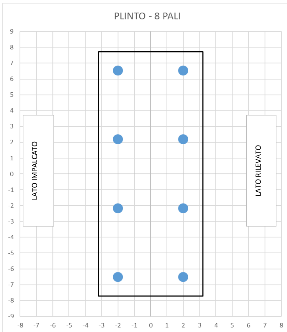
Figura 12 – Geometria Palificata
