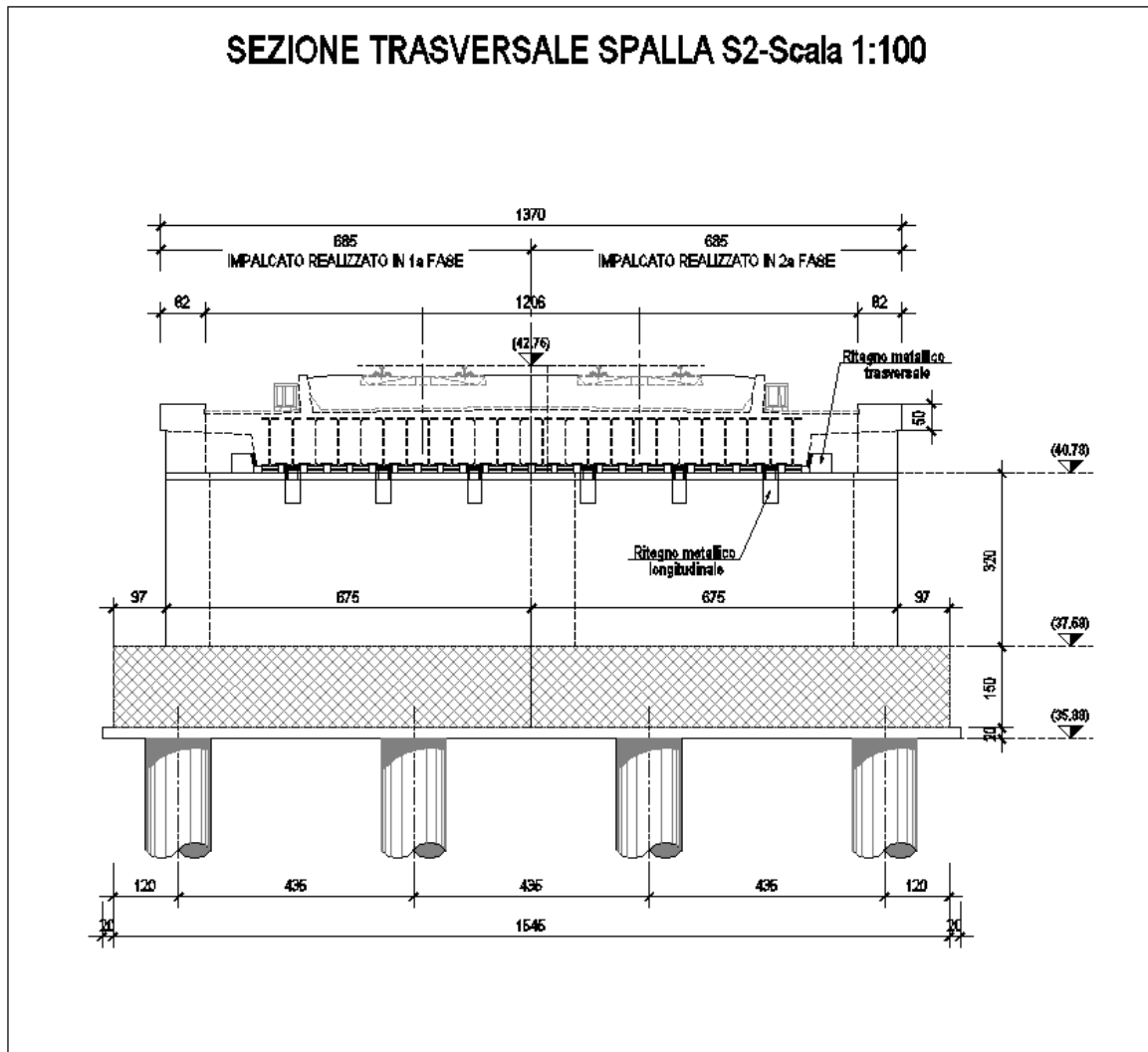
Figura 2 – Spalla S2
