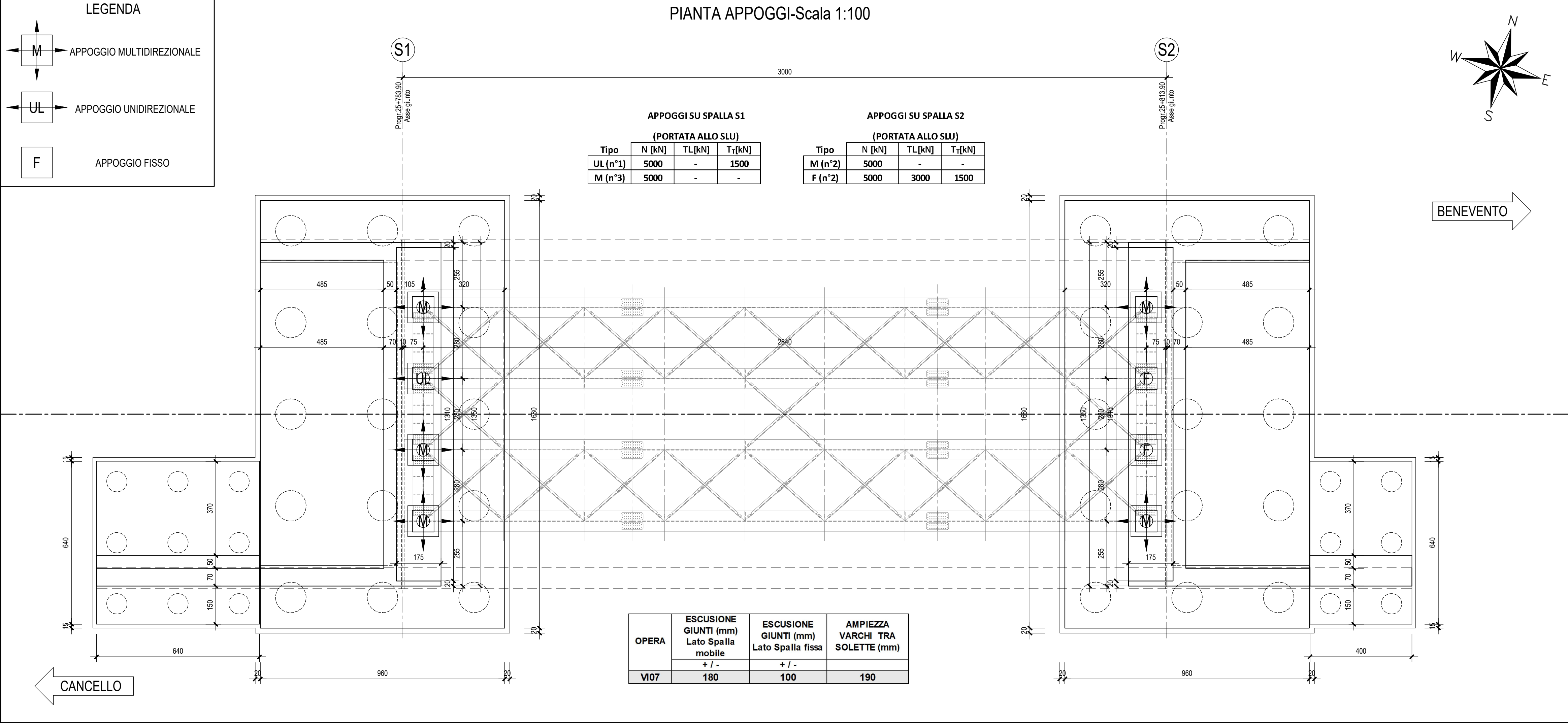
PIANTA APOGGI-Scala 1:100
