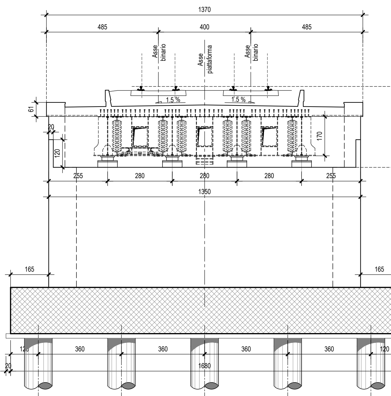
SEZIONE TRASVERSALE SPALLA-Scala 1:100
