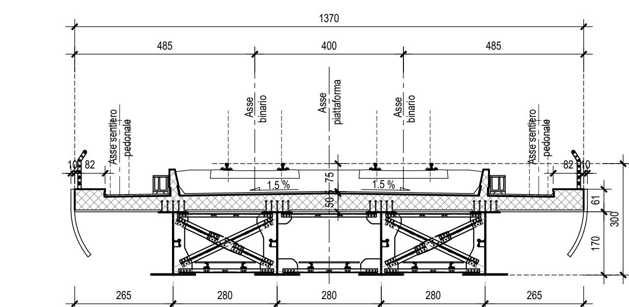
SEZIONE TRASVERSALE SPALLA-Scala 1:100
