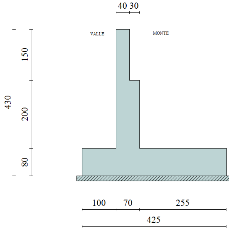
Geometria muro
