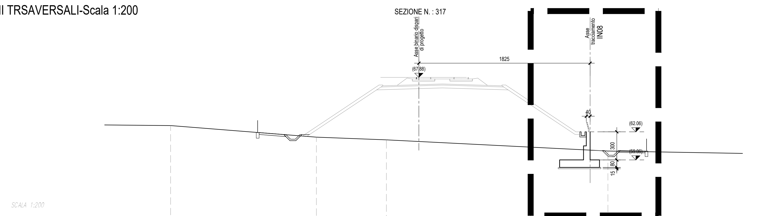
SEZIONI TRSAVERSALI-Scala 1:200
