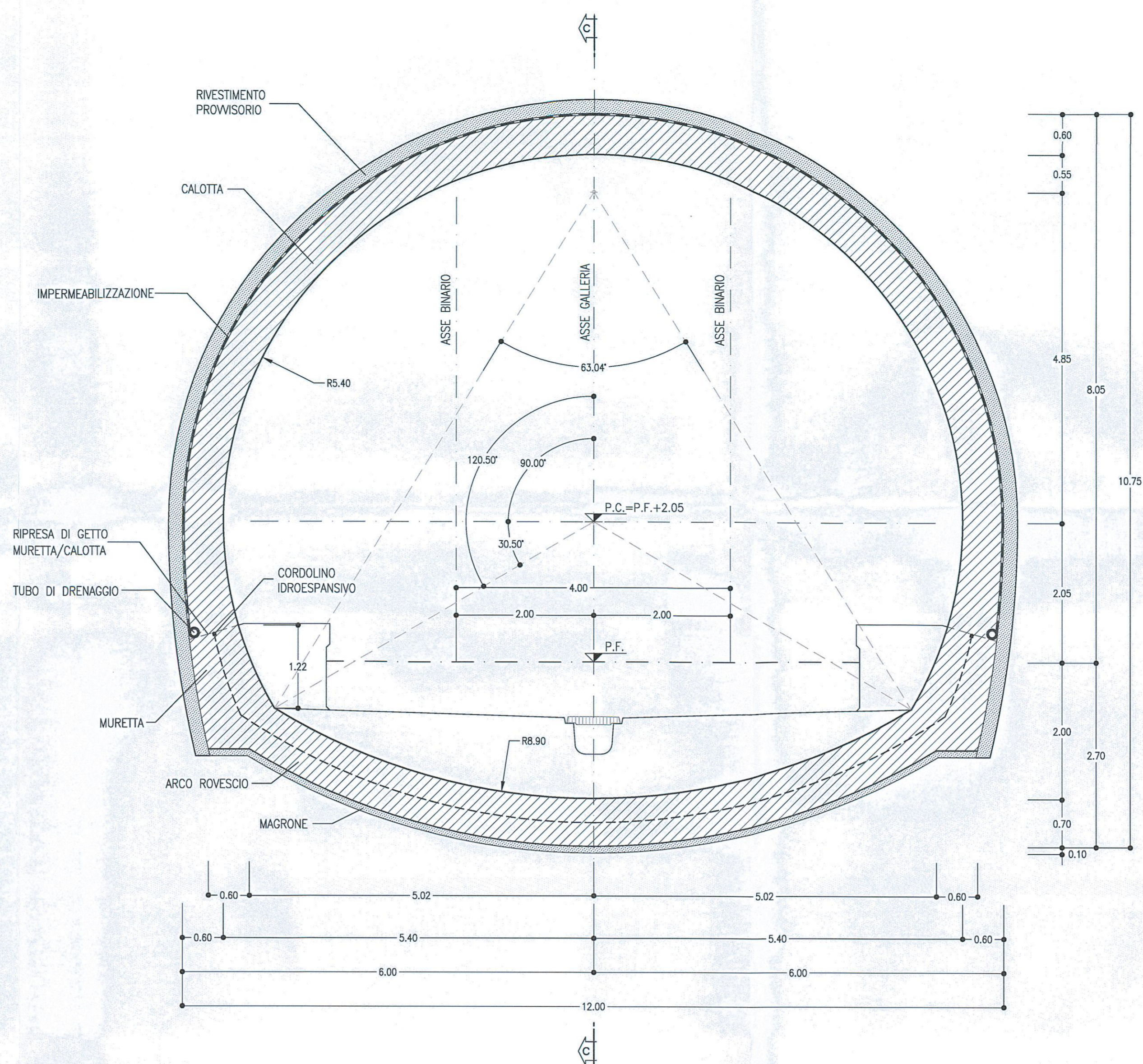
SEZIONE B-B SCALA 1:50 SEZIONE TRASVERSALE CARPENTERIA
