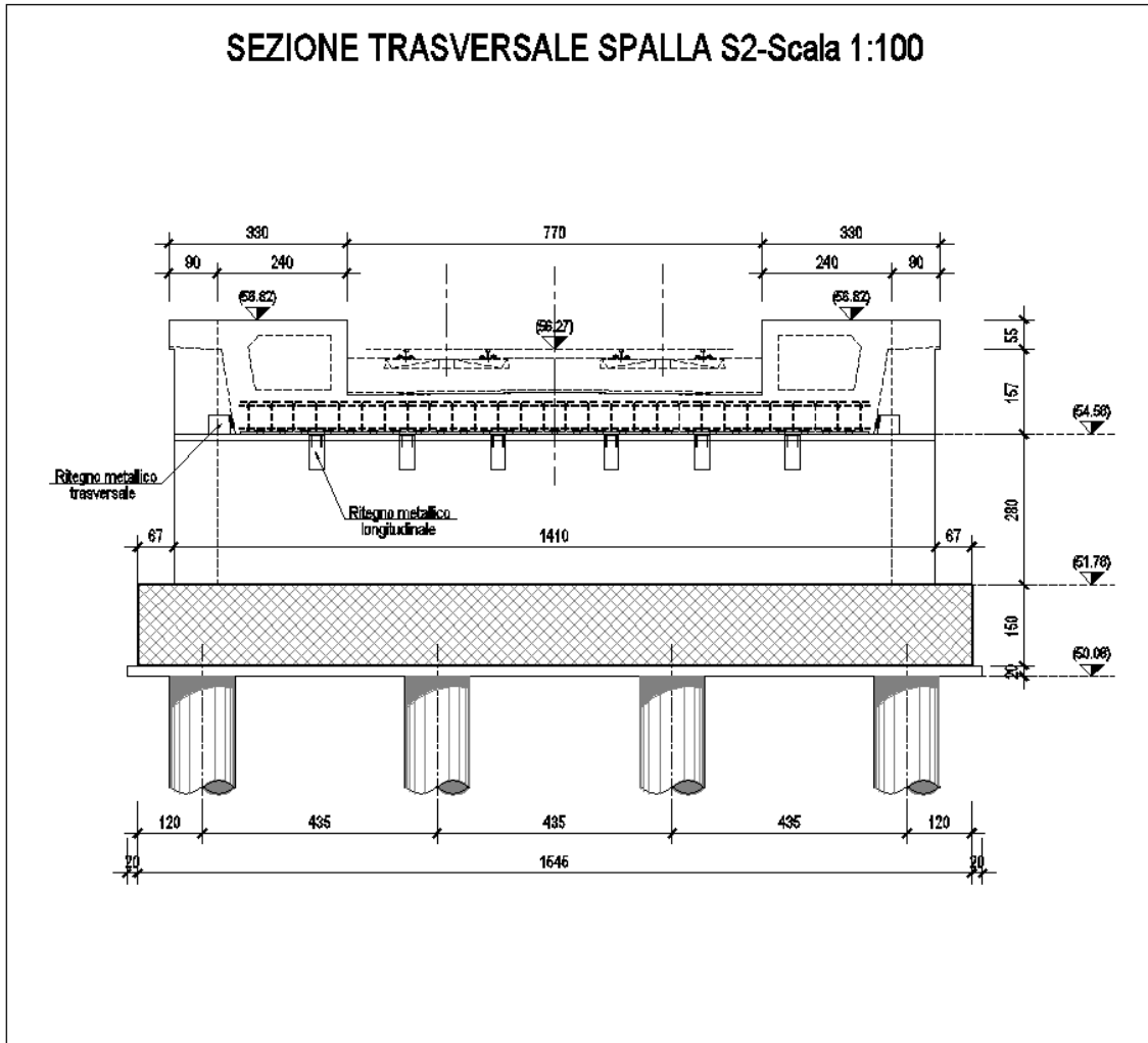
Figura 2 – Spalla S2
