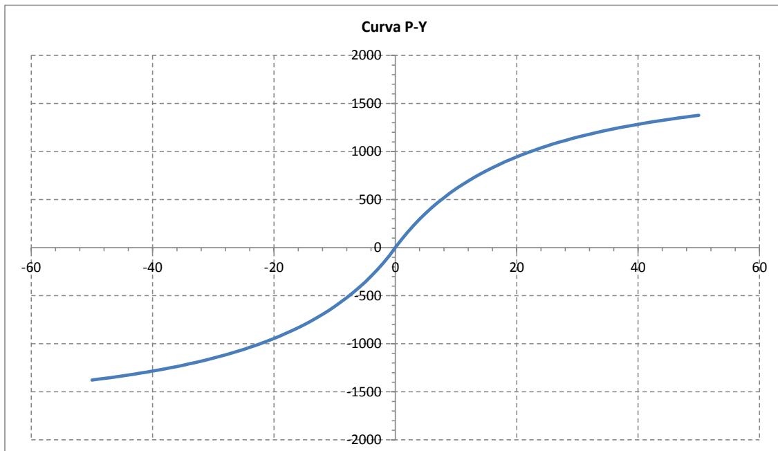
Figura 15 – curva P-Y a quota 10.0 m da testa palo
