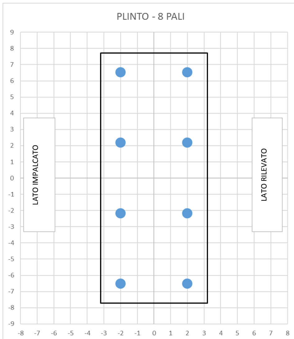
Figura 12 – Geometria Palificata
