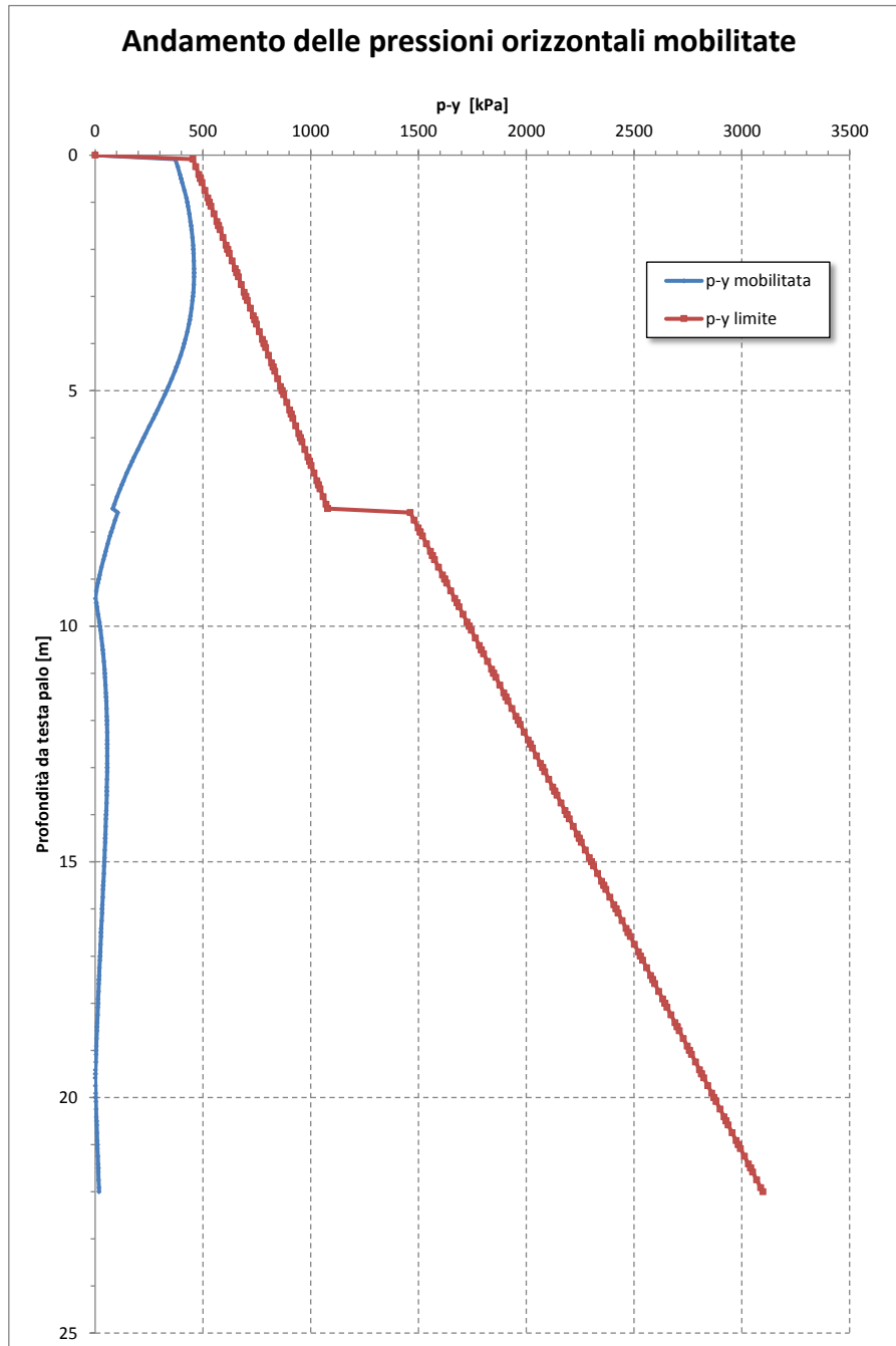
Figura 16 – Andamento pressioni orizzontali
