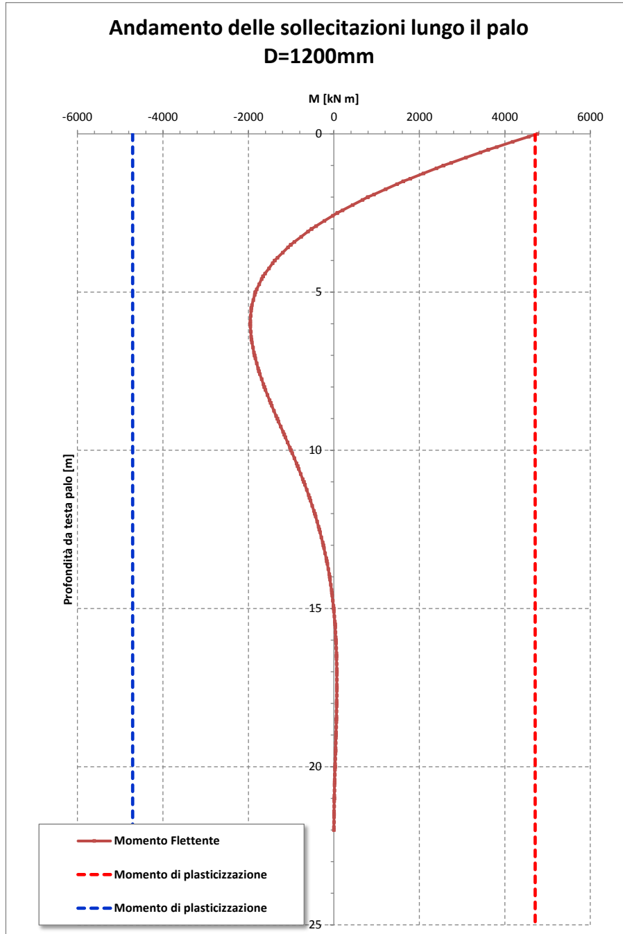
Figura 18 – Andamento momento
