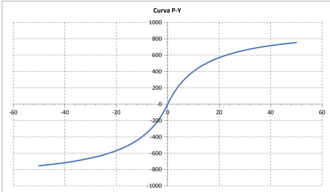
Figura 14 – curva P-Y a quota 5 m da testa palo
