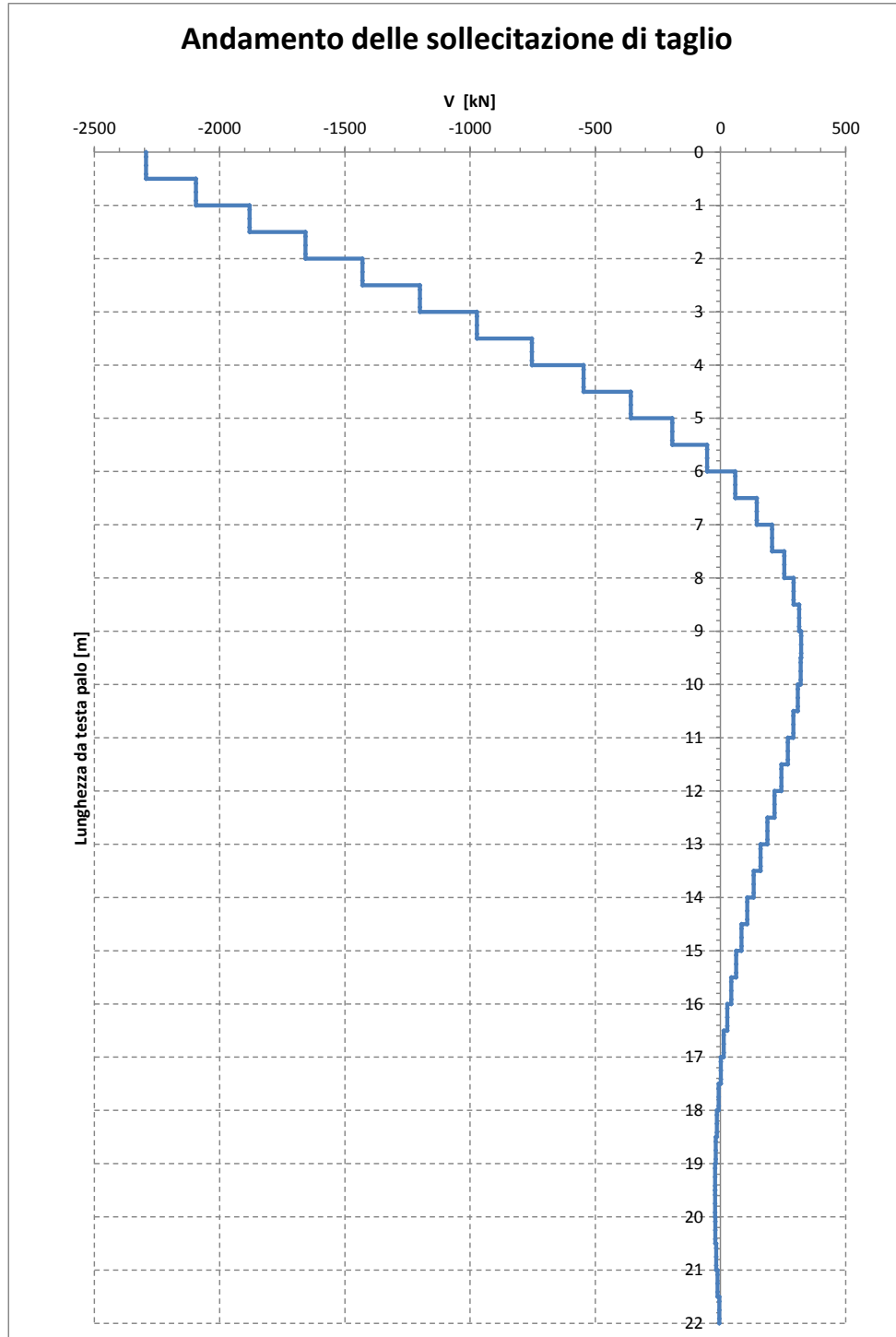
Figura 17 – Andamento taglio
