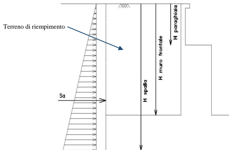
Figura 7: Spinta statica terreno di rinterro
