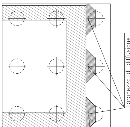
Figura 12 – Diffusione delle azioni dal palo al muro frontale
