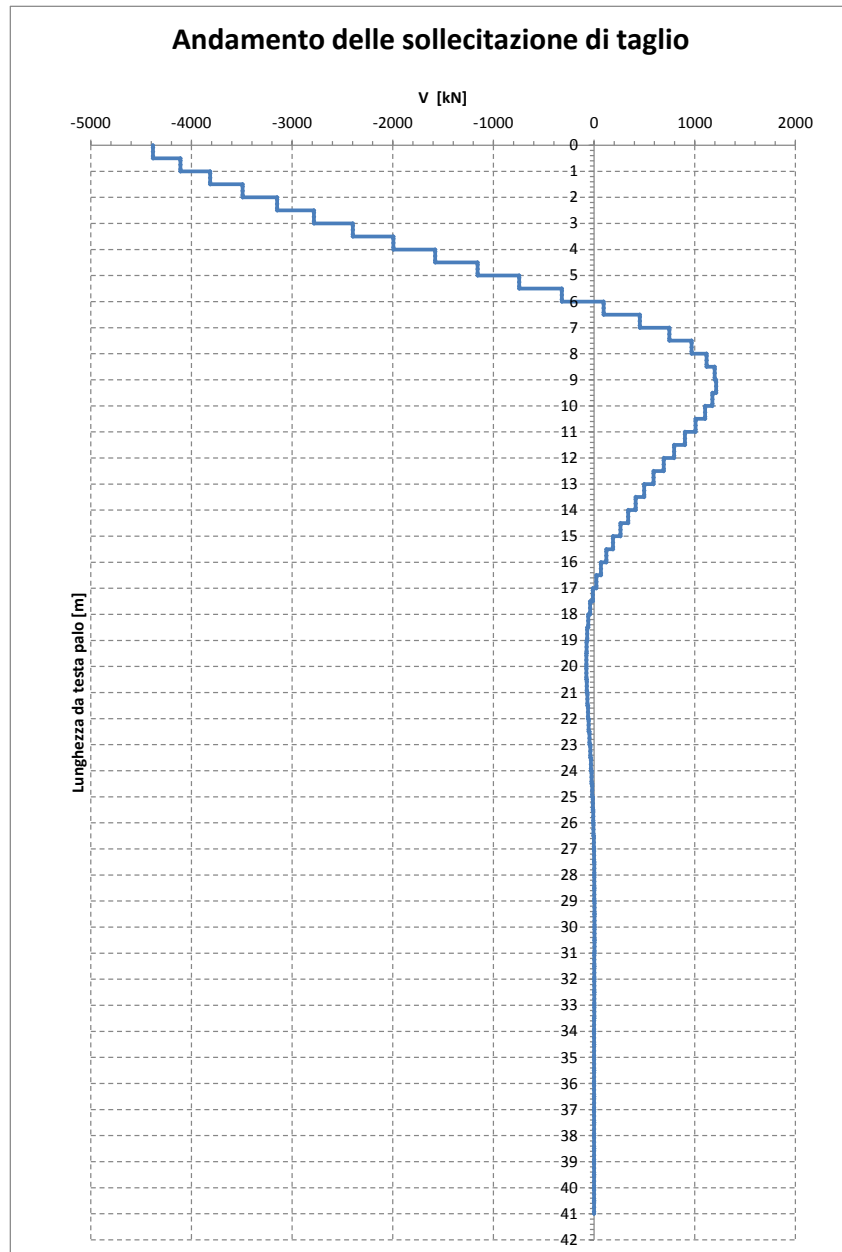
Figura 16 – Andamento taglio
