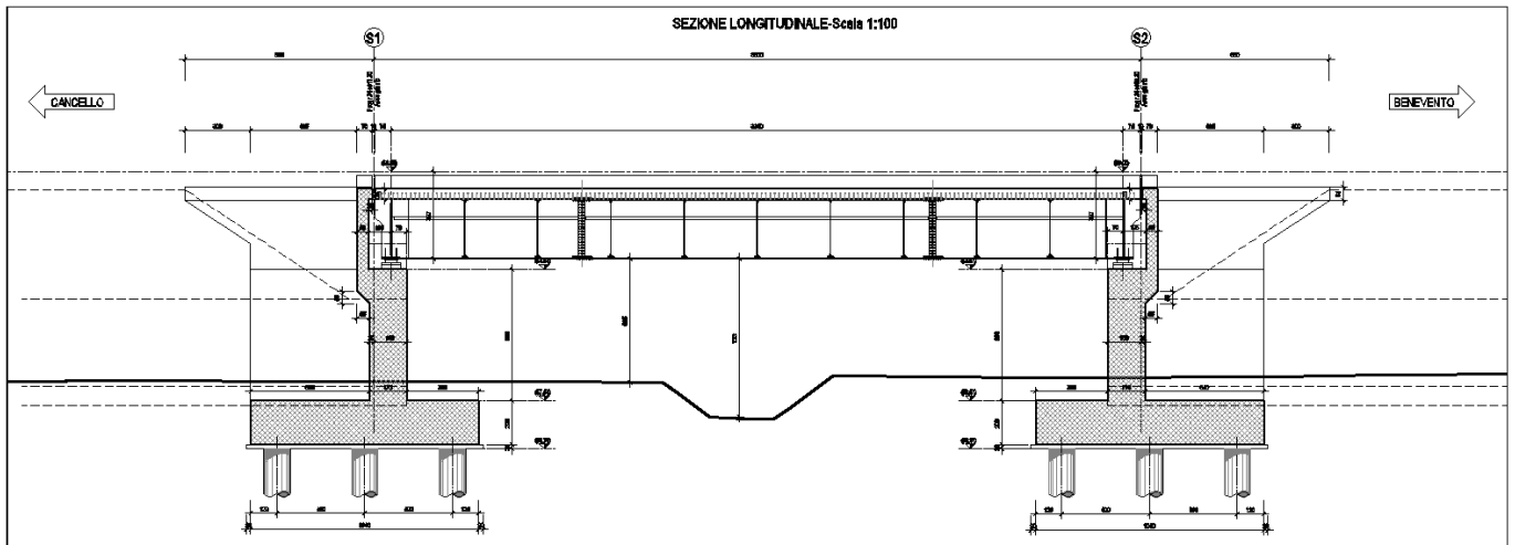
Figura 1 – Sezione Longitudinale Viadotto
