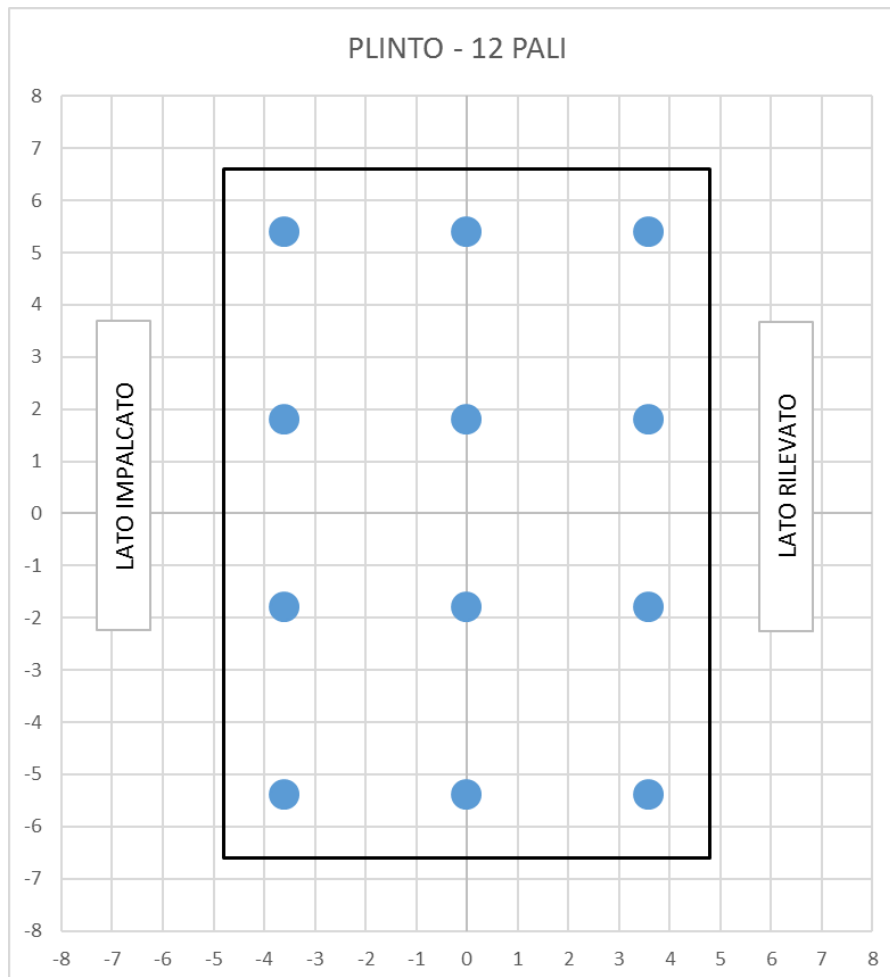
Figura 11 – Geometria Palificata
