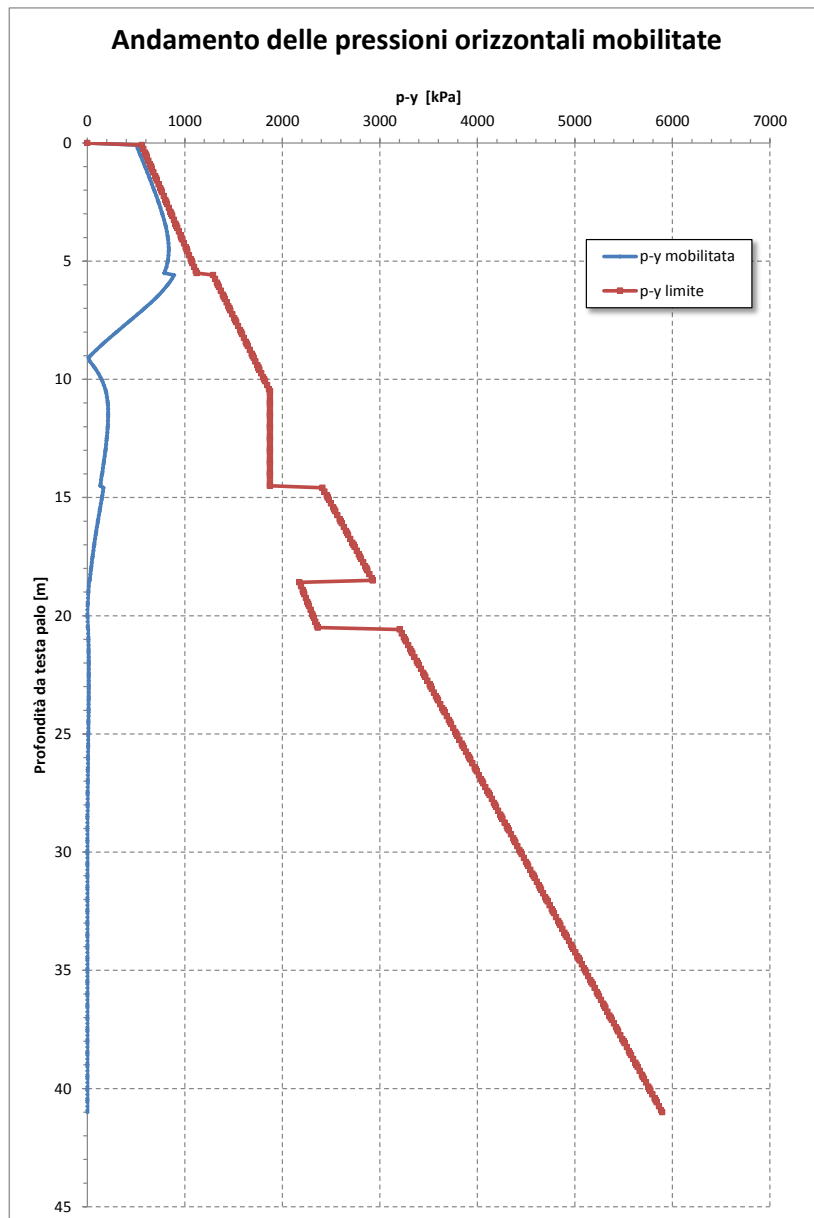
Figura 15 – Andamento pressioni orizzontali
