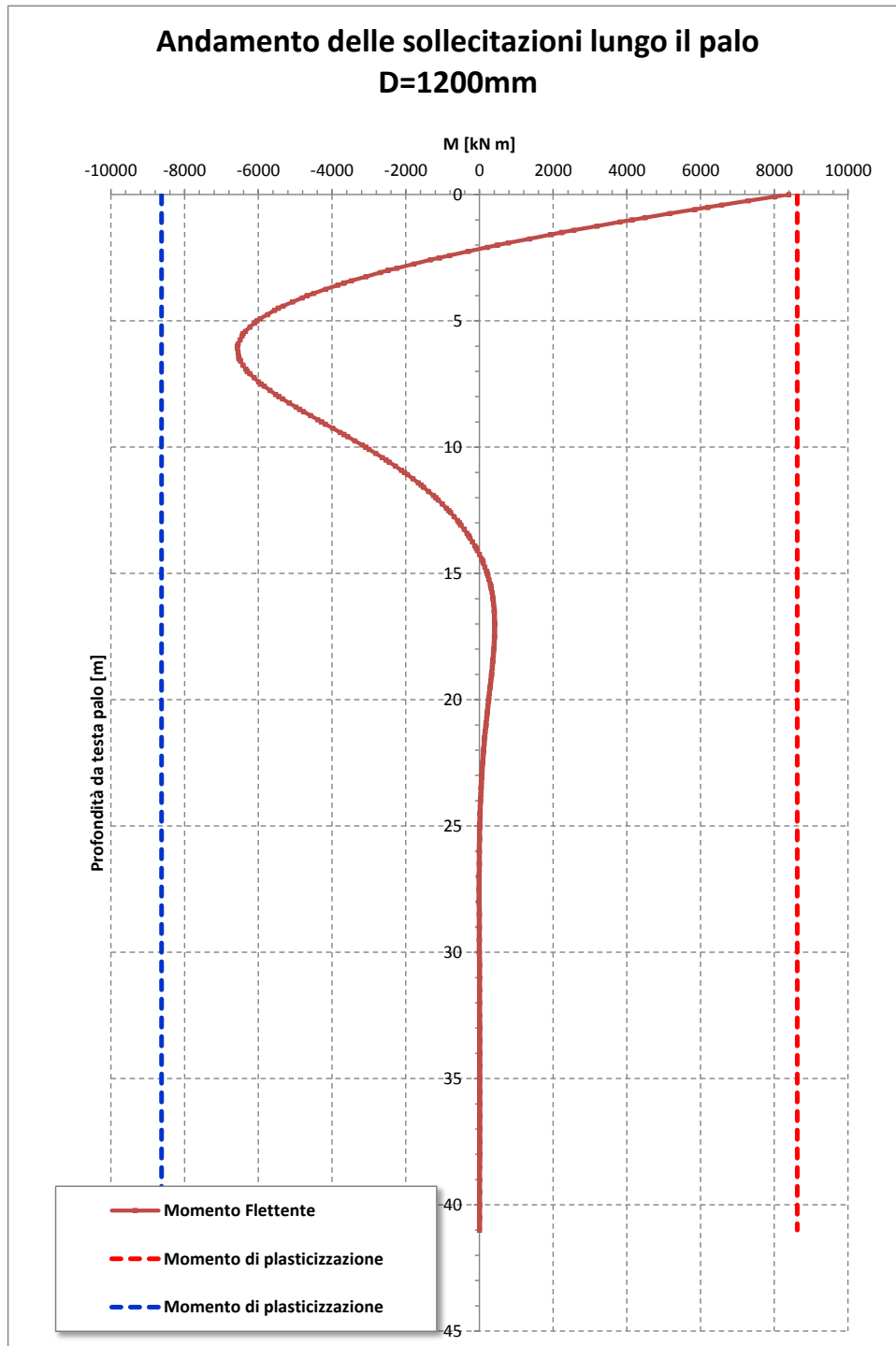
Figura 17 – Andamento momento
