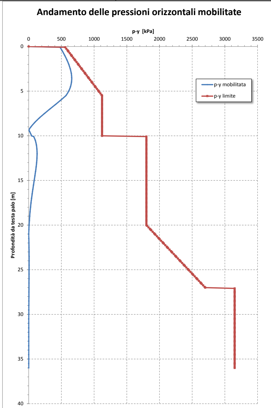
Figura 15 – Andamento pressioni orizzontali
