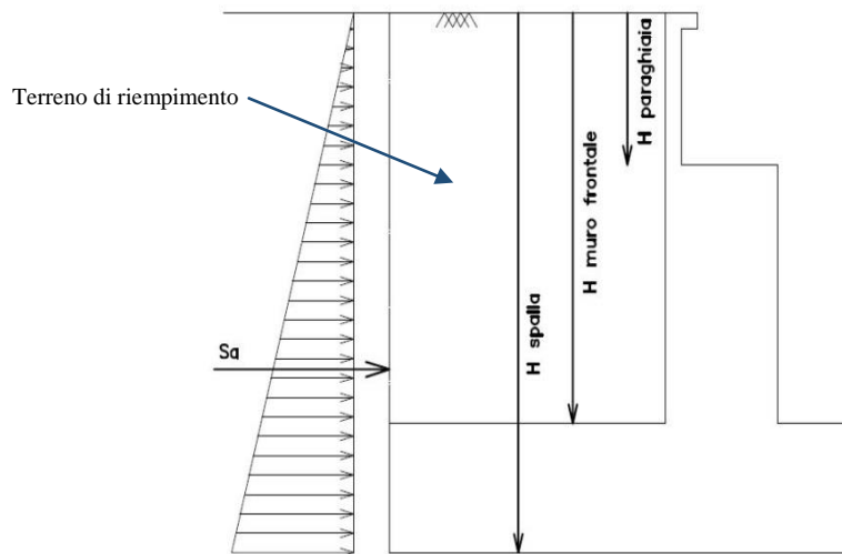
Figura 7: Spinta statica terreno di rinterro
