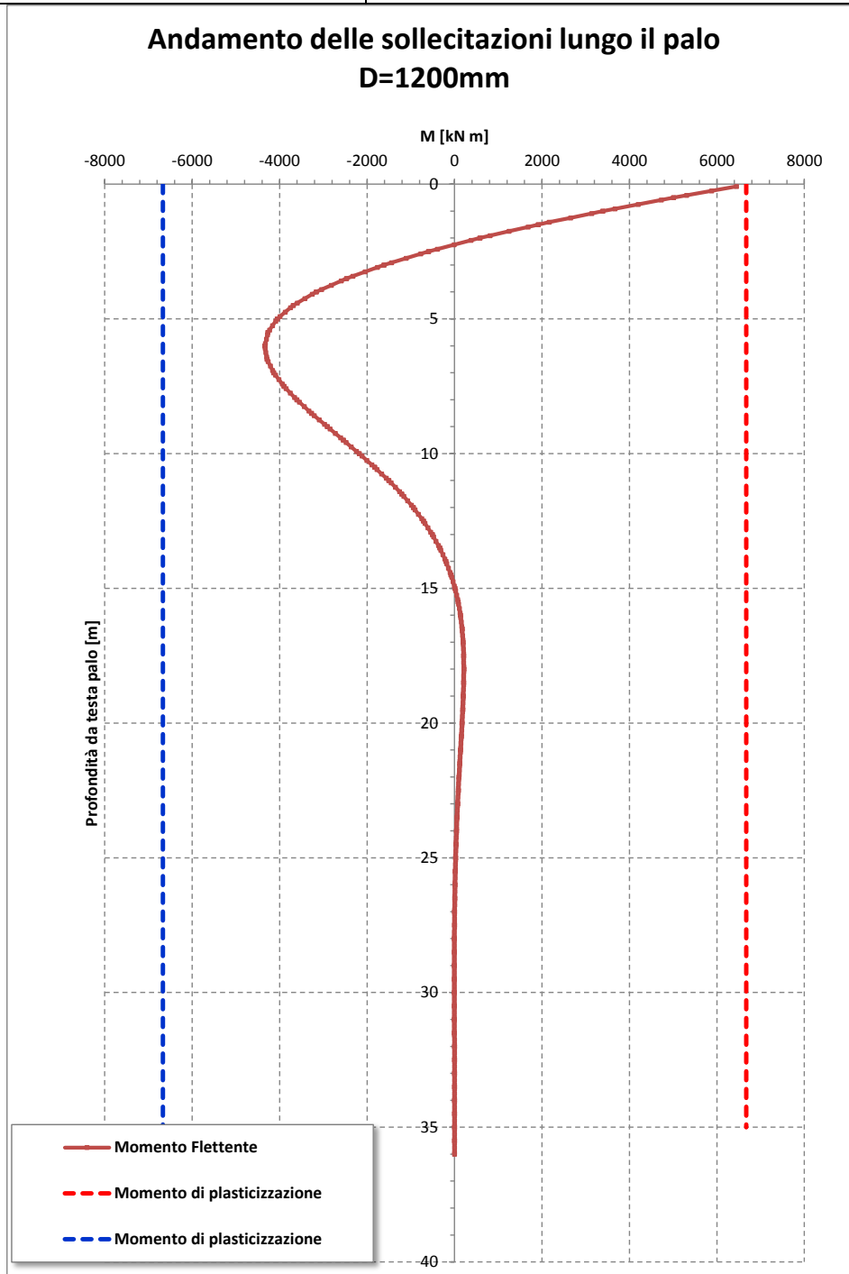
Figura 17 – Andamento momento
