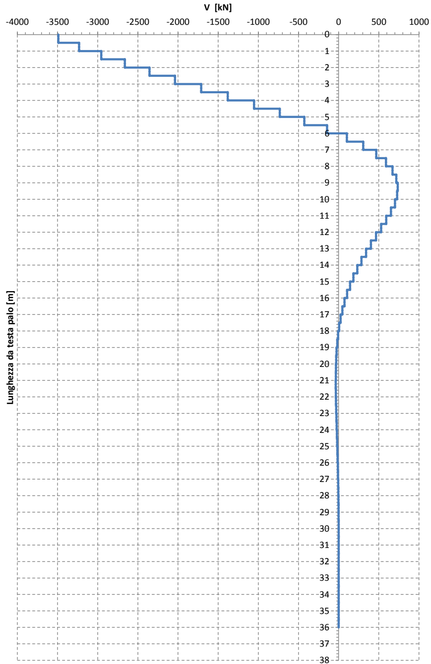
Figura 16 – Andamento taglio
