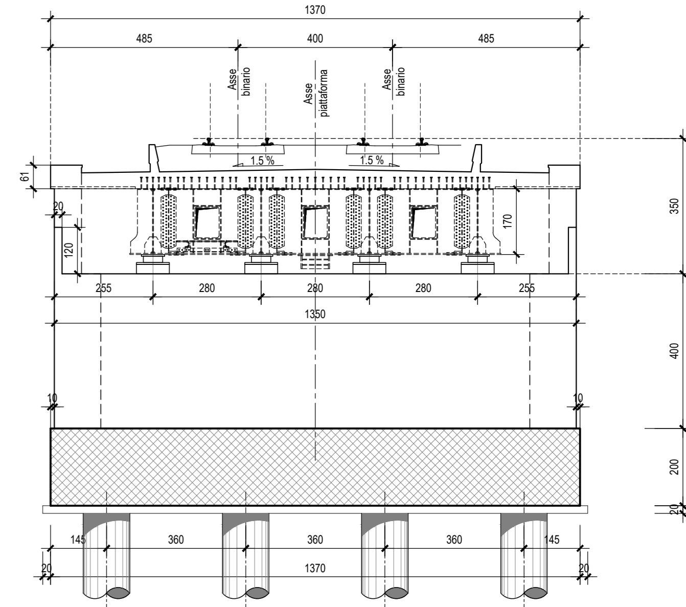
SEZIONE TRASVERSALE SPALLA-Scala 1:100
