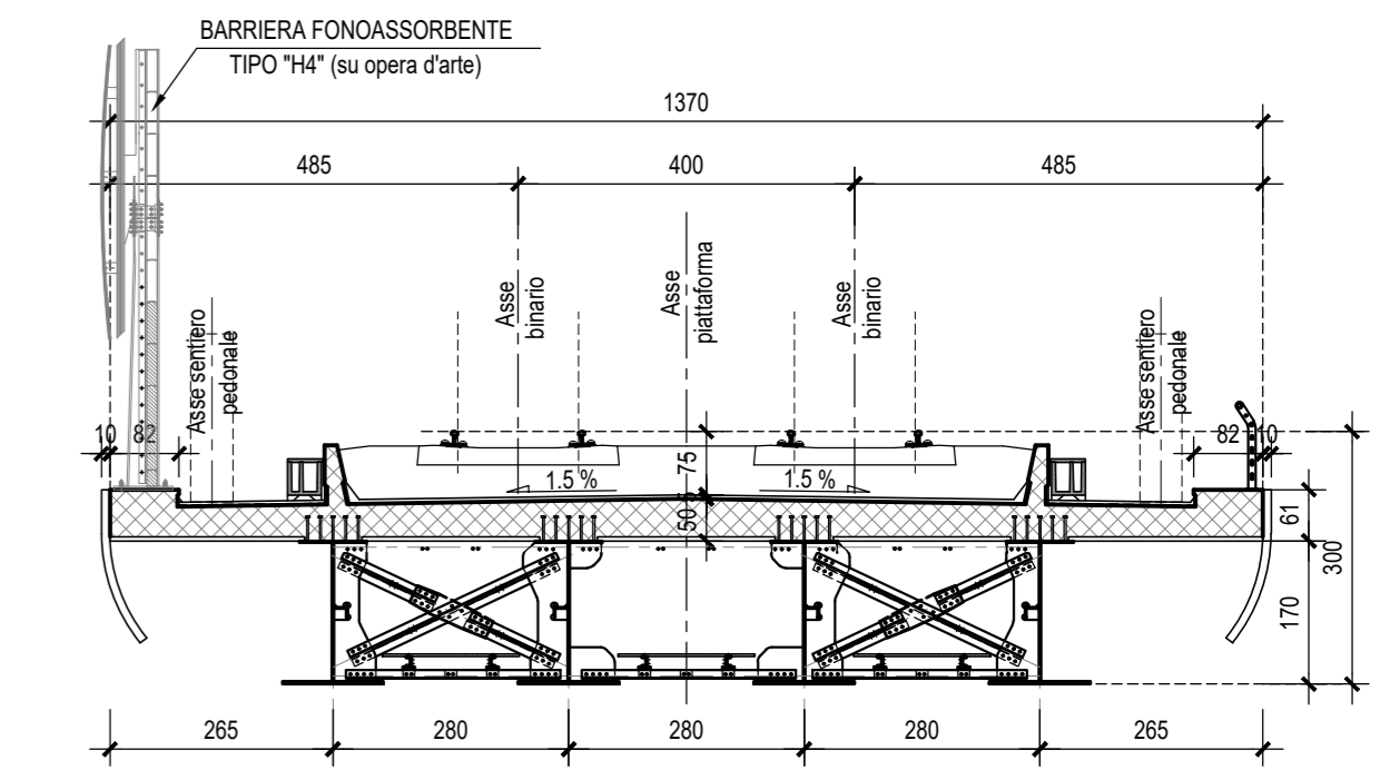
SEZIONE TRASVERSALE CORRENTE-Scala 1:100
