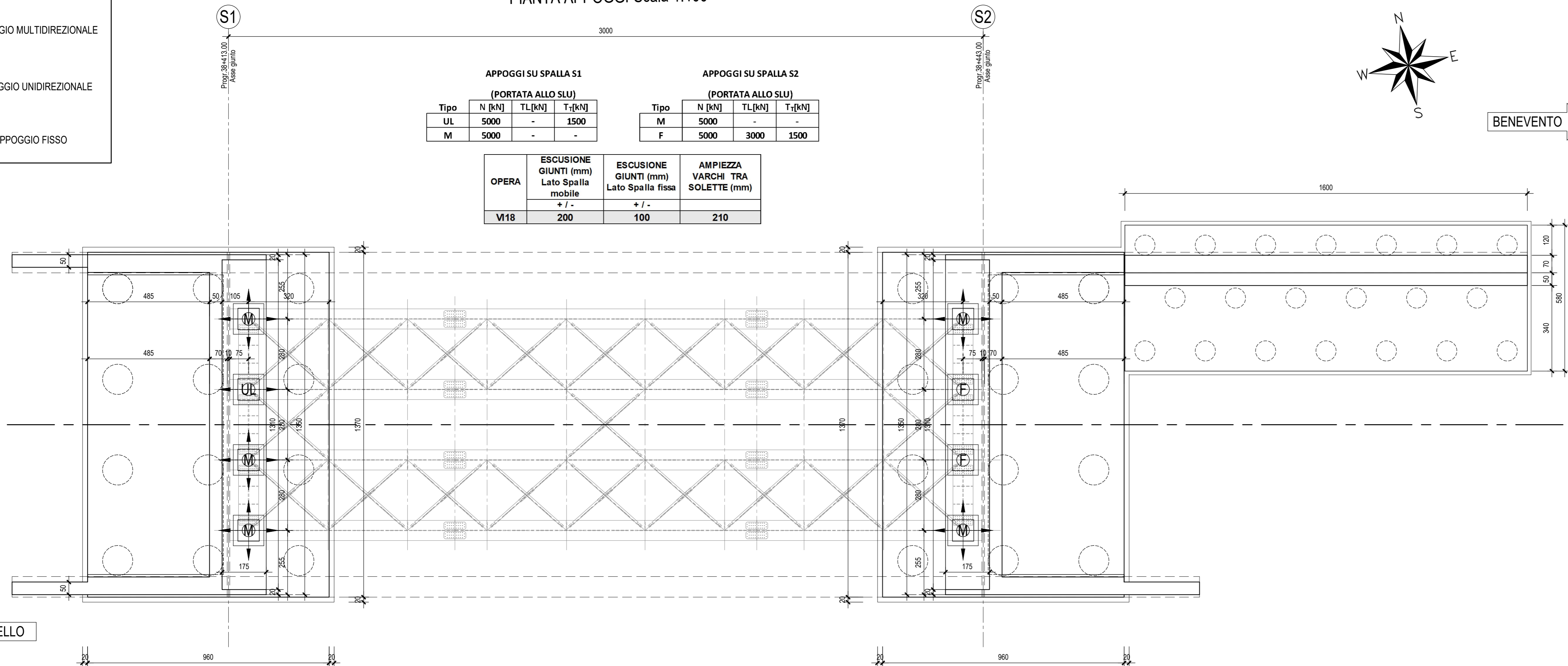
PIANTA APPOGGI-Scala 1:100
