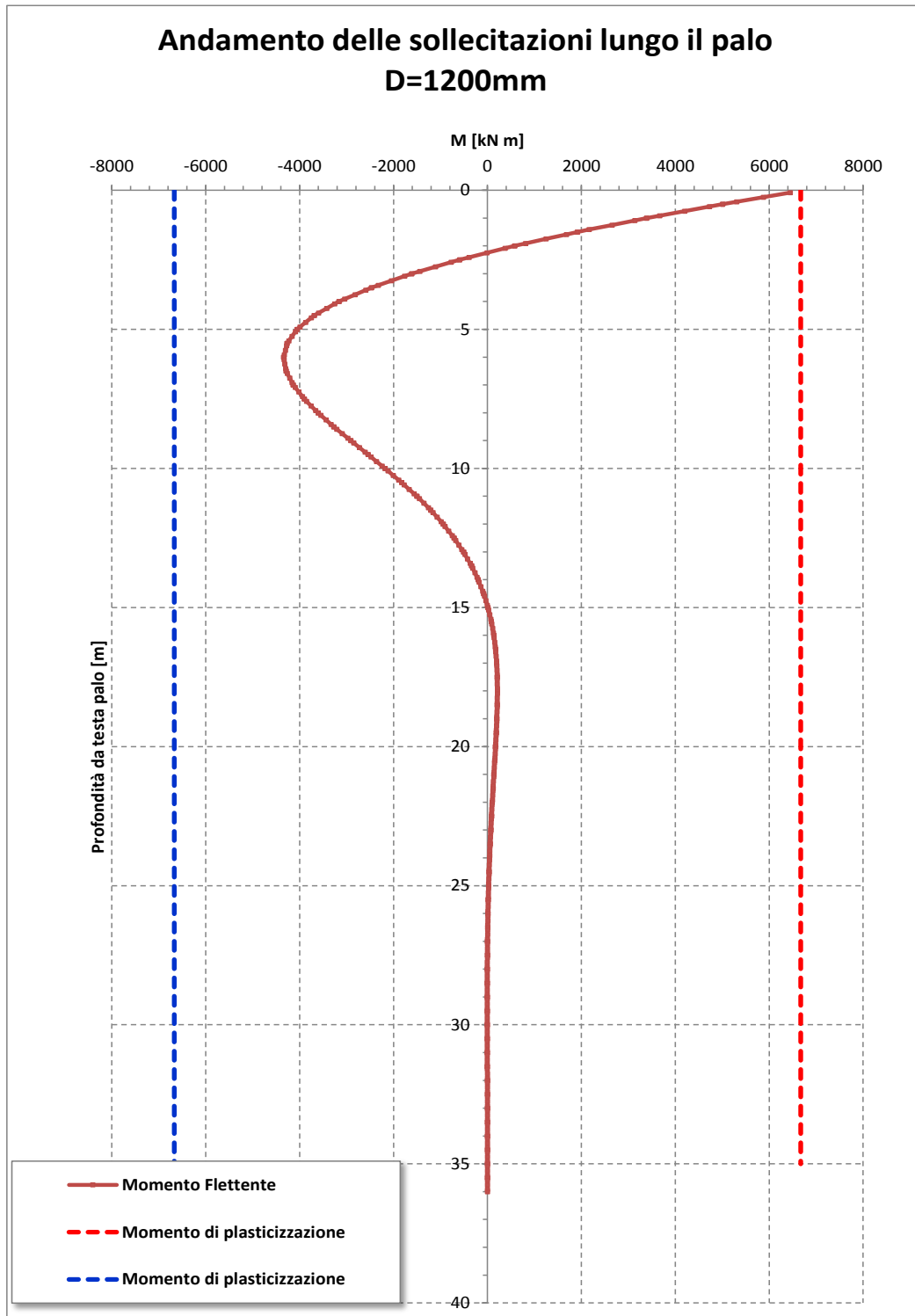
Figura 18 – Andamento momento
