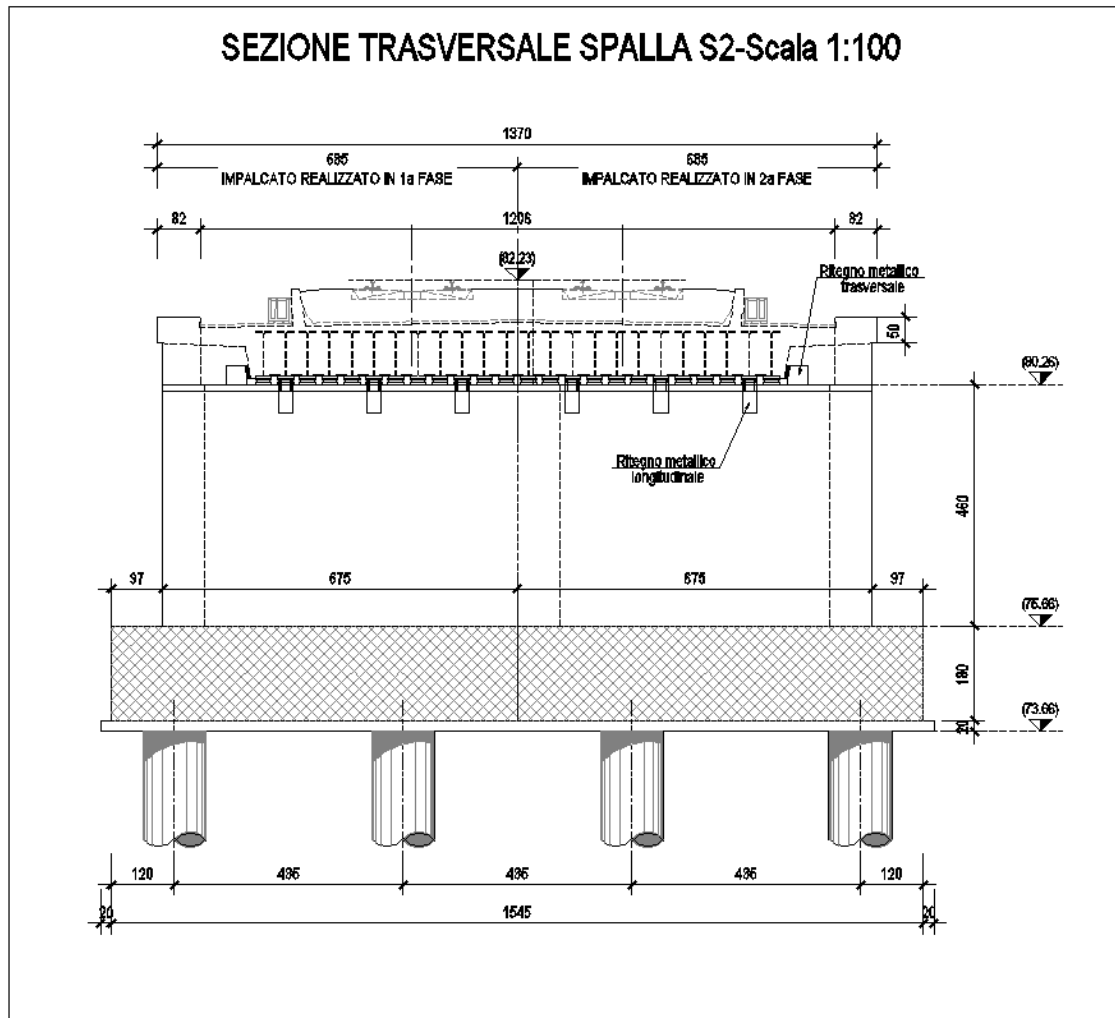
Figura 2 – Spalla S2
