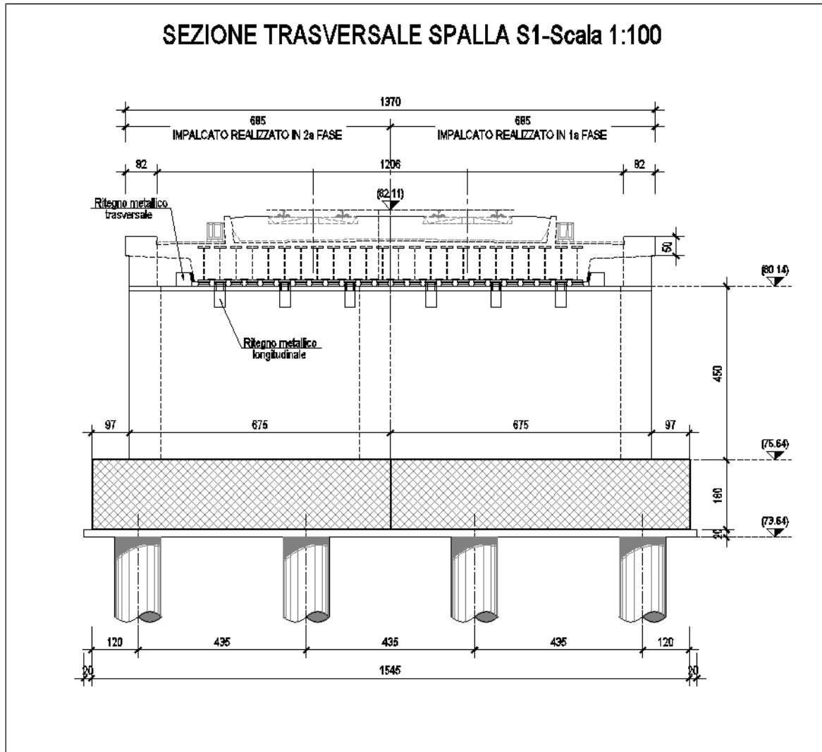
Figura 1 – Spalla S1
