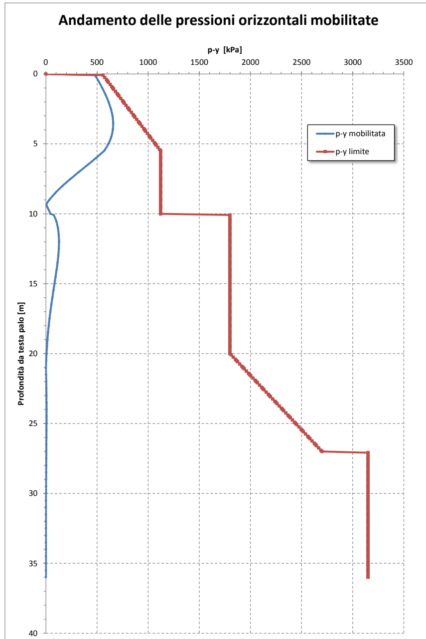
Figura 16 – Andamento pressioni orizzontali
