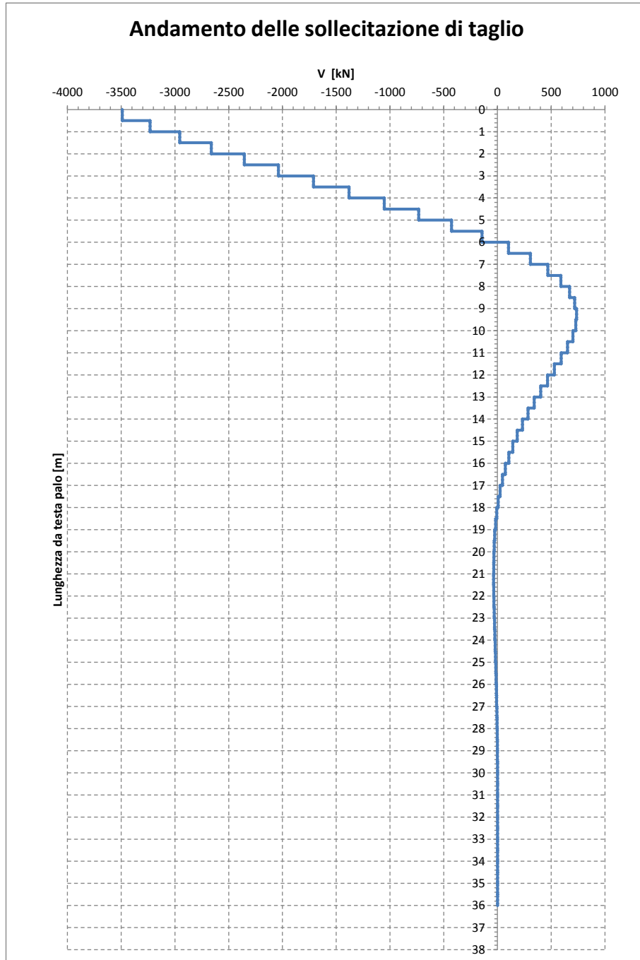
Figura 17 – Andamento taglio
