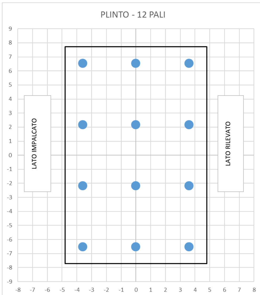
Figura 12 – Geometria Palificata
