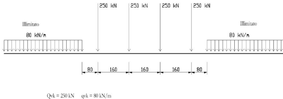
Figura 8 - Treno LM71
