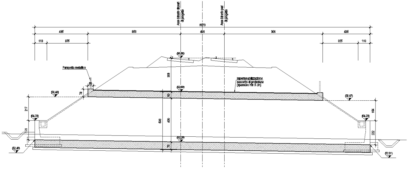
Figura 2 - Sviluppo Longitudinale
