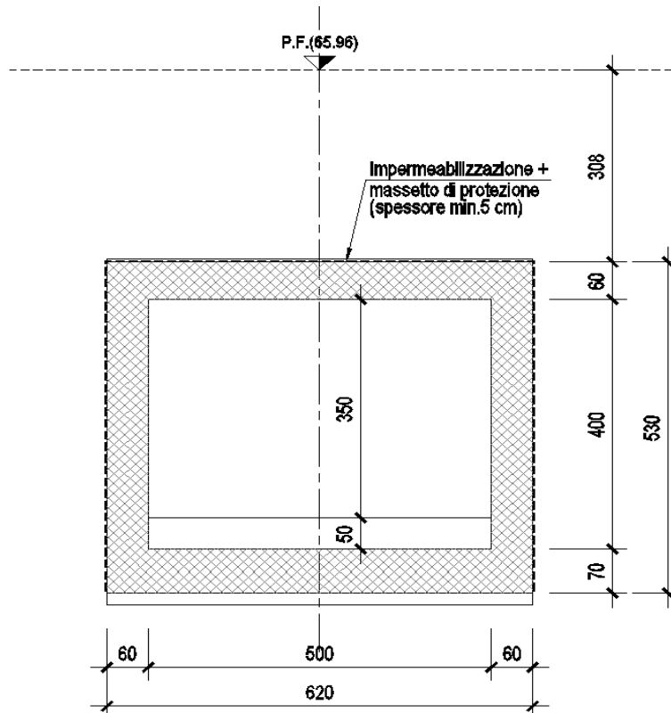
Figura 3 - Sezione trasversale
