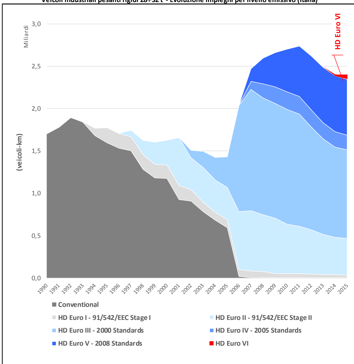
Veicoli industriali pesanti rigidi 28÷32 t - Evoluzione impieghi per livello emissivo (Italia)
