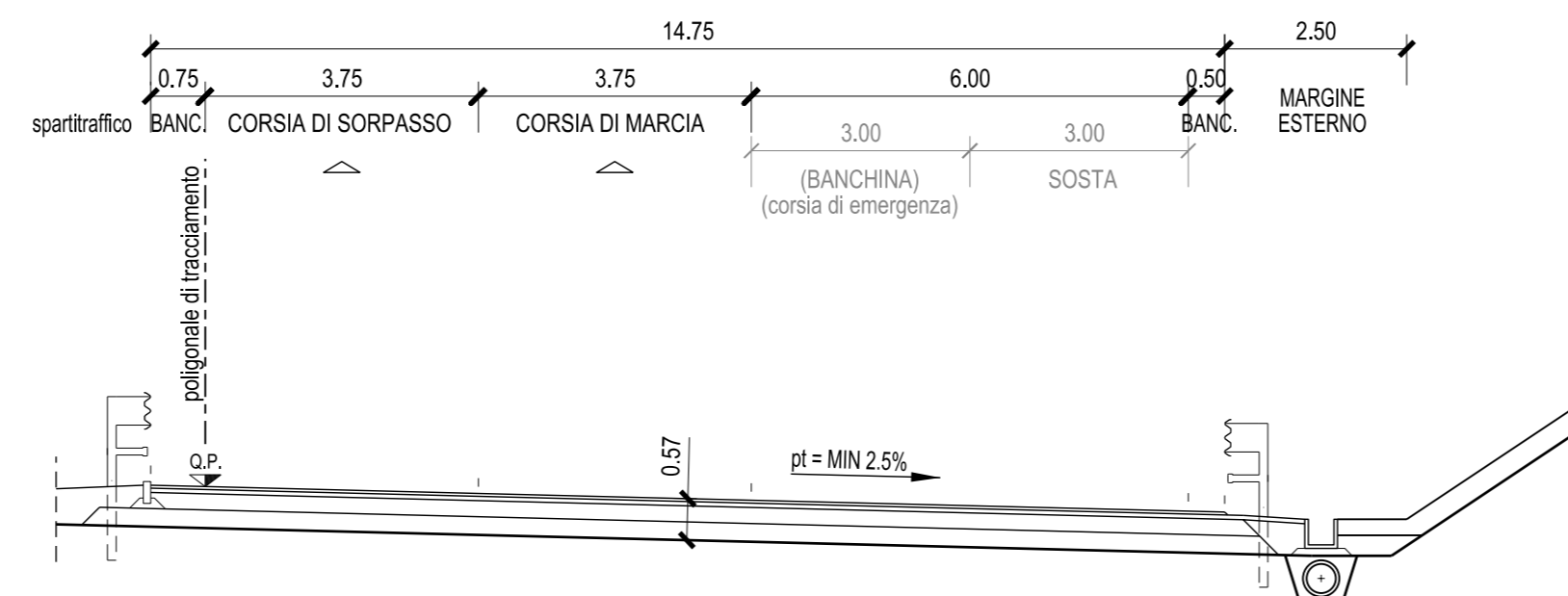
SEZIONE B-B
