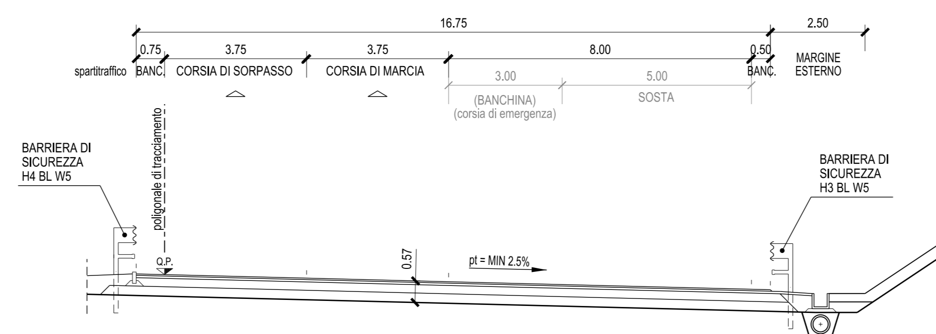
SEZIONE A-A
