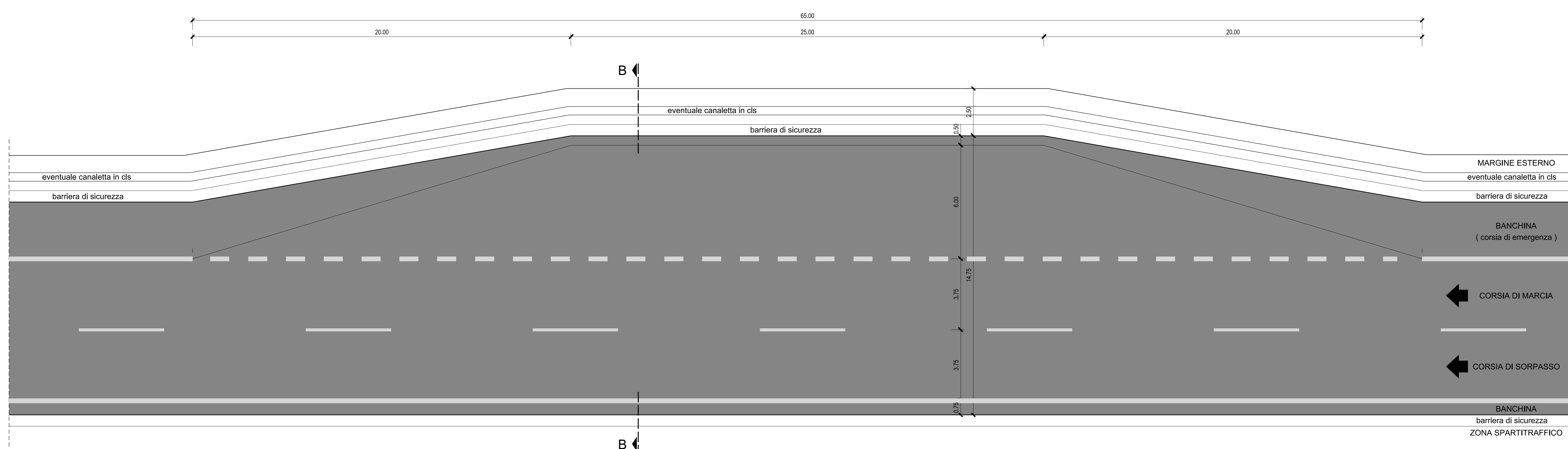
SEZIONE B-B
