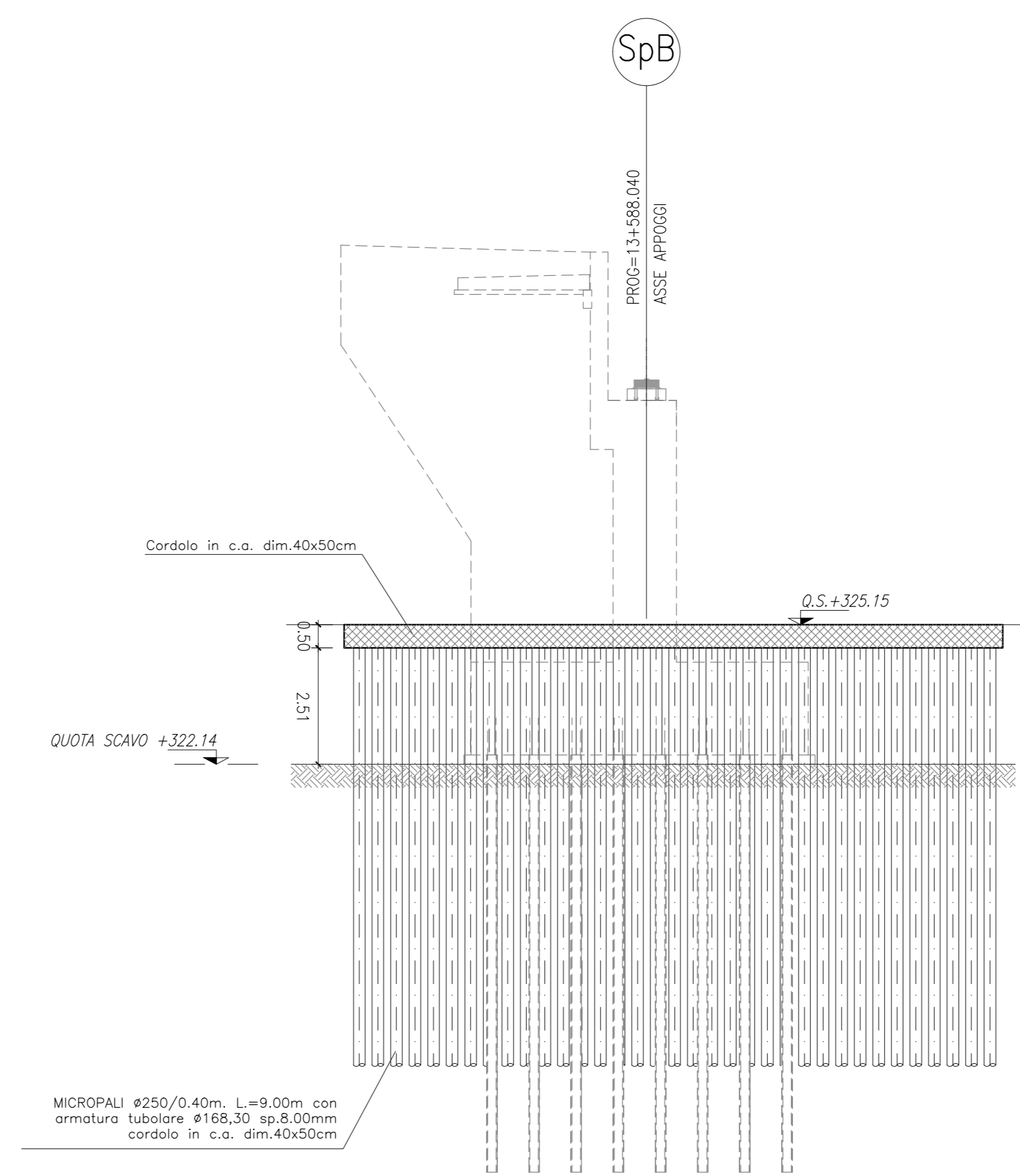
SEZIONE B-B PARATIA CARREGGIATA SUD SCALA 1:100
