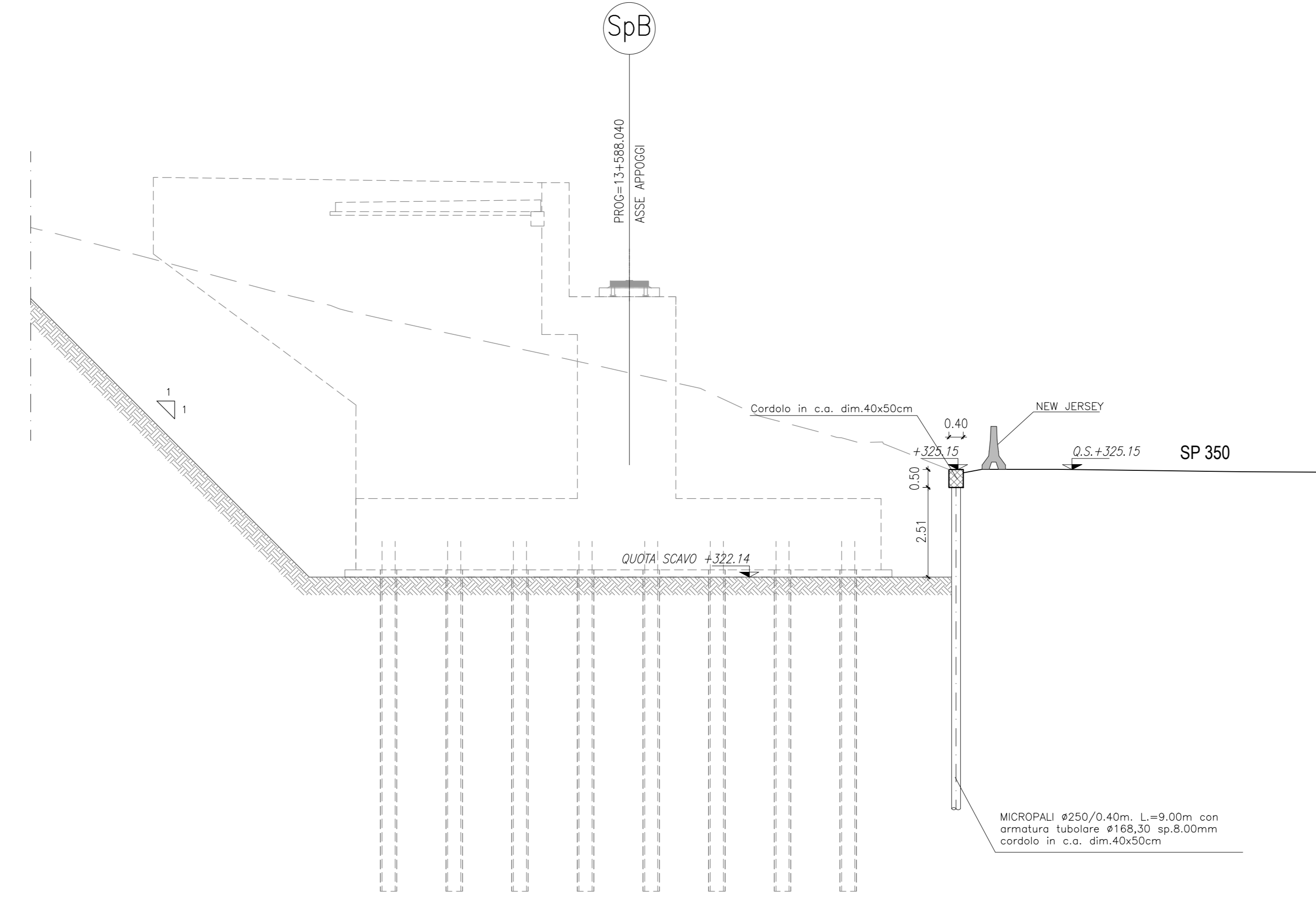
SEZIONE A-A PARATIA CARREGGIATA SUD SCALA 1:100
