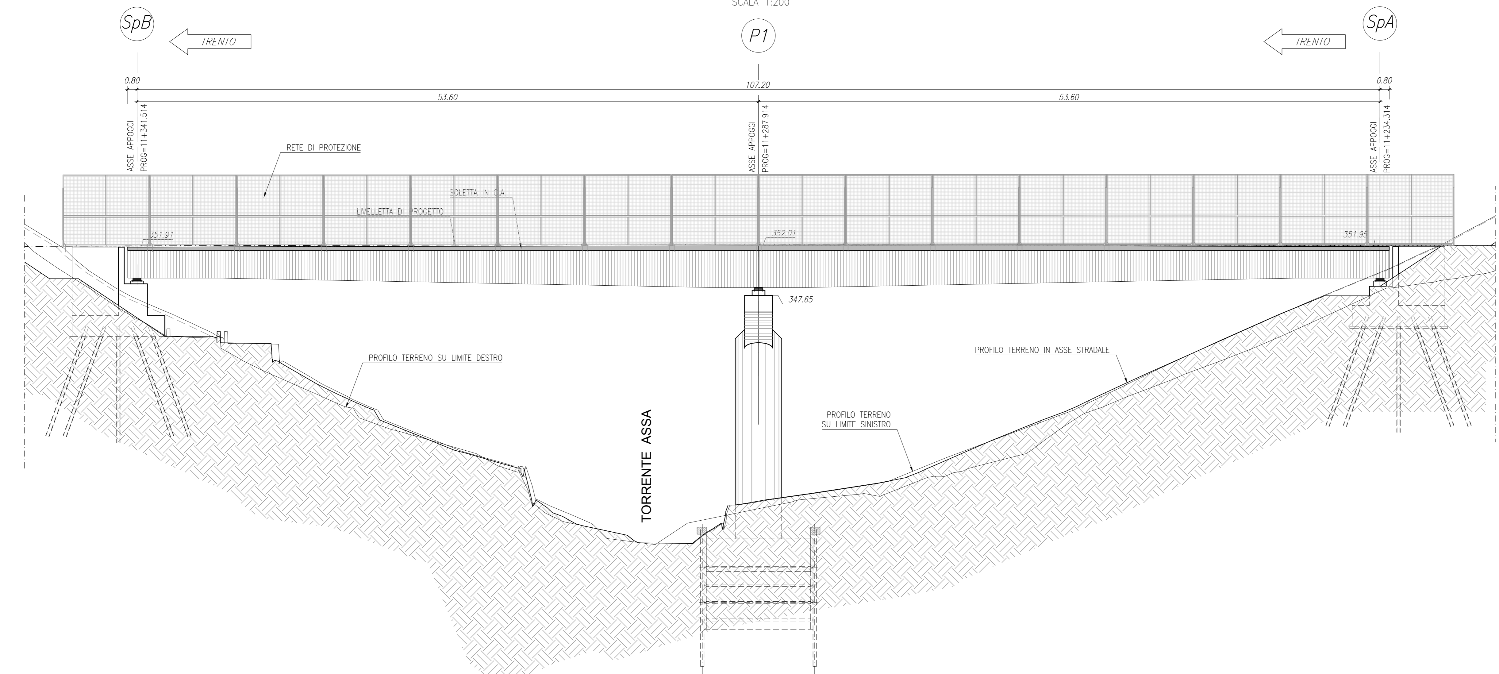
PROSPETTO LONGITUDINALE CARREGGIATA NORD SCALA 1:200
