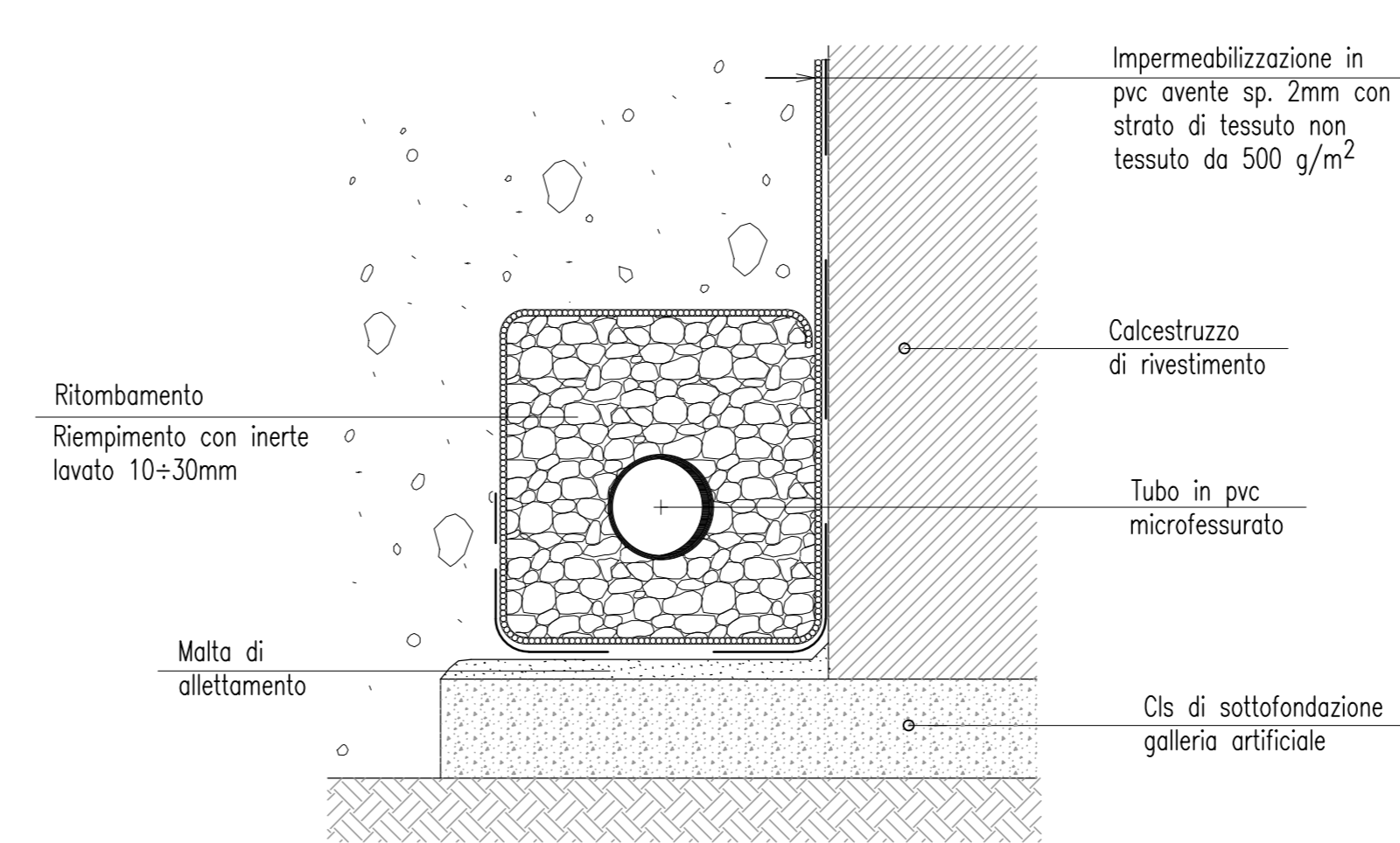
PARTICOLARE "1" IMPERMEABILIZZAZIONE E DRENAGGIO Scala 1:10
