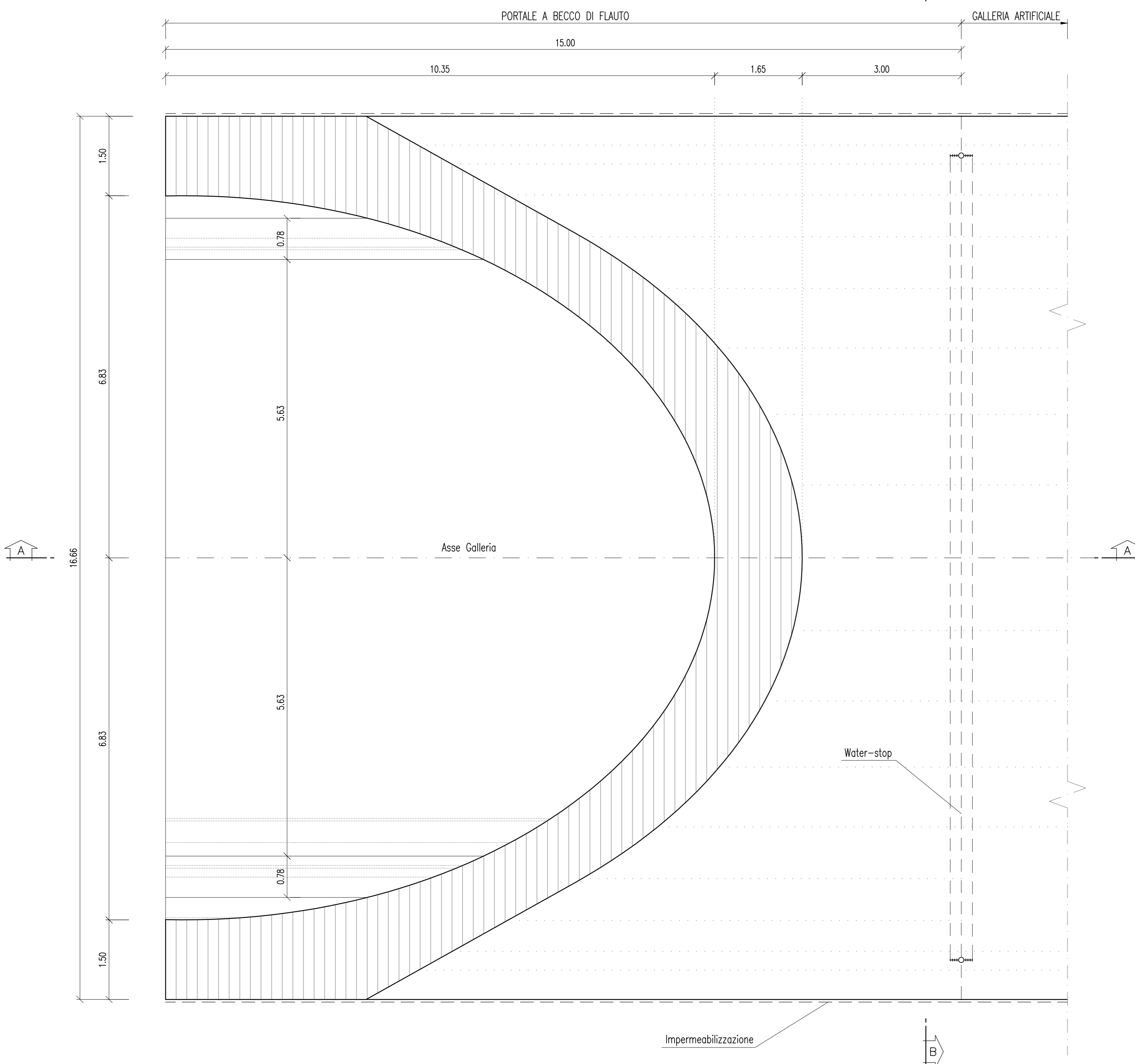
PIANTA PORTALE A BECCO DI FLAUTO Scala 1:50
