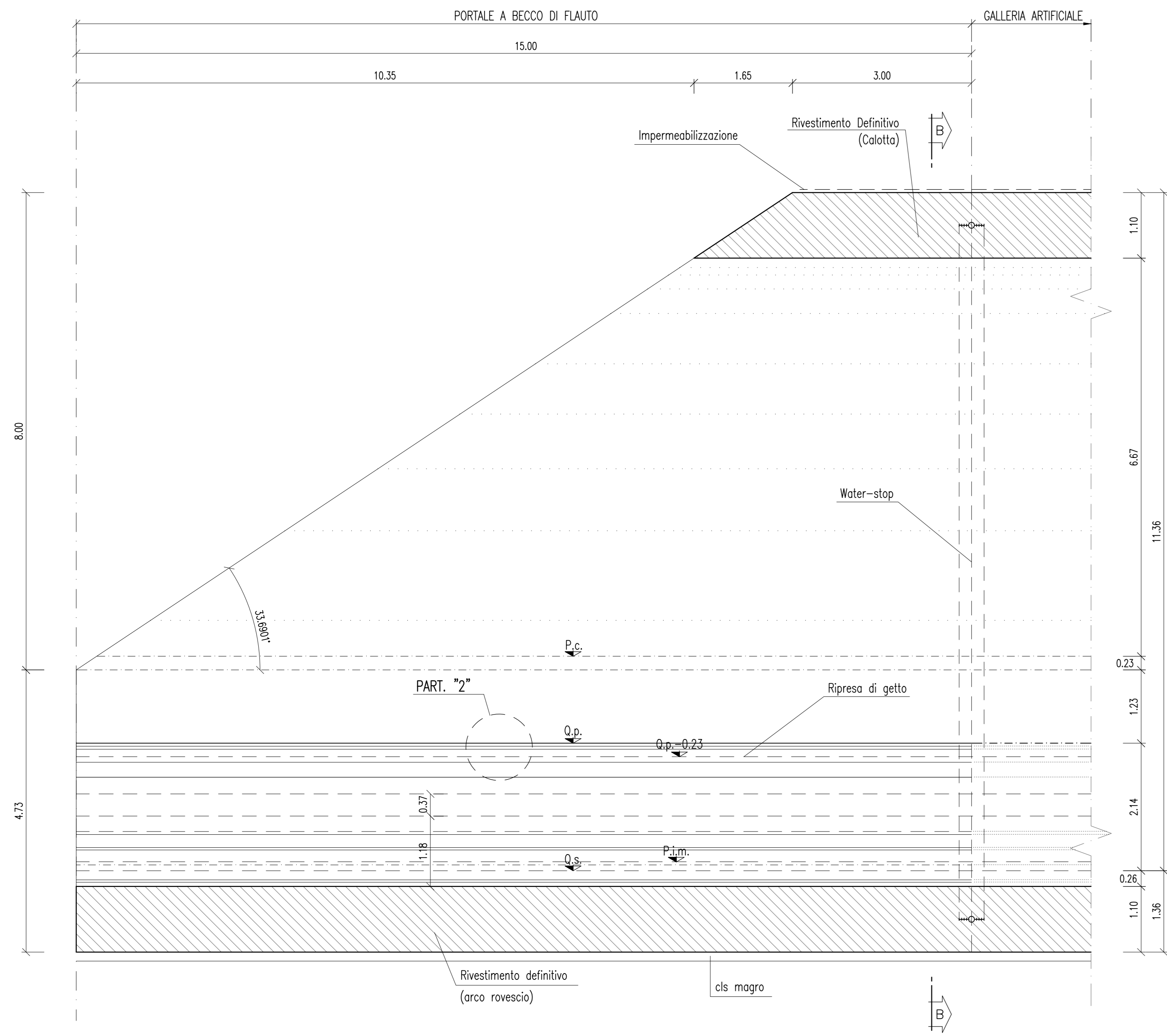
PIANTA PORTALE A BECCO DI FLAUTO Scala 1:50
