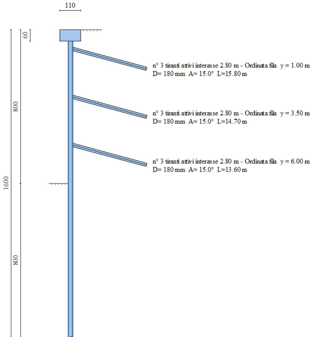
Figura 3: sezione trasversale
