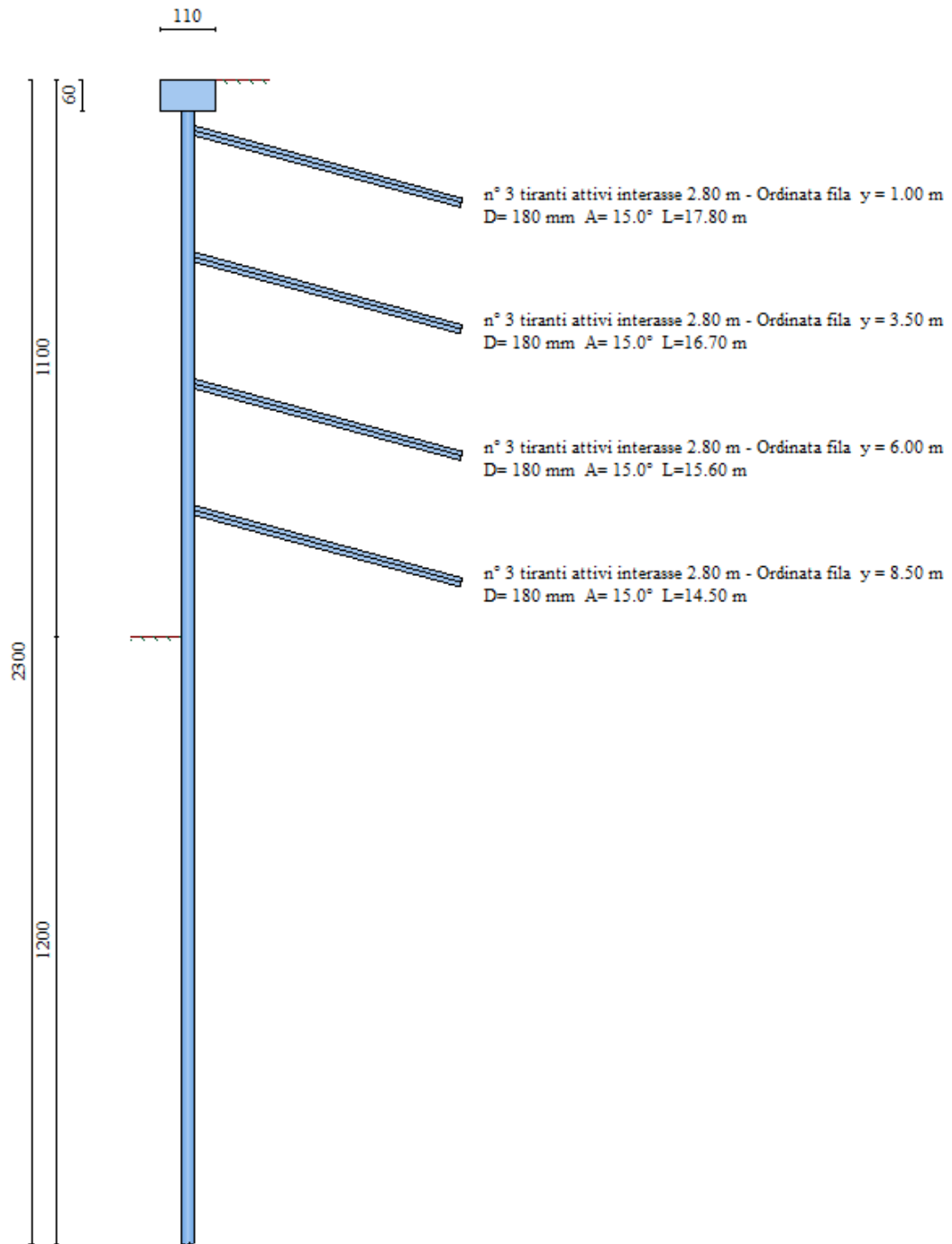
Figura 5: sezione trasversale
