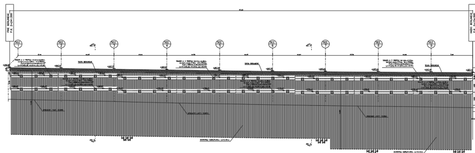
Figura 3 – Prospetto Paratia berlinese, opera 4.
