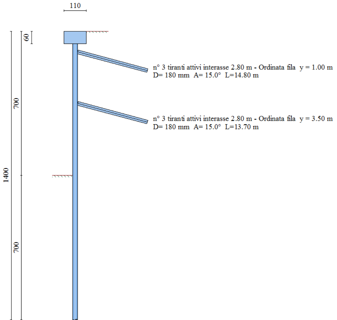
Figura 2: sezione trasversale
