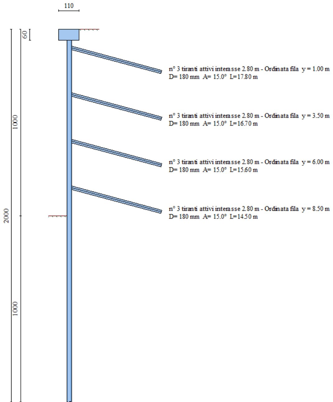
Figura 4: sezione trasversale
