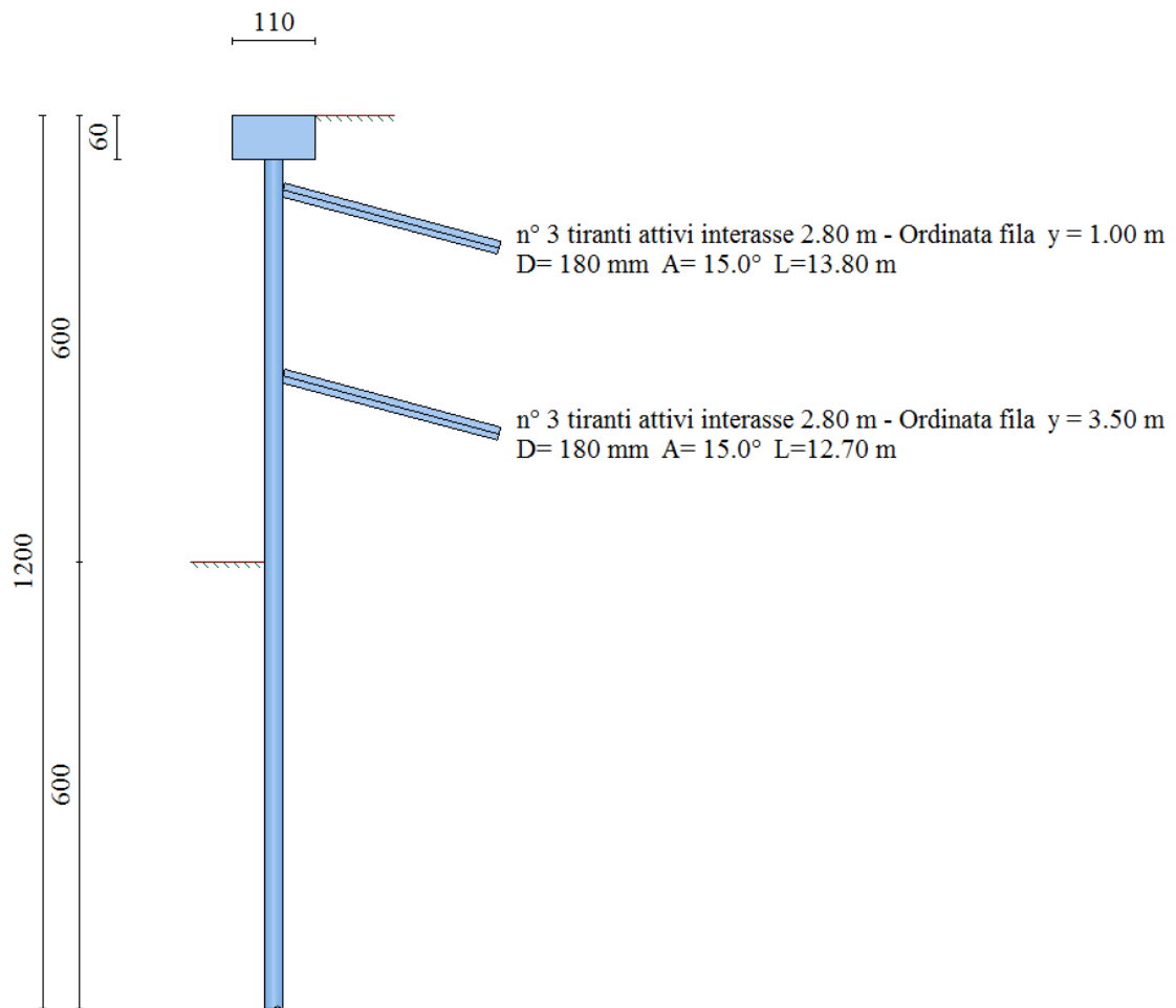
Figura 1: sezione trasversale
