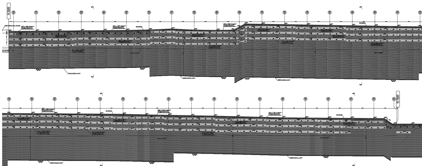
Figura 1 – Prospetto Paratia berlinese carreggiata nord, opera 2.
