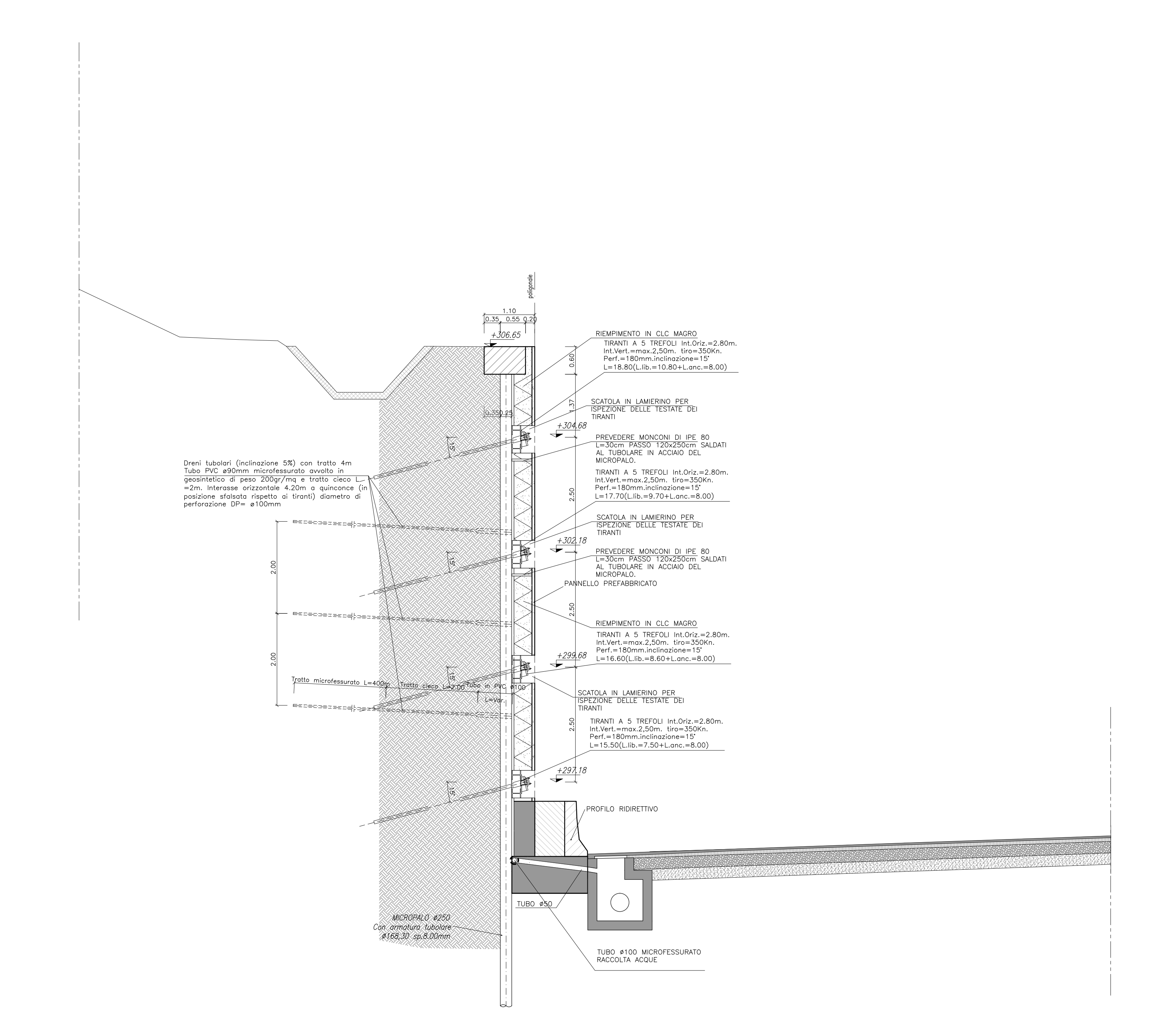
SEZIONE TRASVERSALE D-D SCALA 1:50
