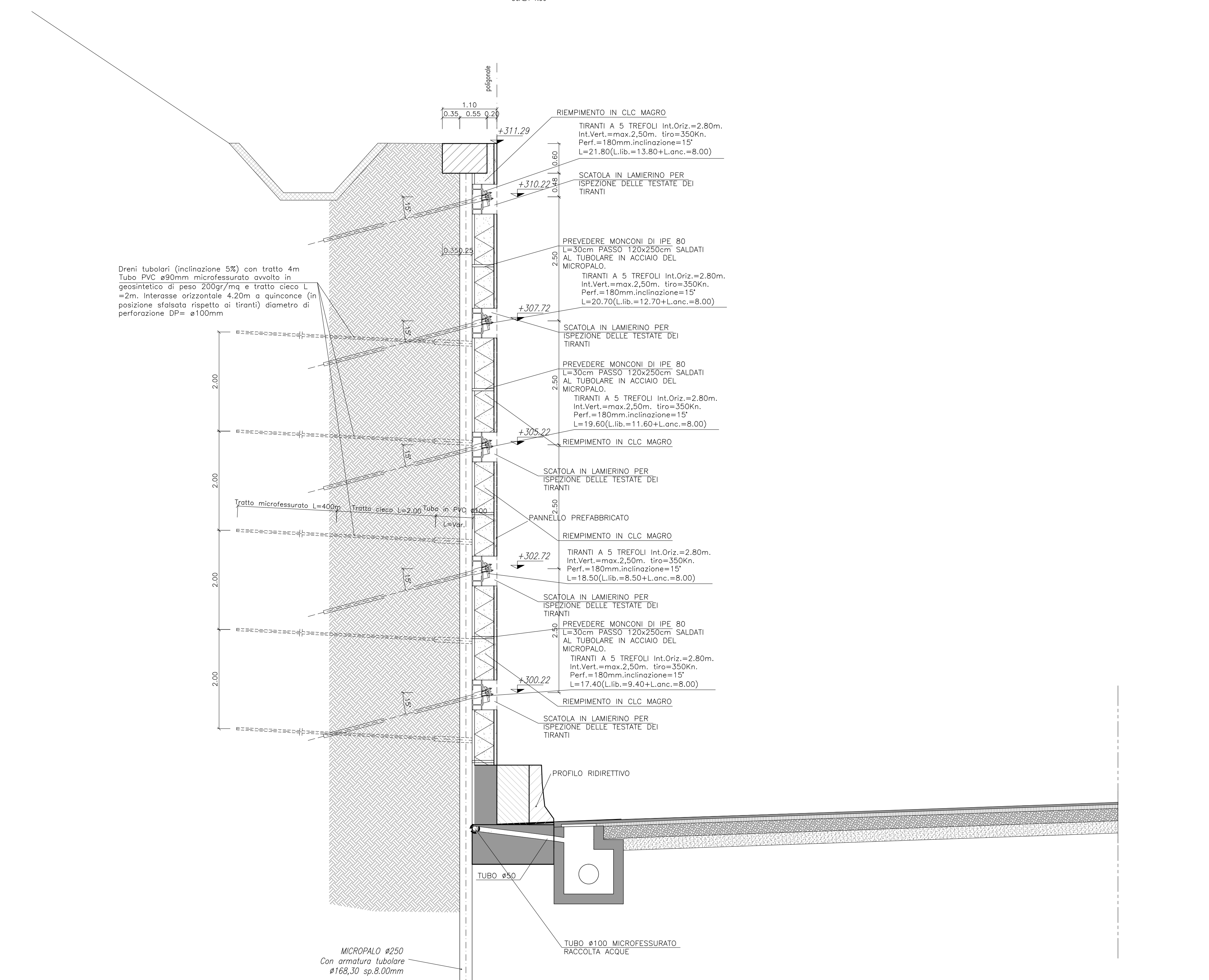
SEZIONE TRASVERSALE C-C SCALA 1:50
