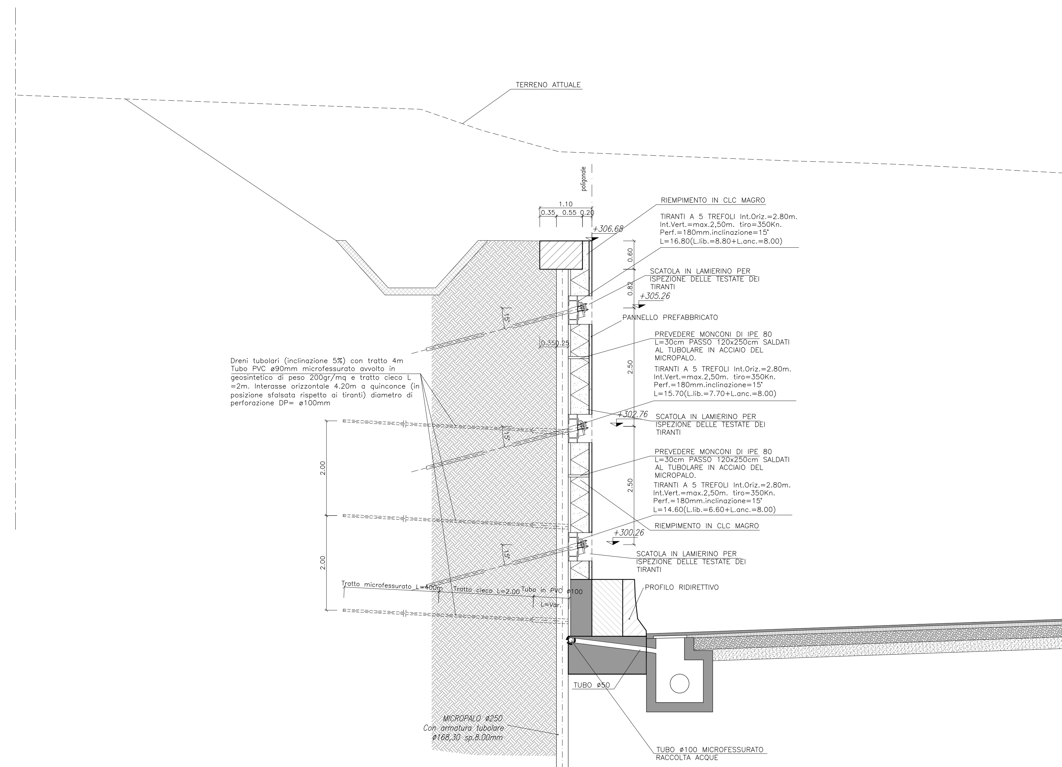
SEZIONE TRASVERSALE B-B SCALA 1:50
