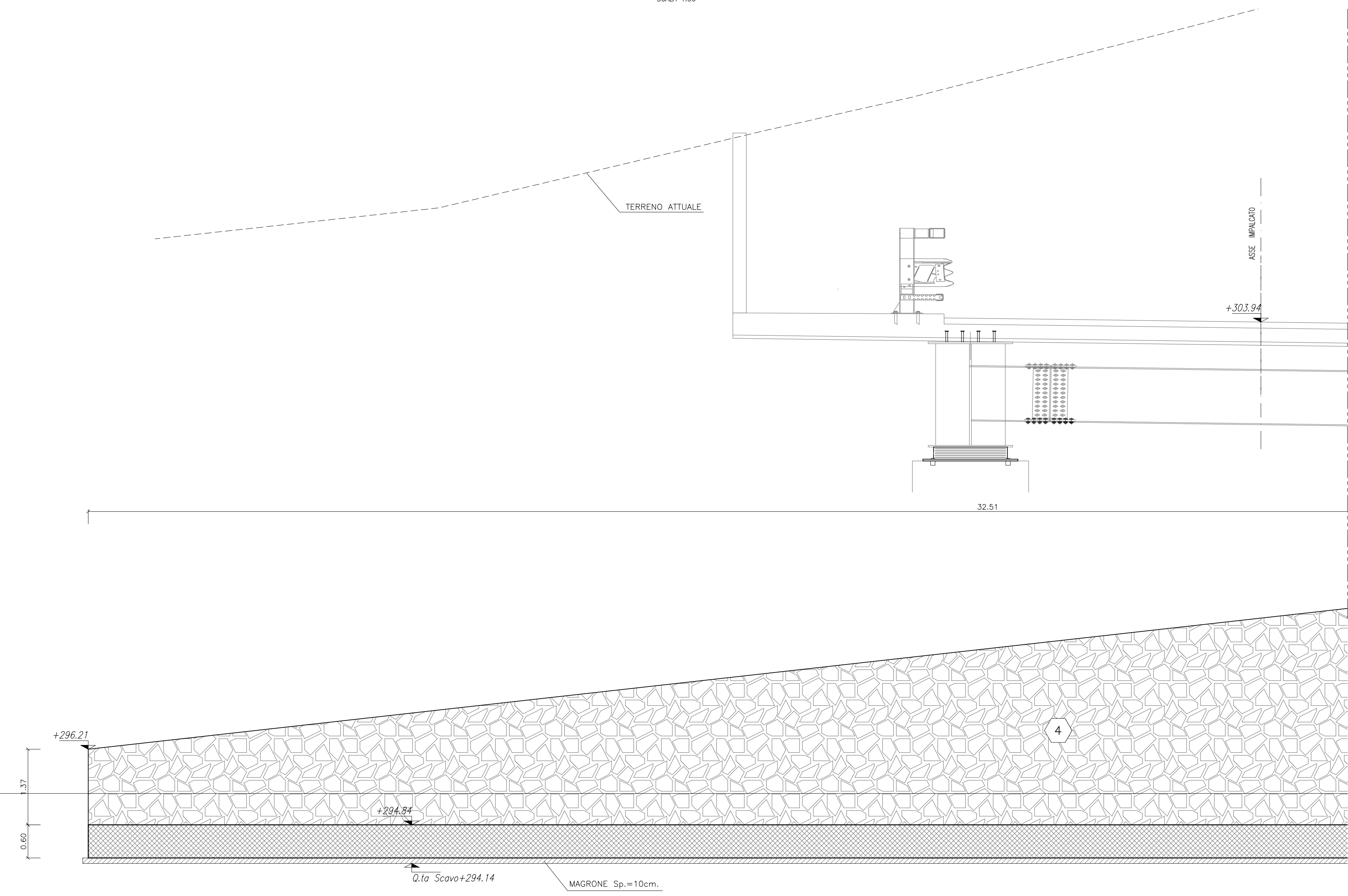
SEZIONE TRASVERSALE A-A SCALA 1:50
