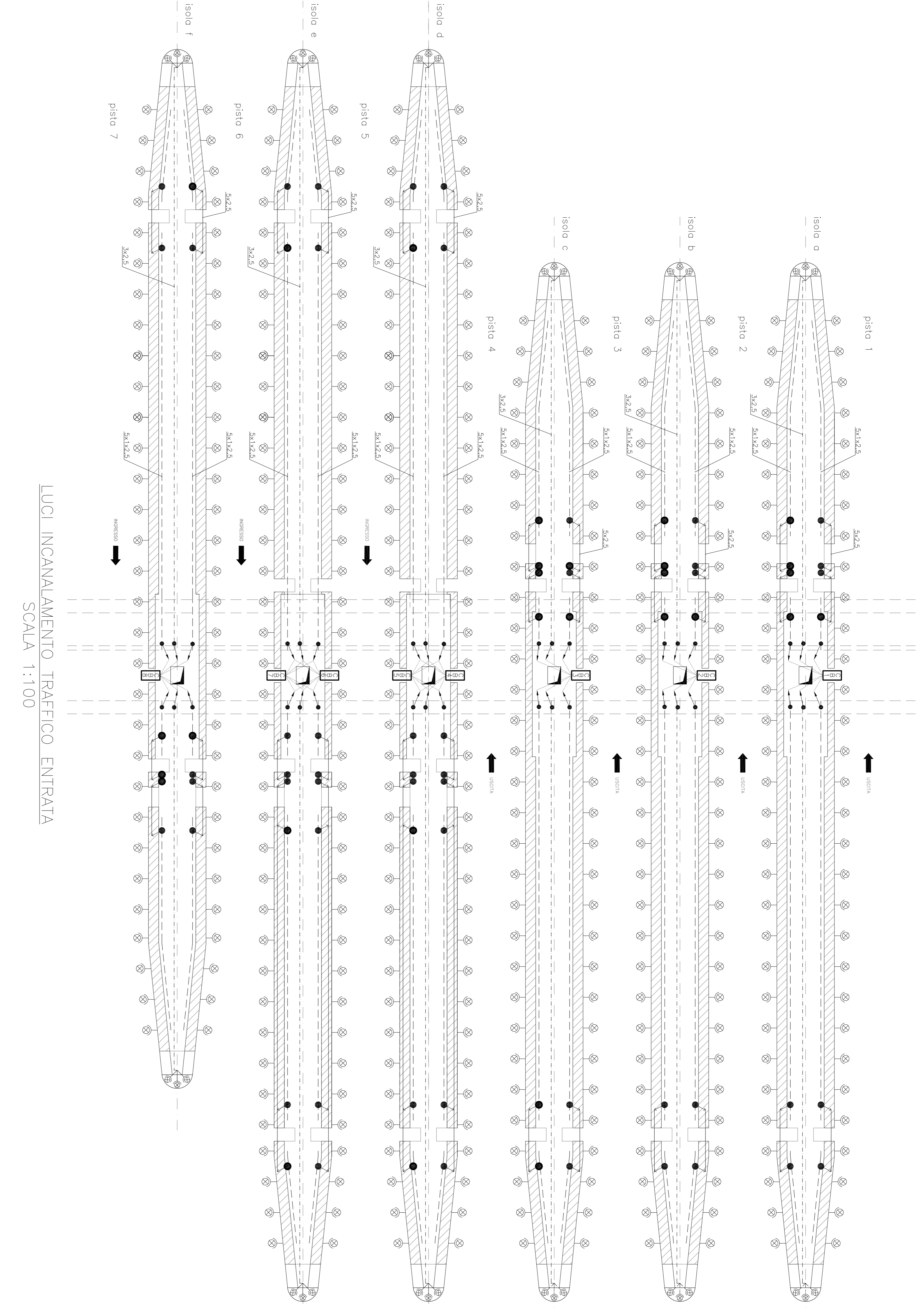
LUCI INCANALAMENTO TRAFFICO USCITA SCALA 1:100
